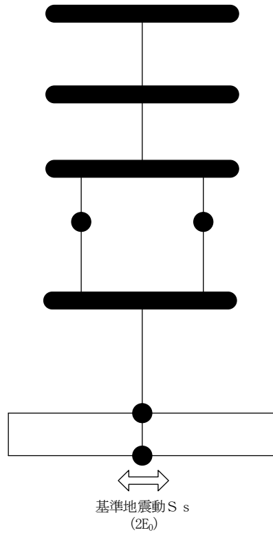
図 3-5 地震応答解析モデルに入力する地震動の概念図
