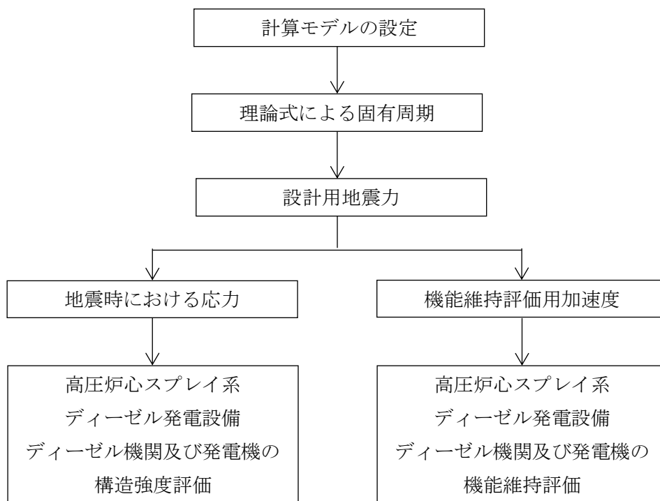
図 2-1 高圧炉心スプレイ系ディーゼル発電設備ディーゼル機関及び発電機の耐震評価フロー
