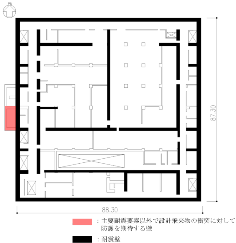
第 5-1 図(1/3) 燃料加工建屋 耐震壁の位置(T. M. S. L. 50. 30m)
