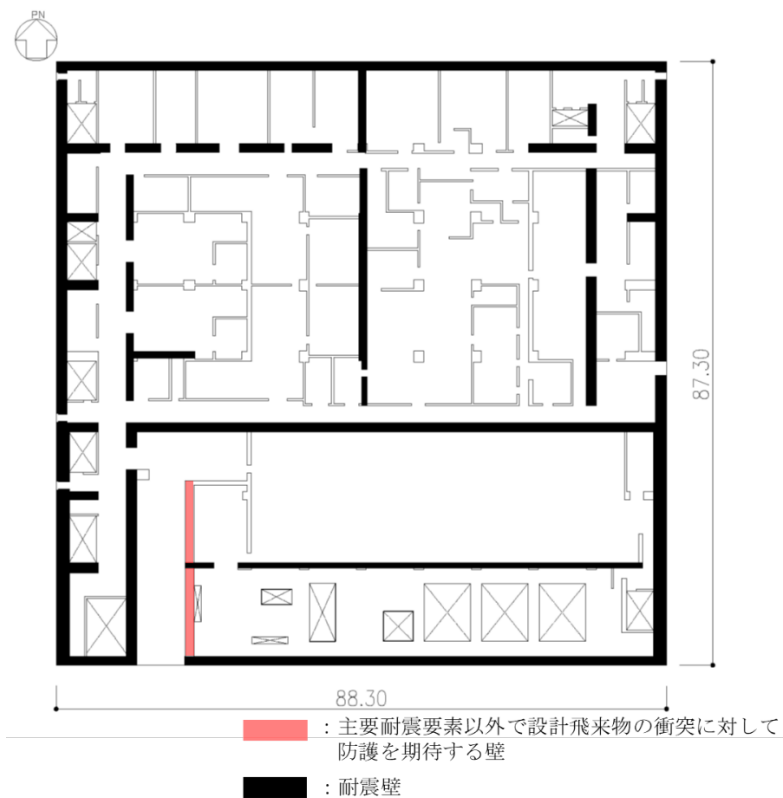
第 5-1 図(2/3) 燃料加工建屋 耐震壁の位置(T. M. S. L. 56. 80m)
