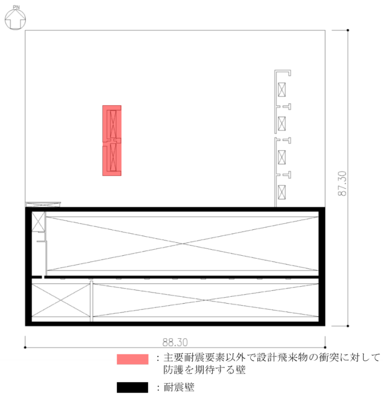
第 5-1 図 (3/3) 燃料加工建屋 耐震壁の位置 (T. M. S. L. 70. 20m)
