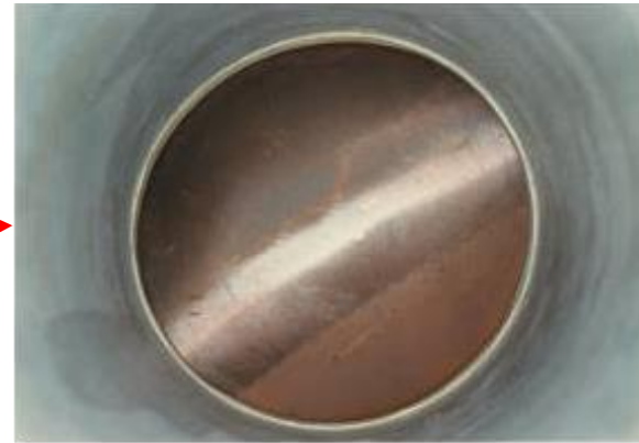
コールドレグ (例：Aループ (A-12))
