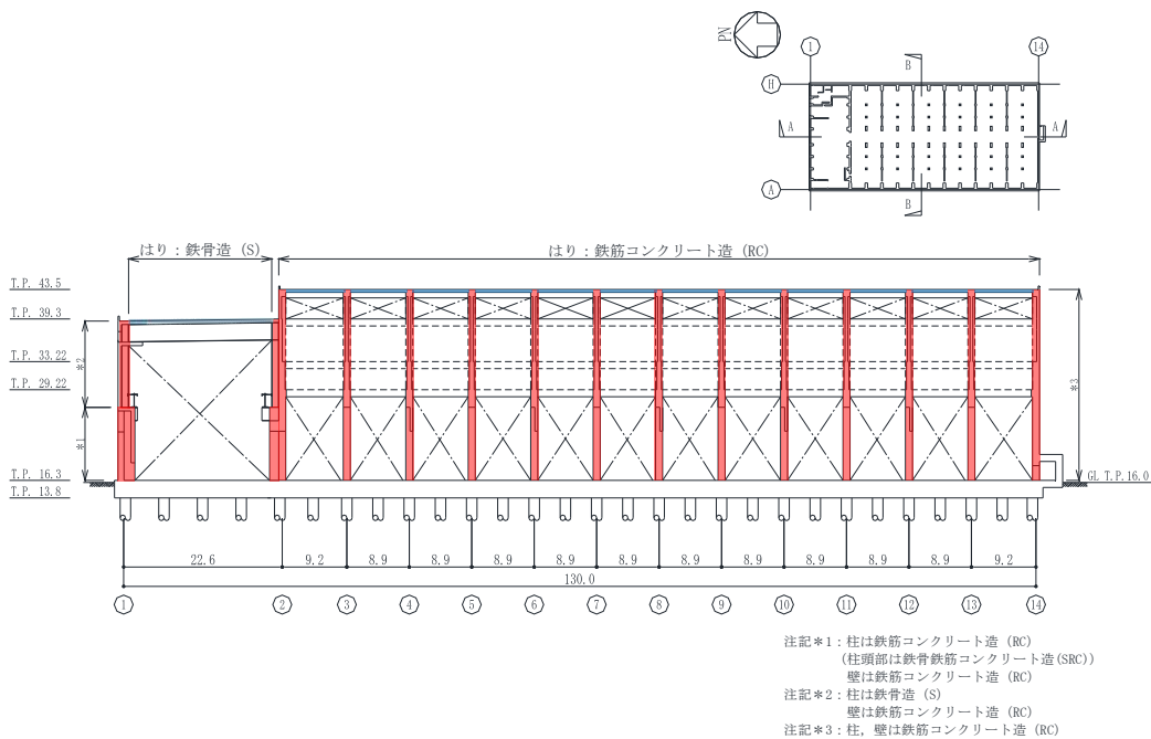
図2-3 A-A断面図(NS方向)(単位:m)
