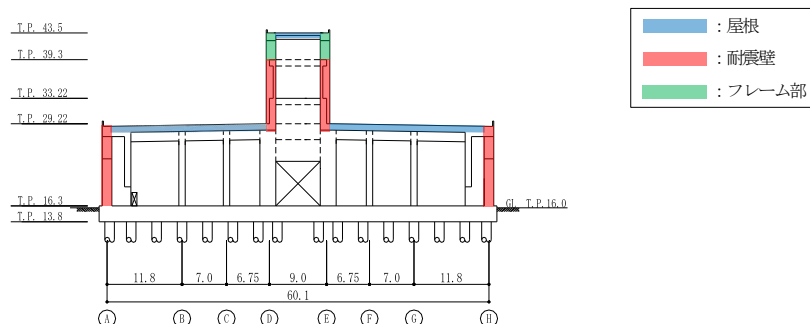
図2-4 B-B断面図(EW方向)(単位:m)
