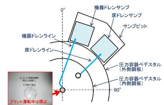
図 1-2 ドライウエルサンブの配置
