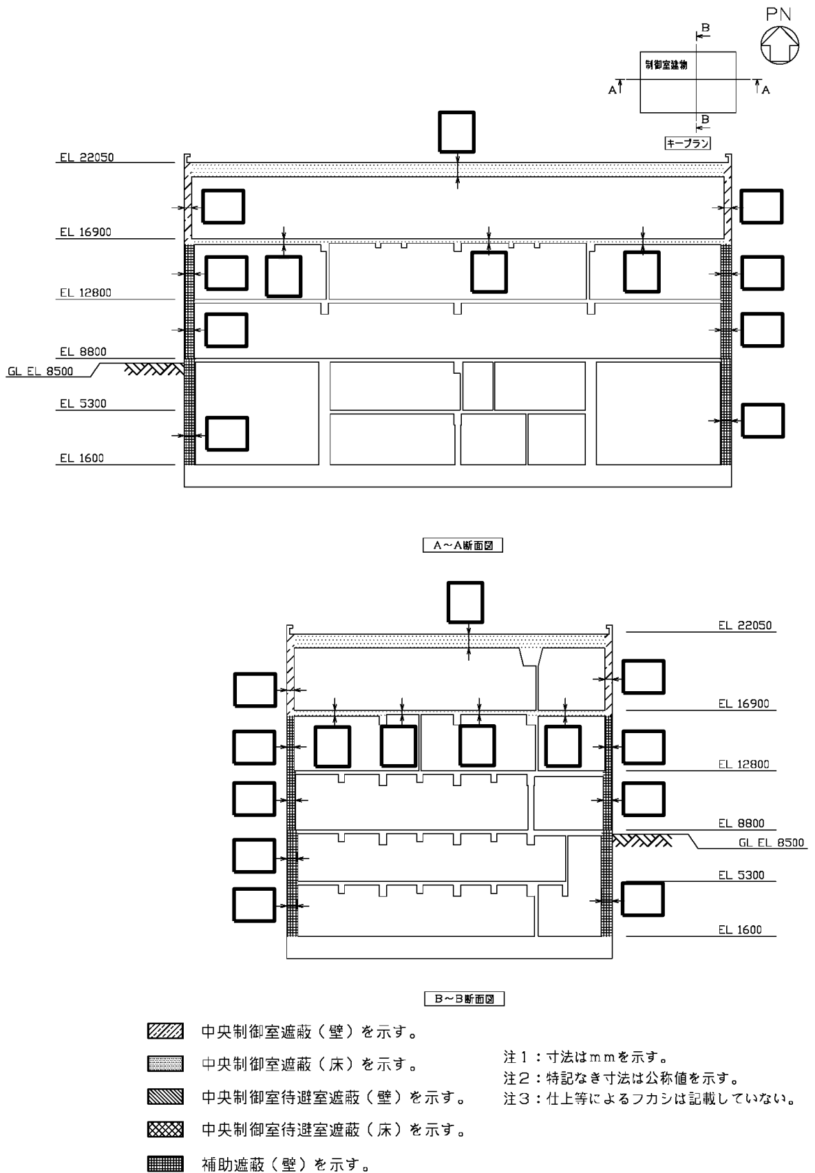
図 4-1 遮蔽構造図 (4/4)
