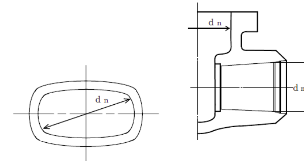
注：本図は告示第 5 0 1 号第 82 条解説の図 82. 3 又は設計・建設規格 VVB-3210 解説図 VVB-3210-3 と同じ。
