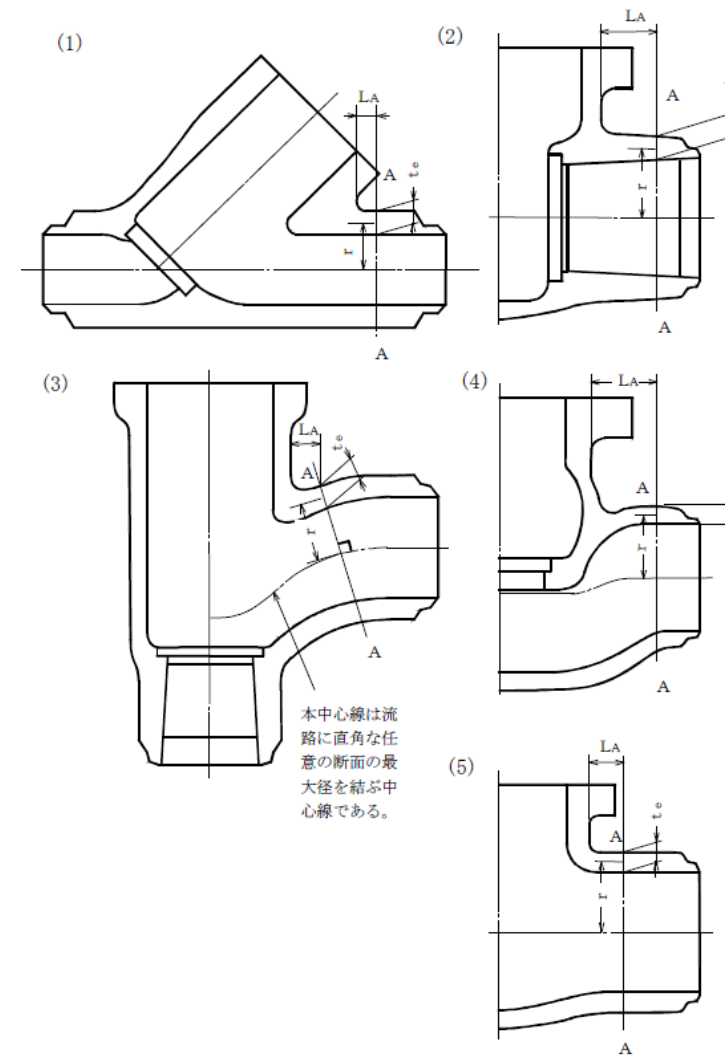
注：本図は告示第501号第81条第1項第1号口の図1又は設計・建設規格 VVB-3330の図 VVB-3330-1と同じ。 図 3-2 t e 及びrを明示した図
