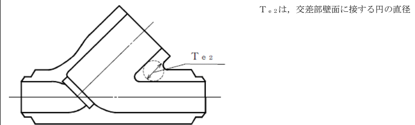
注：本図は図 3-3 の (3) の内容を図 3-2(1) の構造に適用したもの
