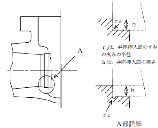
注：本図は設計・建設規格 VVB-3411 の図 VVB-3411-2 と同じ。
