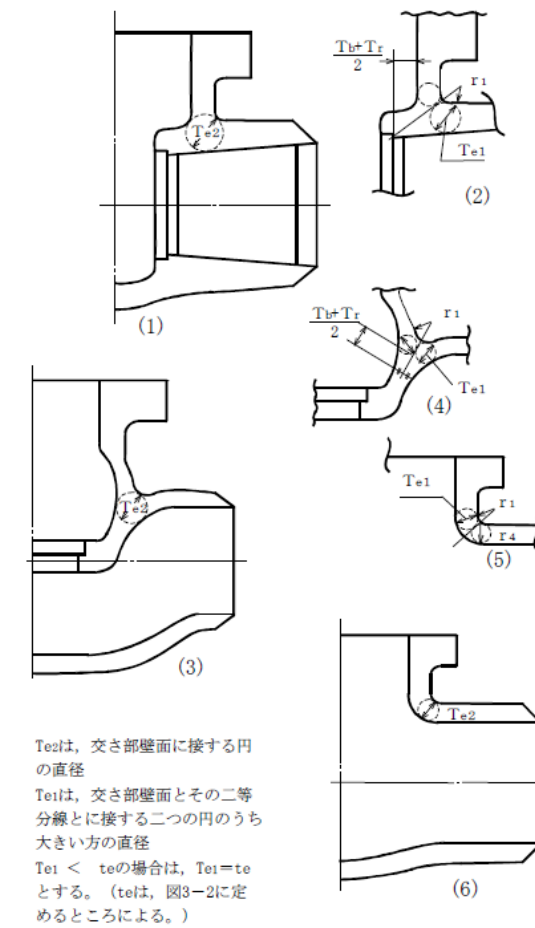
注 : 本図は設計・建設規格 VVB-3340 の図 VVB-3340-1 と同じ。 図 3-3 T_{e1} 及び T_{e2} を明示した図
