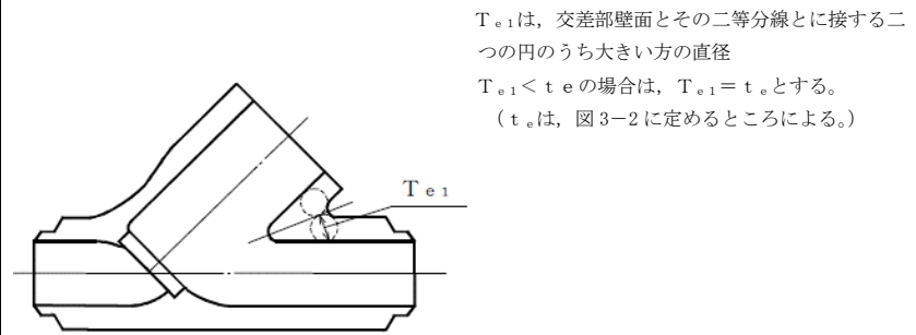
注：本図は図 3-3 の (4) の内容を図 3-2(1) の構造に適用したもの
