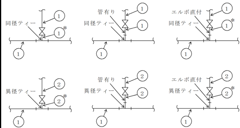
管番号及び管継手マーク記載原則の実例 (その2)
