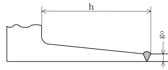
図 2-10 一体形フランジ
