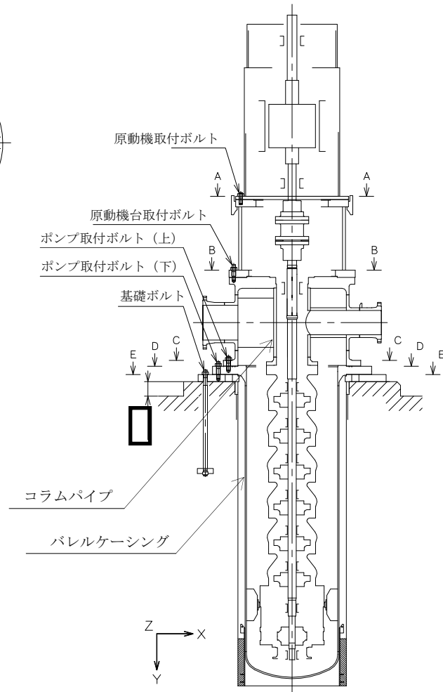
ポンプ取付ボルト (上)
