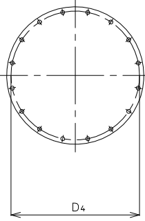
B~B矢視図
