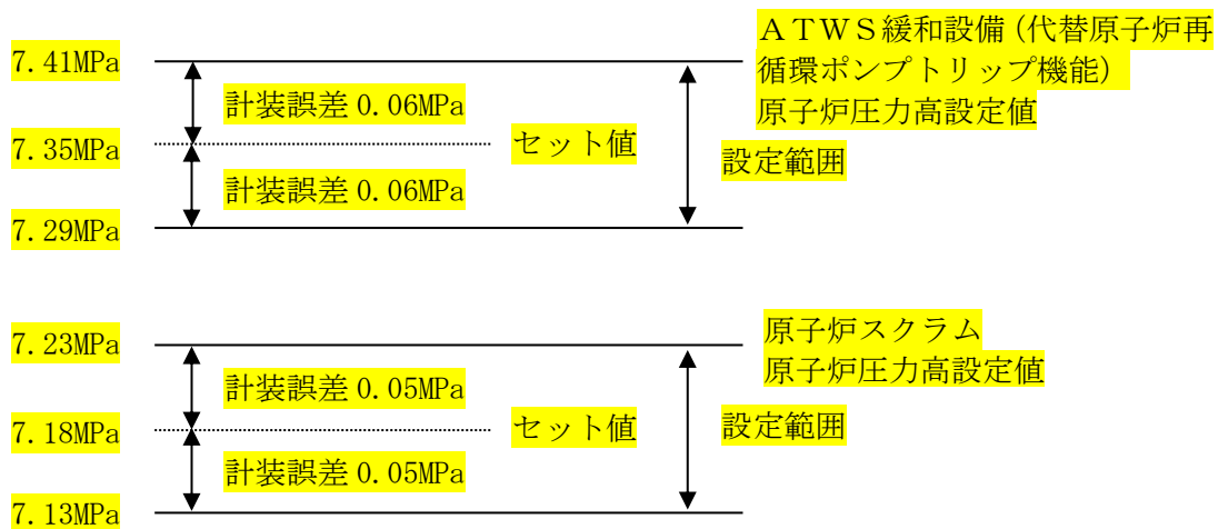
図 4-3 原子炉圧力高設定値の概要図
