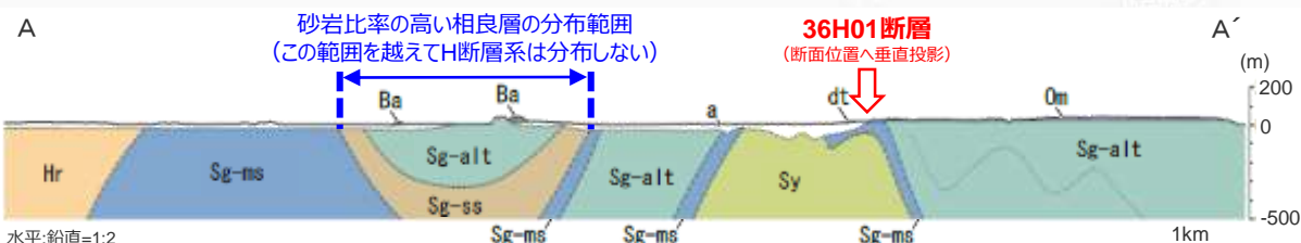
図 36H01断層の位置
