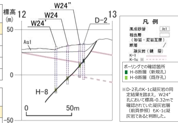
追加調査結果を踏まえたH-8断層断面図
