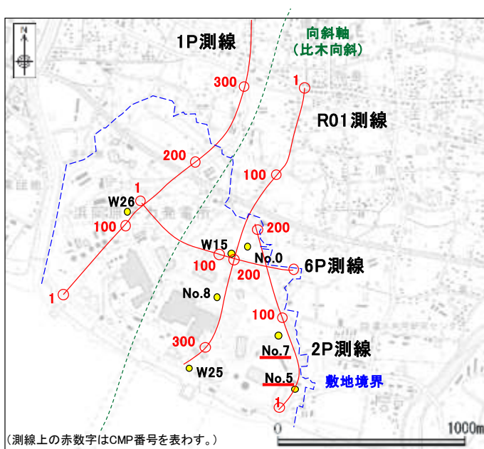
ボーリング孔位置図
