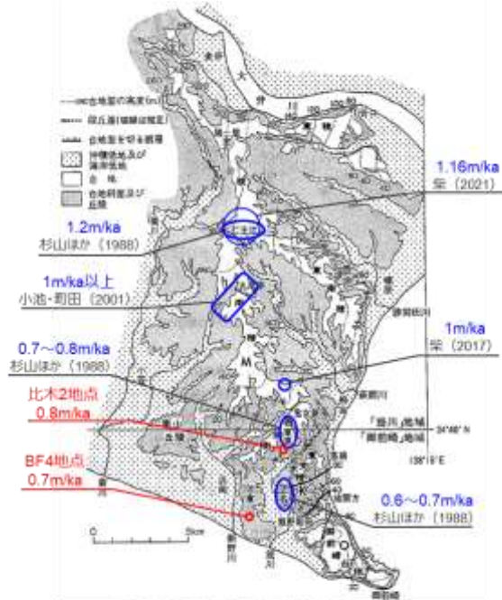
第3図 数ノ原古地周辺の地形と古地層の隆起速度分布 杉山ほか(2007)の第1図を一部修正 M: 数ノ原段丘, K: 美濃段丘, O: 濃尾断崖 各知見における隆起速度と当社調査による隆起速度（補足説明資料p.39再掲） 杉山ほか（1988）に加筆
