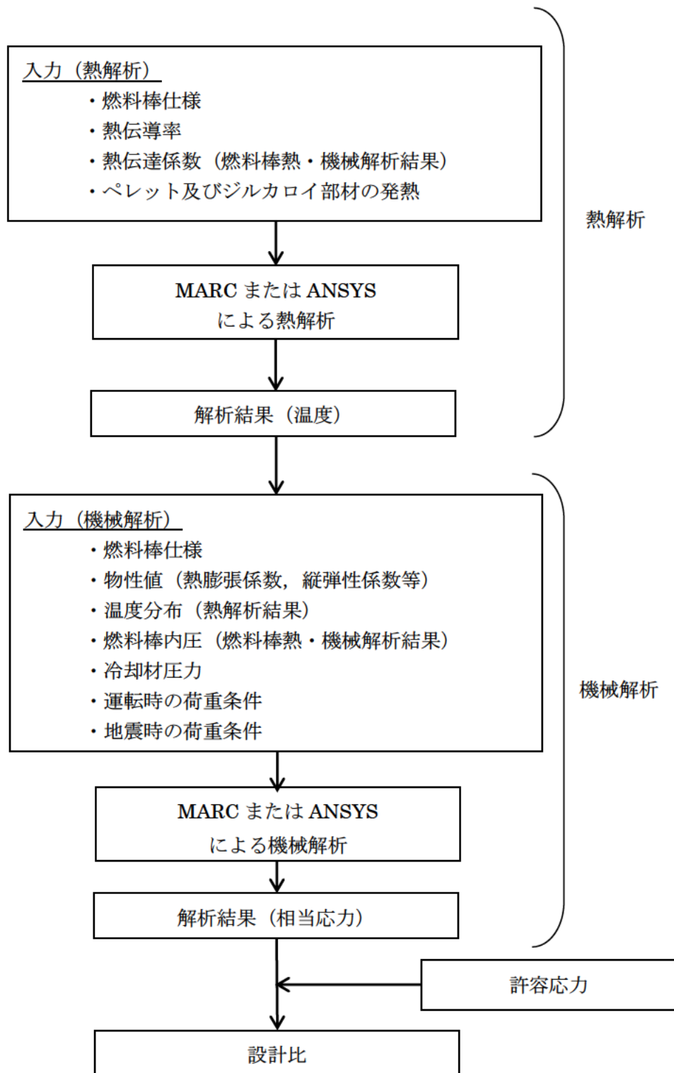
図 3-1 下部端栓溶接部の応力評価のフロー
