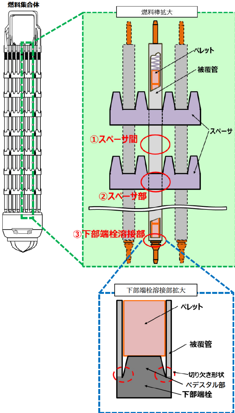
図 1-1 下部端栓溶接部の拡大図
