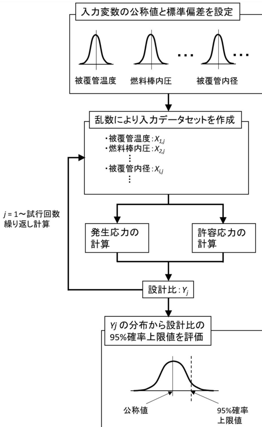
図1 モンテカルロ法による統計処理の概要フロー
