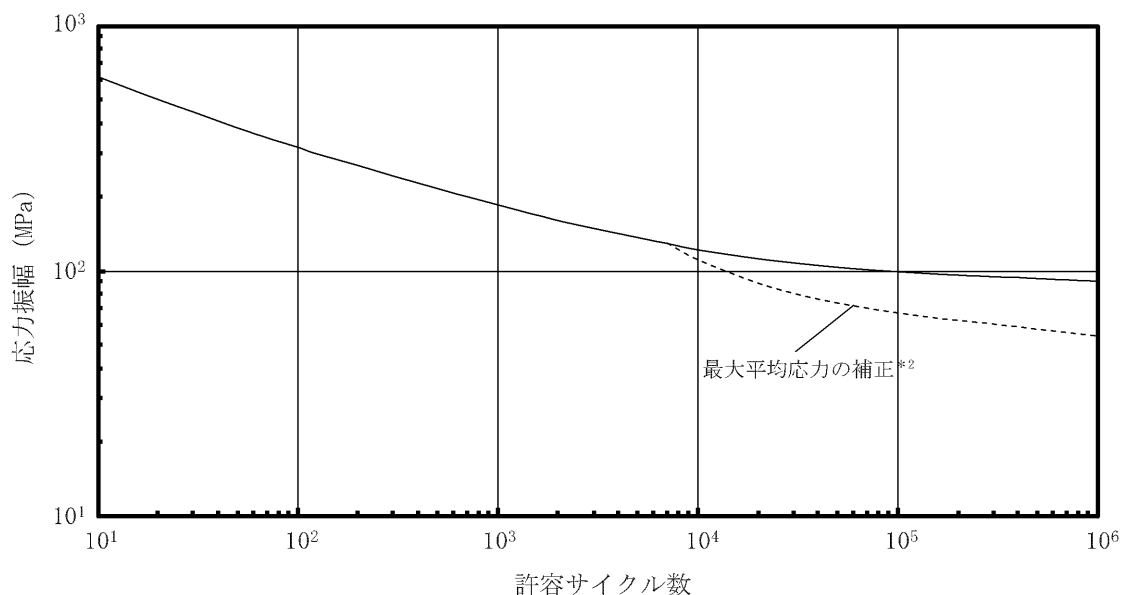
図 1 ジルカロイ設計疲労曲線
