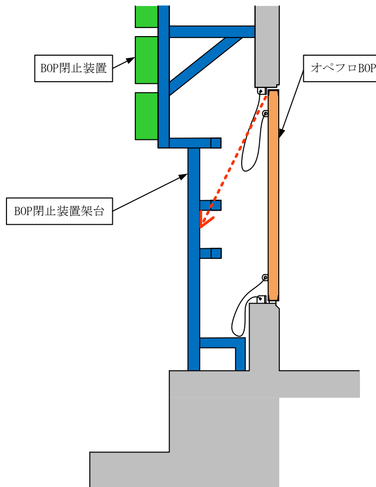
図 2-1 BOP 閉止装置架台図（断面図）
