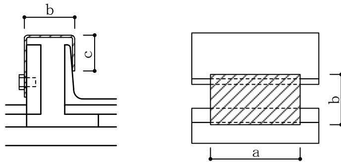
図 3-2 試験体寸法測定箇所
