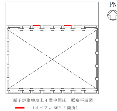
図7-1 オペフロBOP の設置位置
