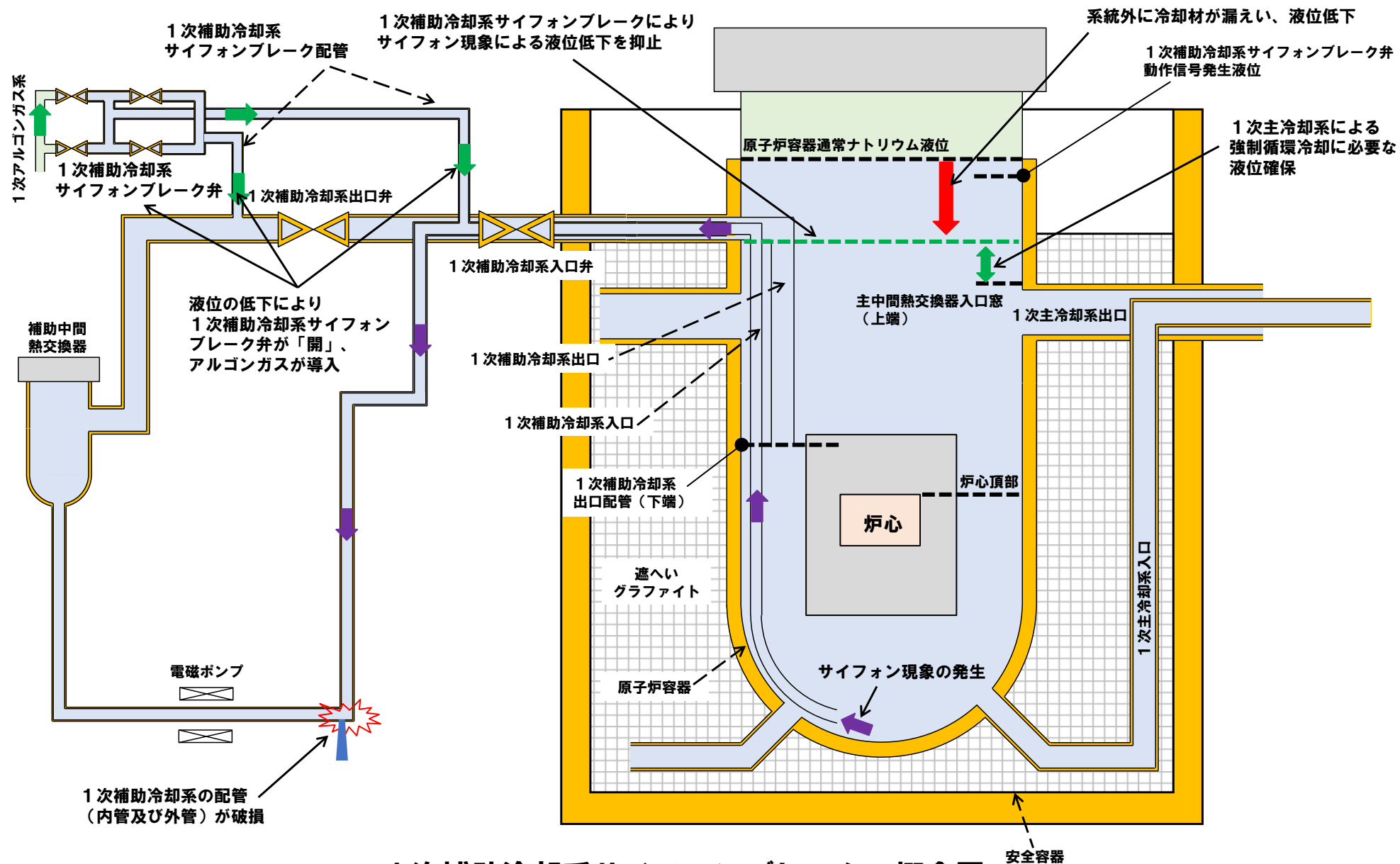
1次補助冷却系サイフォンブレークの概念図
