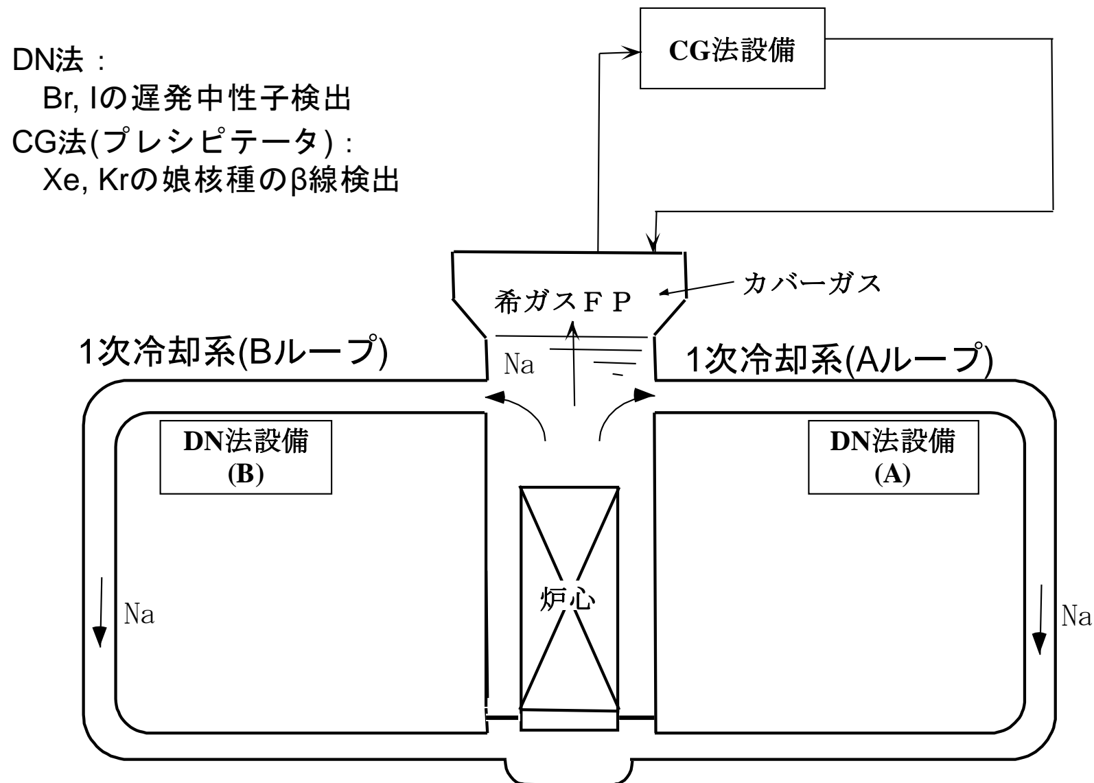
燃料破損検出系の概念図
