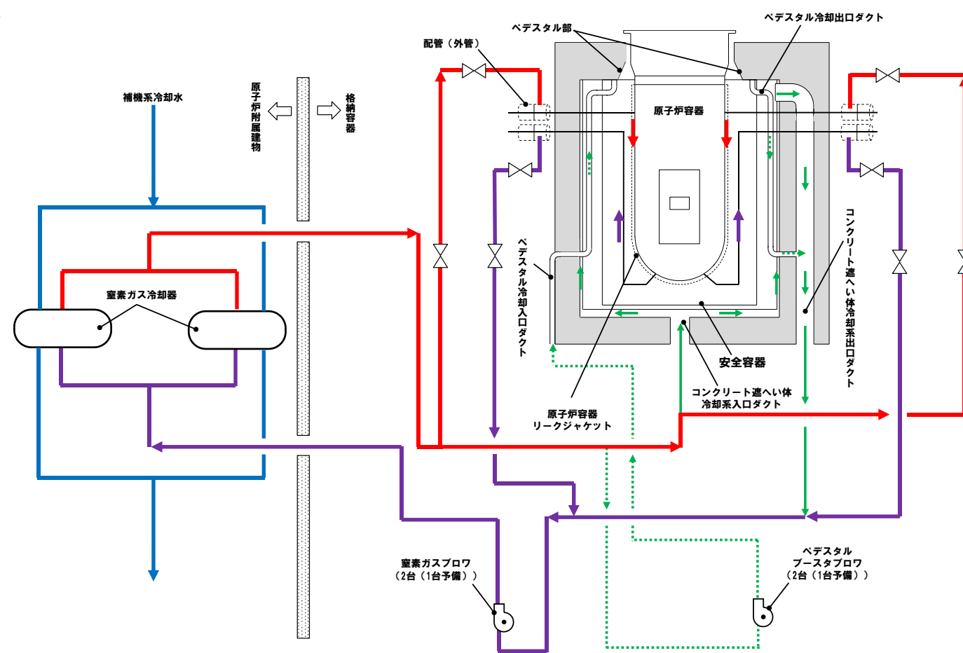
第2図 原子炉容器外面冷却
