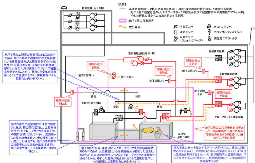
図 4-1 地震を要因とした重大事故等に機能維持することを期待する設備等の概要図
