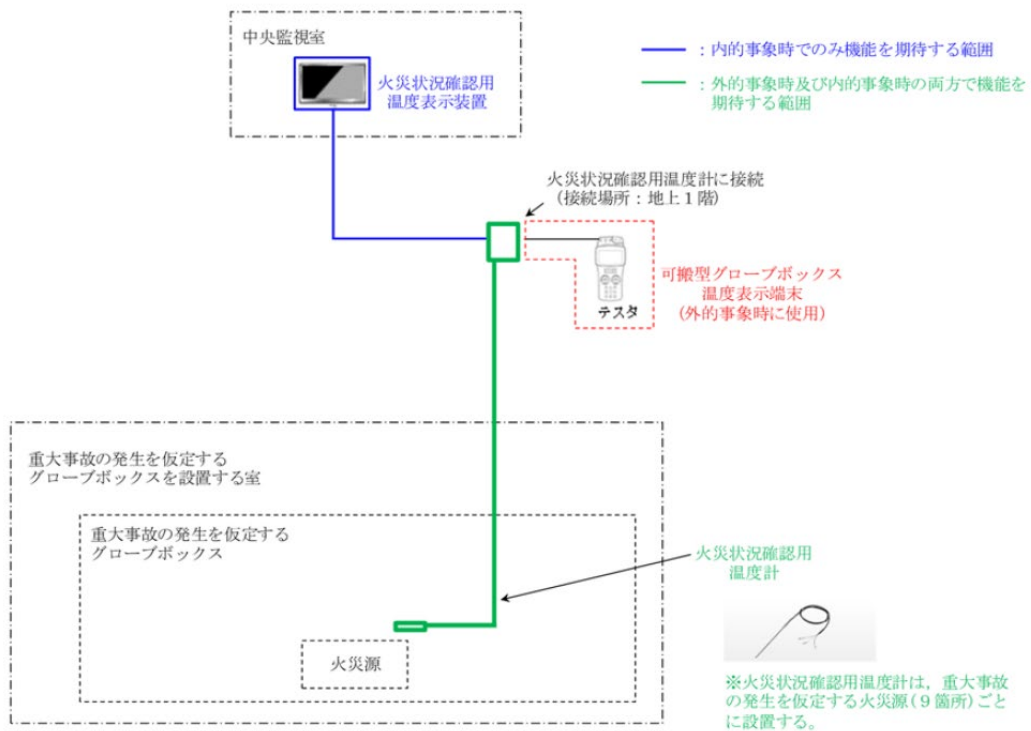
図3-2 火災状況の確認のための重大事故等対処設備の概要図
