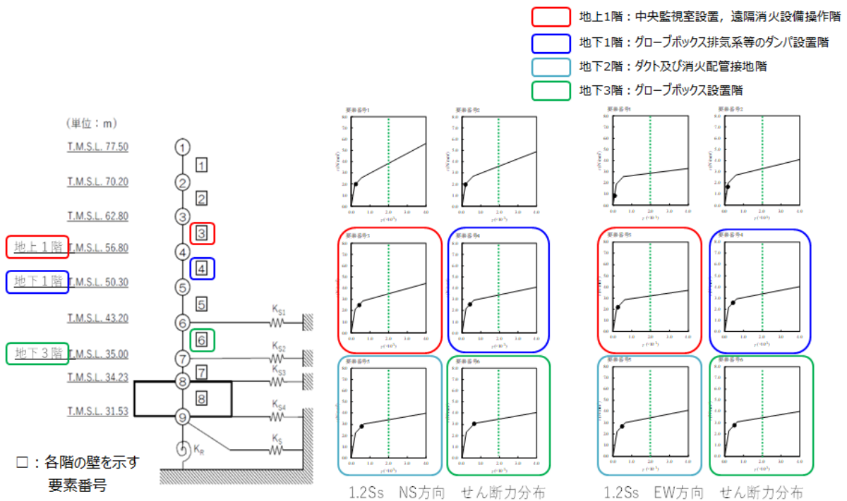
図7-1 燃料加工建屋 各階における 1.2 \times S_s による最大せん断ひずみ度
