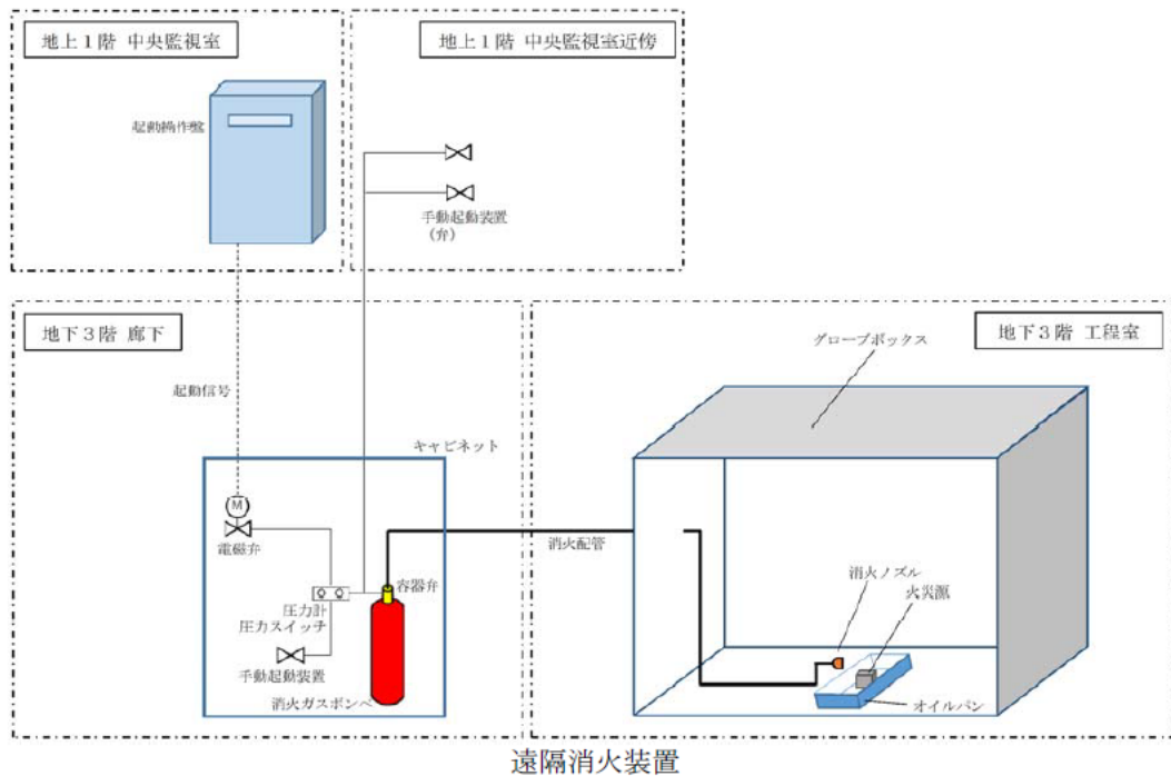
図3-3 火災の消火のための重大事故等対処設備の概要図
