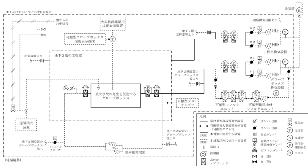
外部放出抑制設備の系統概要図
