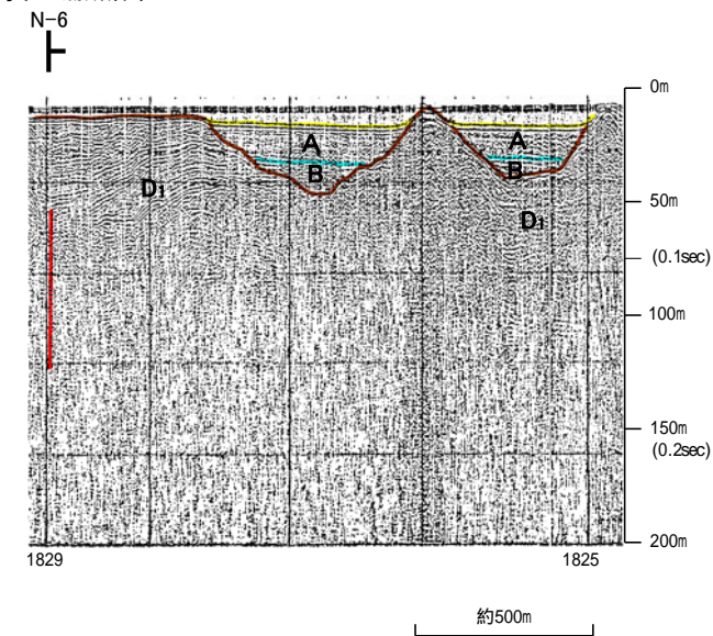
能登島半の浦断層帯
