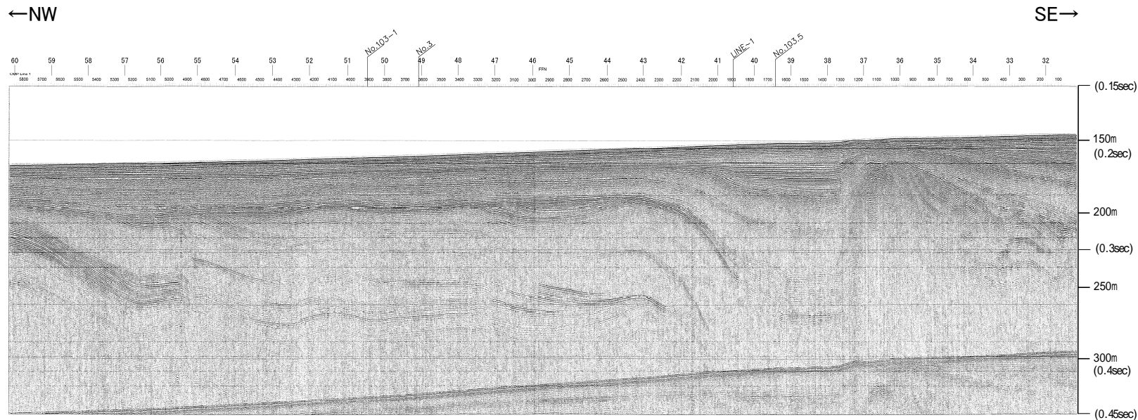
前ノ瀬東方断層帯
