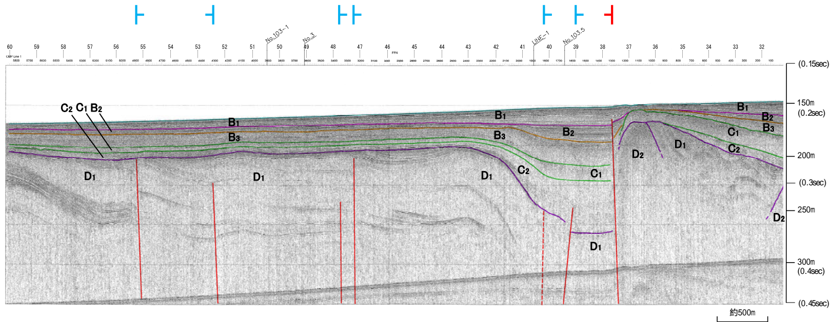
前ノ瀬東方断層帯
