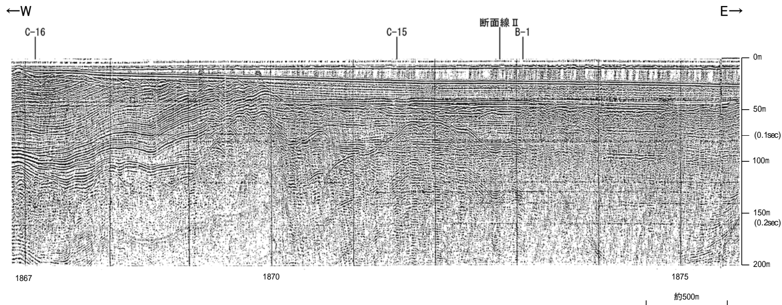
能登島半の浦断層帯
