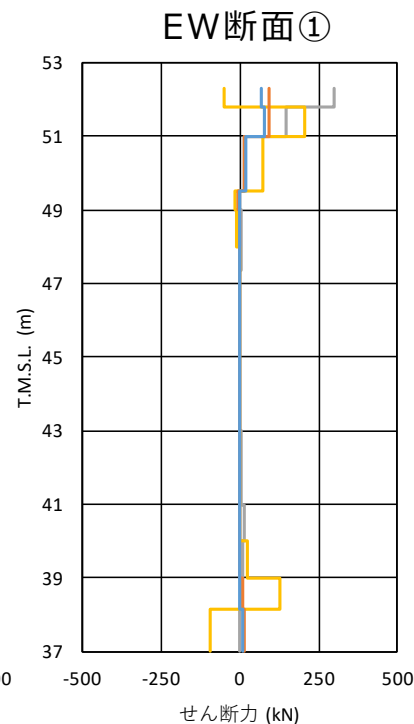
杭のせん断力分布 （検証用モデル）
