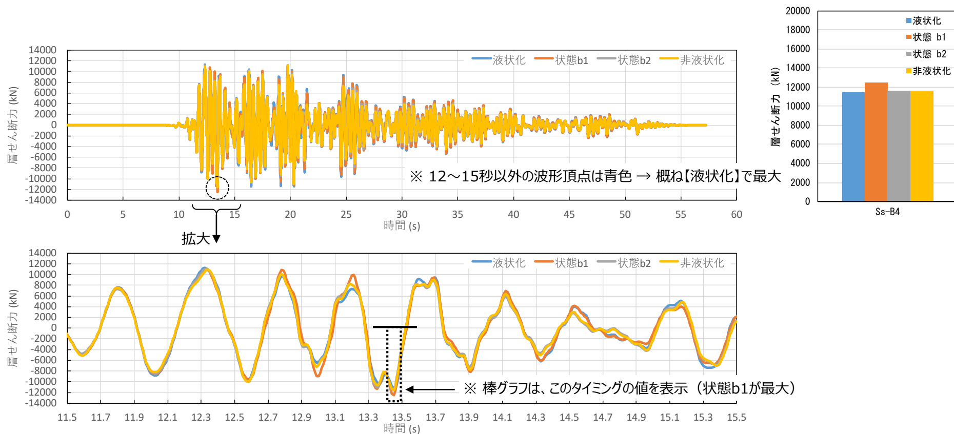
Ss-B4加振時の層せん断力の時刻歴
