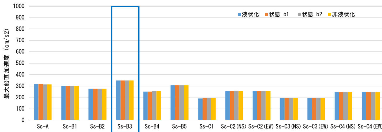
E)最大鉛直加速度 (基礎梁)
