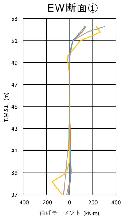
杭の曲げモーメント分布 （検証用モデル）
