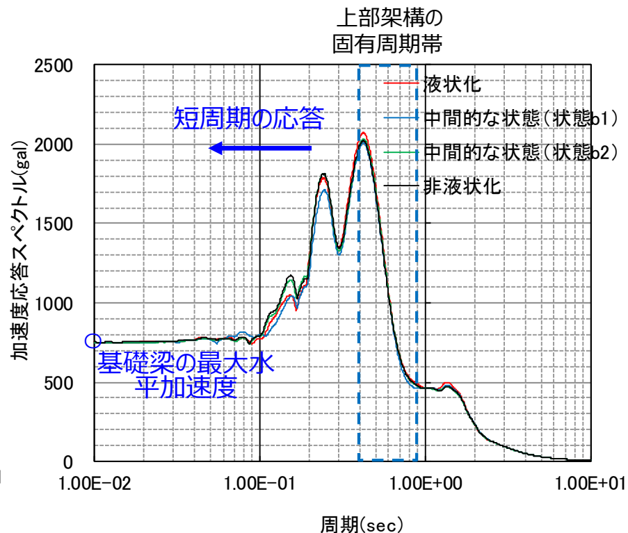
Ss-C1加振時の基礎梁上端の水平加速度応答スペクトル
