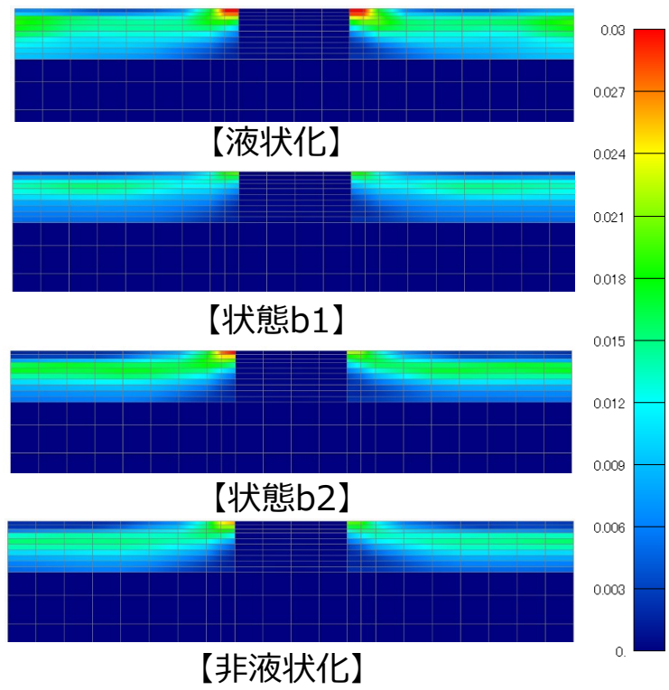
最大せん断ひずみの最大応答分布（Ss-C1加振時）
