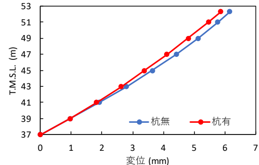
改良地盤の最大相対変位分布 b) Ss-C1
