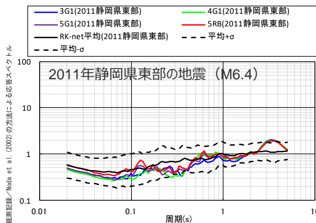
<地震観測記録とNoda et al.(2002)の方法による応答スペクトルの比（水平平均）>
