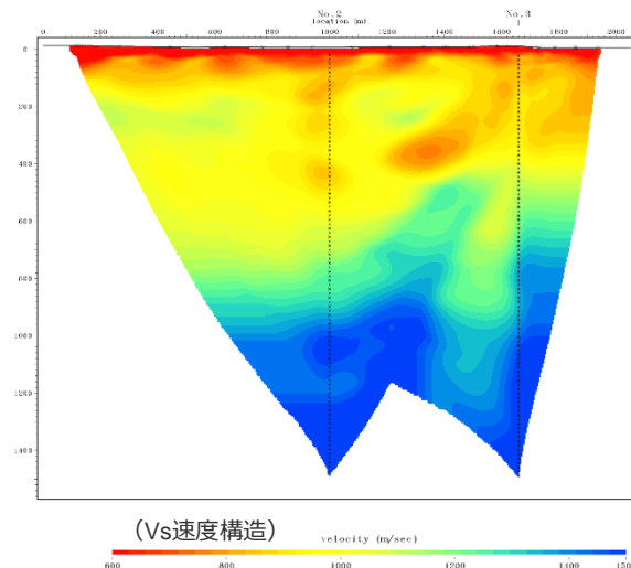
S波の初動解析結果（2-3測線）
