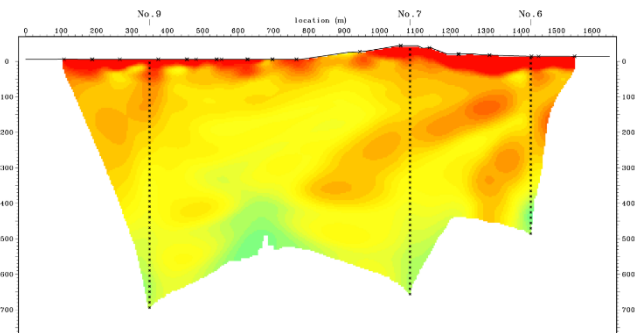
S波の初動解析結果（6-7-9測線）
