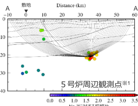
＜振幅比（No.7基準）の断面図（A-A'断面）＞
