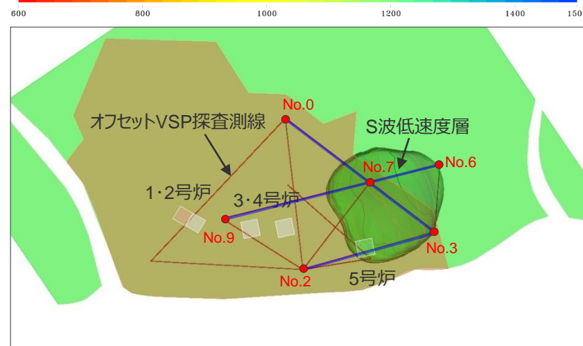
S波低速度層の分布 (平面図)
