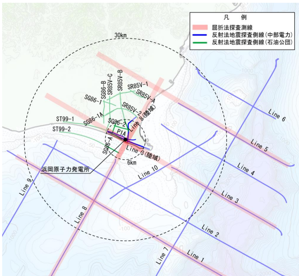
<層境界の設定に用いた地下構造調査>
