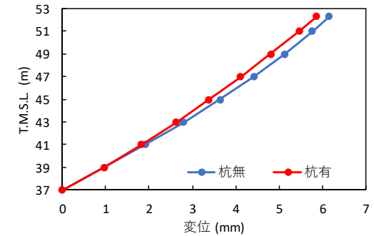
改良地盤の最大相対変位分布 a) Ss-A b) Ss-C1 応答値比較表
