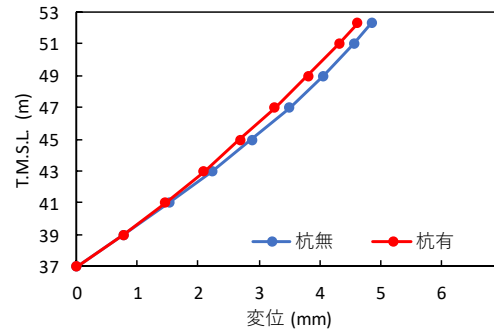
改良地盤の最大相対変位分布 a) Ss-A b) Ss-C1 応答値比較表
