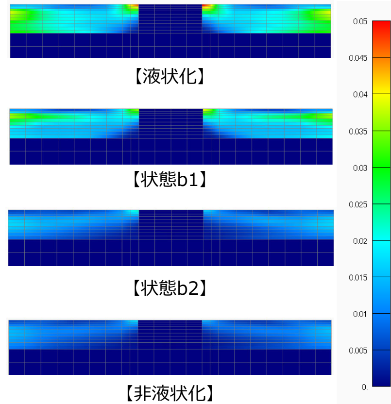
最大せん断ひずみの最大応答分布 (Ss-A加振時)
