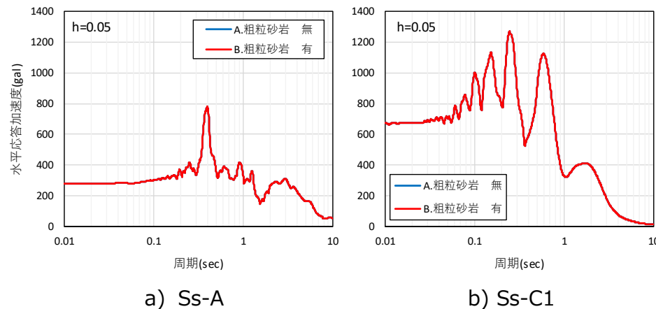
地表面（埋戻土上端）の水平加速度応答スペクトル
