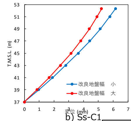
改良地盤の最大相対変位分布
