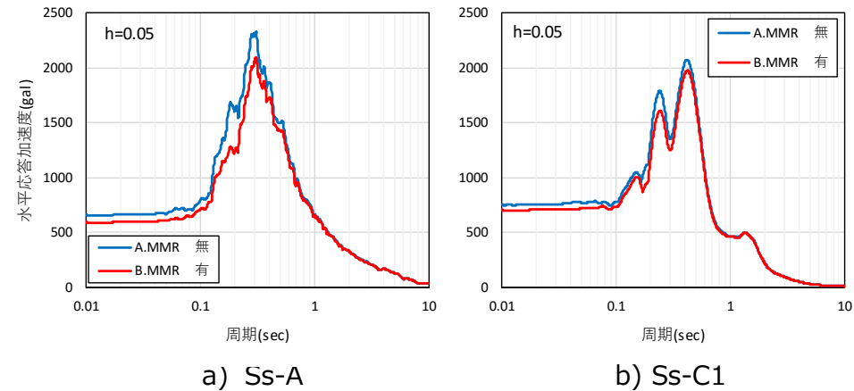
基礎梁部（T.M.S.L.+55.3m）の水平加速度応答スペクトル
