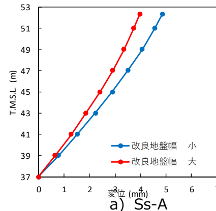
改良地盤の最大相対変位分布
