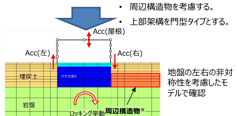
鉛直確認モデル
