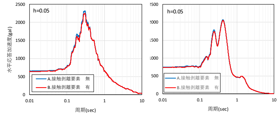
a) Ss-A 基礎梁部 (EL+55.3m) の水平加速度応答スペクトル b) Ss-C1
