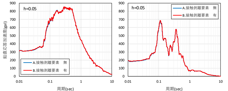
a) Ss-A 基礎梁部 (EL+55.3m) の鉛直加速度応答スペクトル b) Ss-C1
