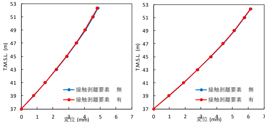
a) Ss-A 改良地盤の最大相対変位分布 b) Ss-C1
