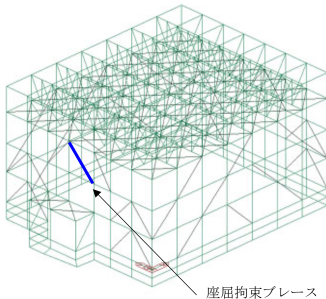
最大軸ひずみ発生位置
