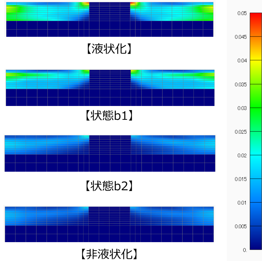
最大せん断ひずみの最大応答分布 (Ss-A加振時)
