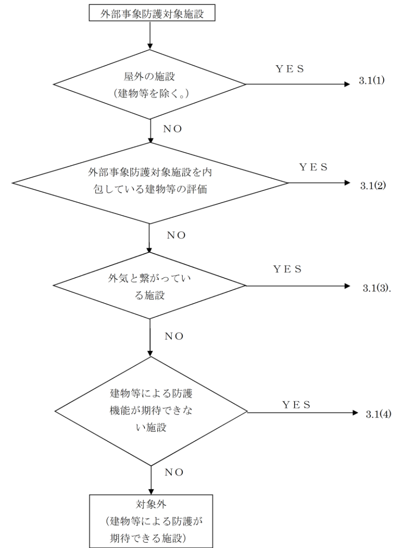
図 3-1 外部事象防護対象施設のうち竜巻の影響を考慮する施設の選定フロー
