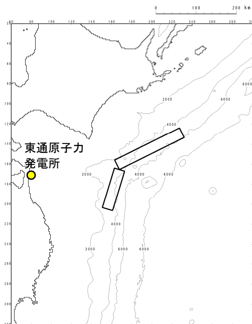
波源位置
