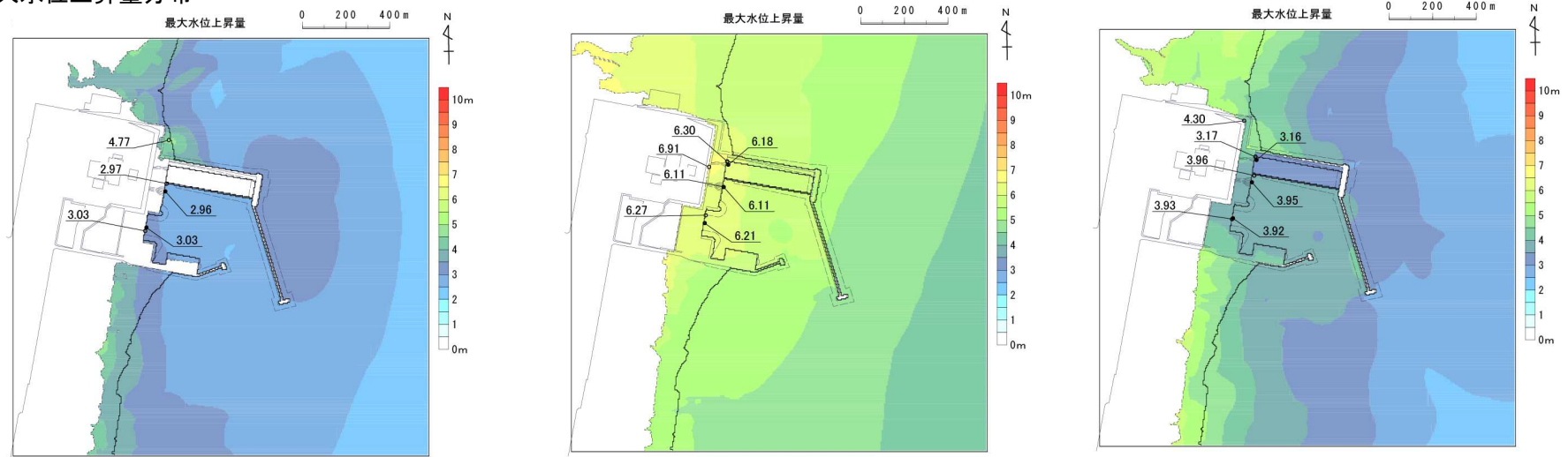
十勝沖・根室沖から千島前弧スリバー北東端の連動型地震
