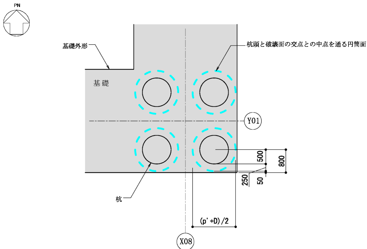
第 4.4.2-8 図 隅角部 P1 のはしあきと円筒面の関係
