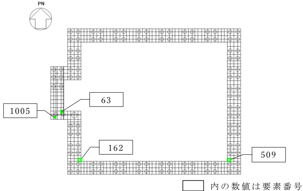
第4.4.2-1図 最大検定値発生位置（基礎応力）
