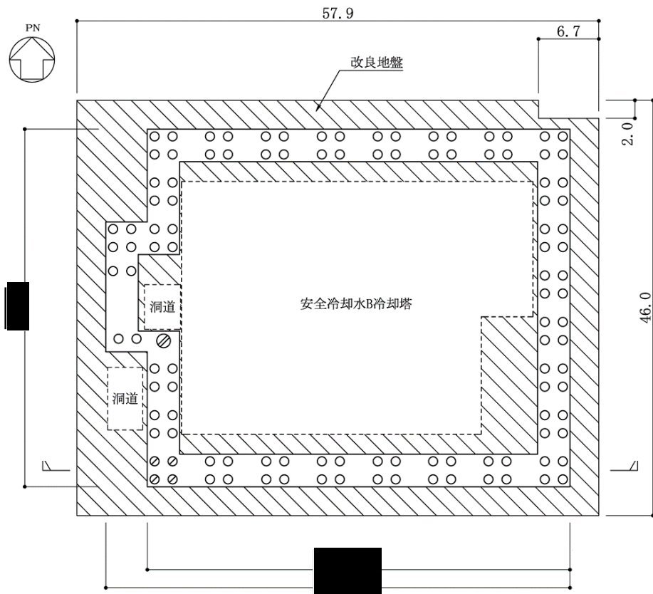
(平面図)
