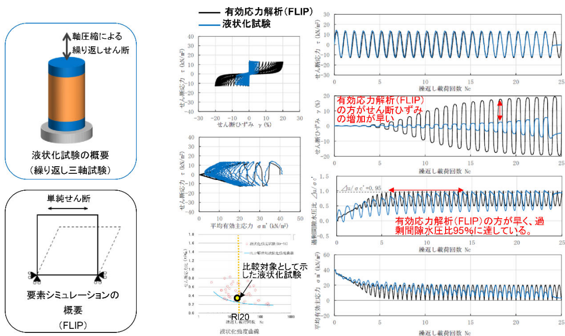
第 2-2 図 先行発電炉の埋戻し土を対象とした液状化試験と当社との対比
