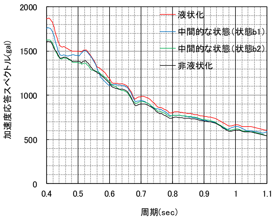
(b) 周期 0.4~1.1 秒
