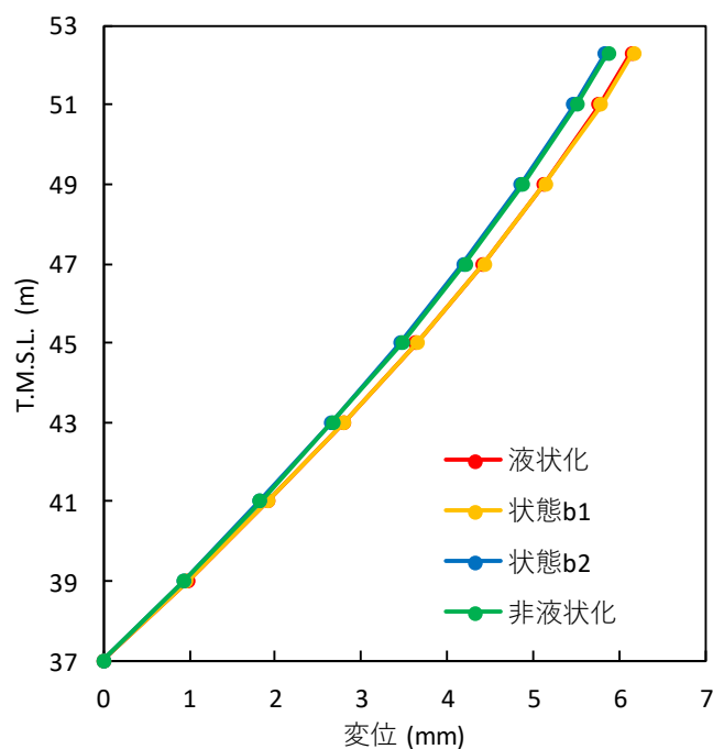
第 2.5.4-2 図 改良地盤の最大相対変位分布 (Ss-C1)
