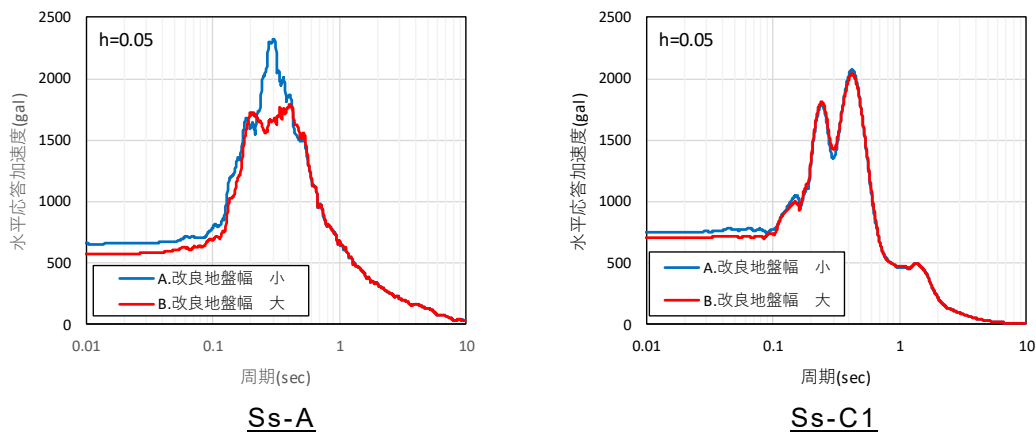
第 2.4.4-3 図 基礎梁部 (EL+55.3m) の水平加速度応答スペクトル
