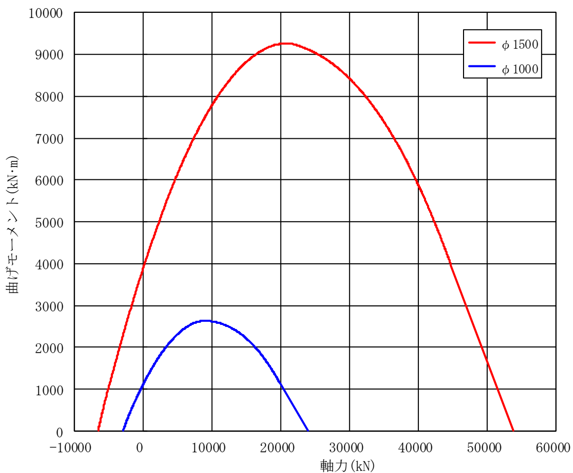
第 4.4.1-7 図 許容限界（Nu-Mu 関係）
