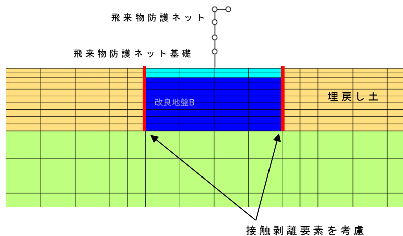
第 2.4.3-1 図 接触剥離を考慮する場合の箇所
