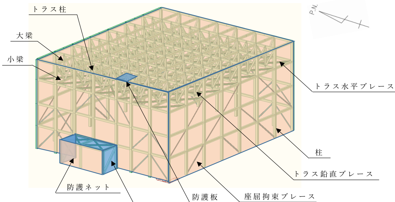
第 1.1.1-1 図 飛来物防護ネット 概要図
