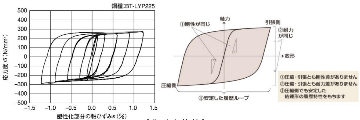
《復元力特性》
