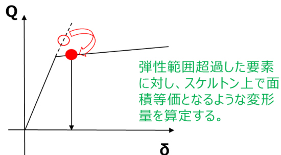
第 3.3-4 図 非線形化の影響の考慮方法
