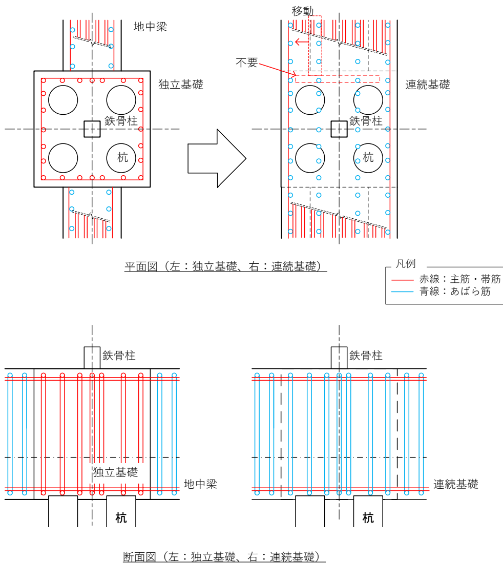
第4.1.1-3図 基礎配筋例(1/2)：(平面図，長辺方向断面図)
