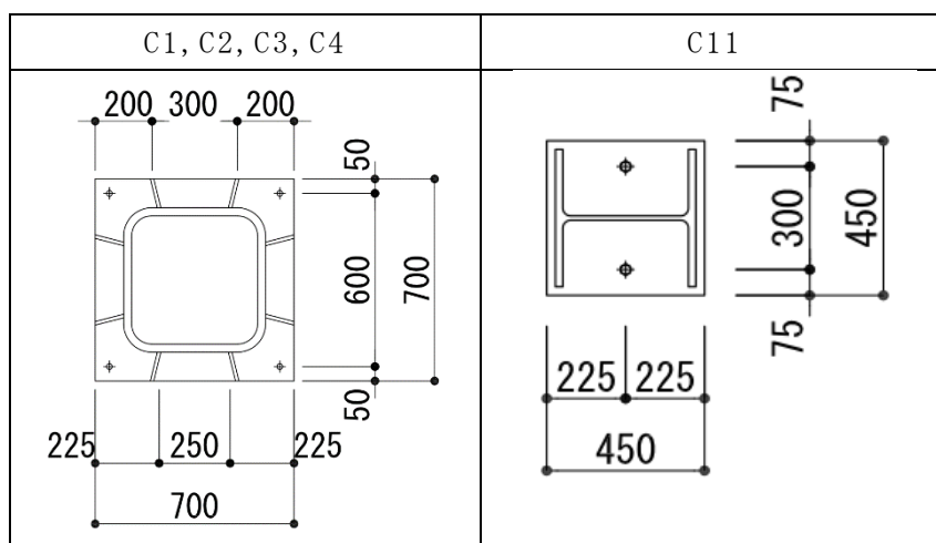
第 4.4.2-10 図 ベースプレート形状図
