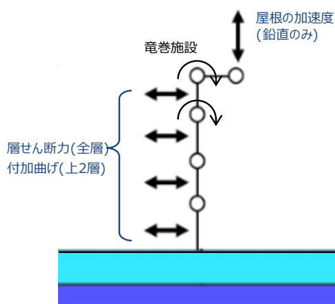
第 3.2.2-2 図 全応力/有効応力解析結果から引用する応答値
