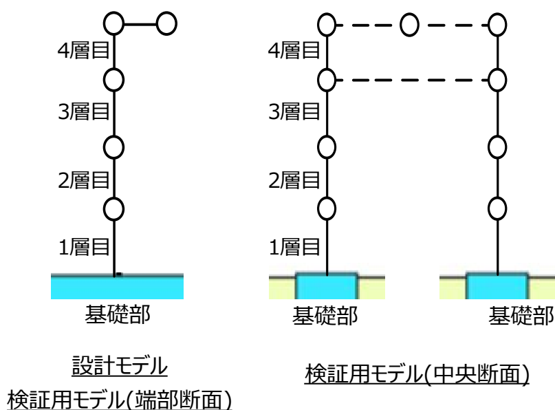
第2.5.5-1図 最大せん断力・曲げモーメントを算定する層
