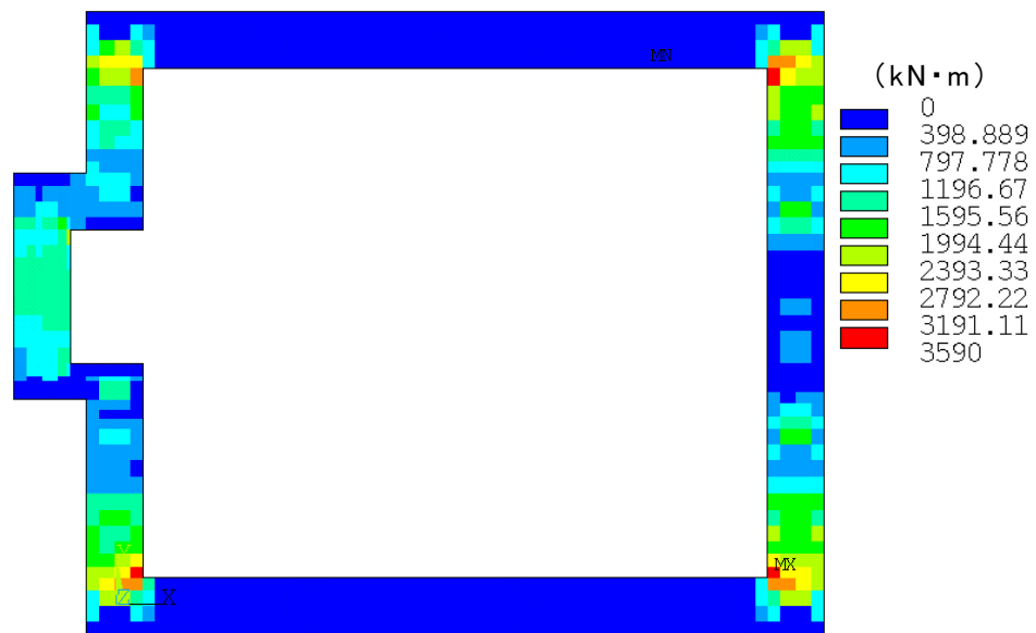
第 4.4.1-4 図 曲げモーメント図 (包絡 M_y )
