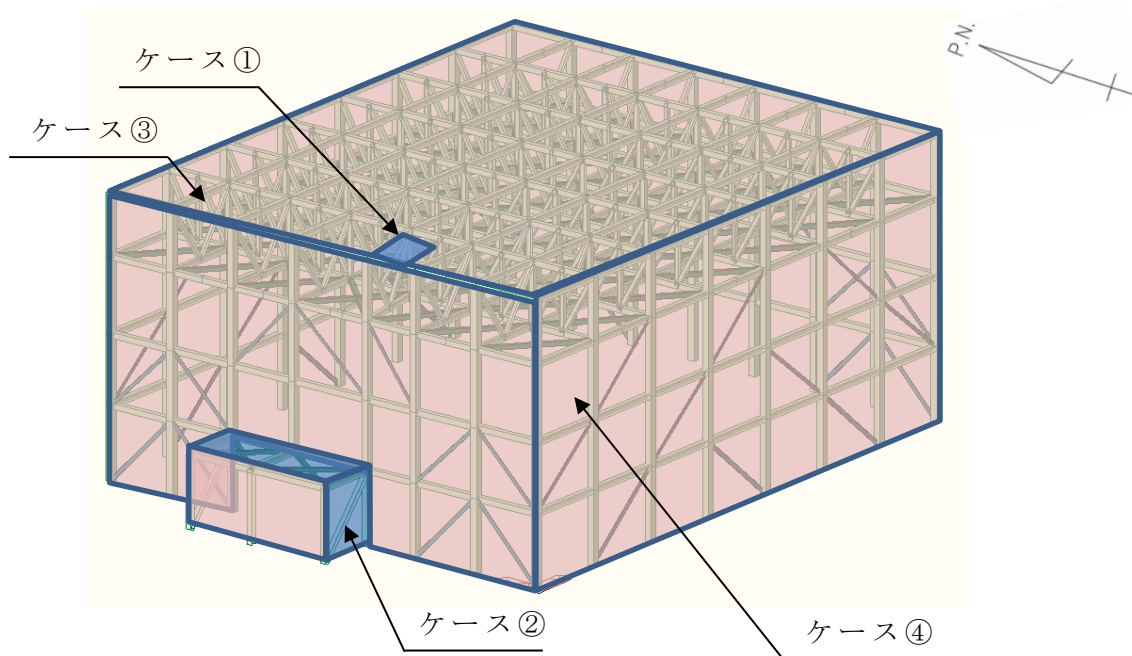
第2-1図 評価対象部位
