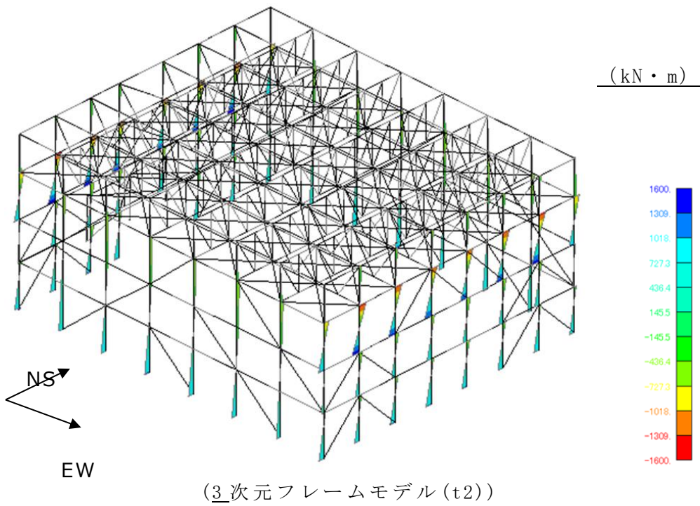
第 3.2.2-1 図 3次元フレームモデルのモーメント図(NS方向)(1/2)
