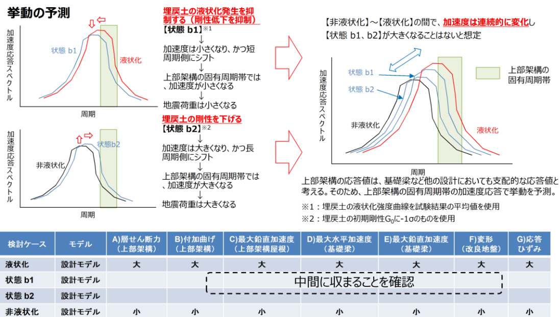
第 2.5.4-1 図 液化化の中間状態のイメージ図
