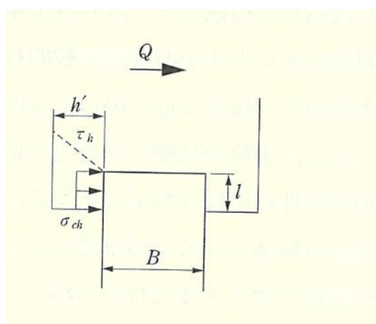
第4.4.2-9図 杭頭接合部の水平力に対する評価イメージ図
