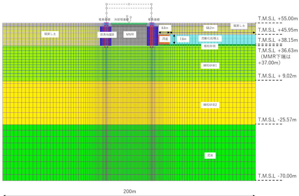
第 2.3.2-2 図 検証用モデル断面①-NS
