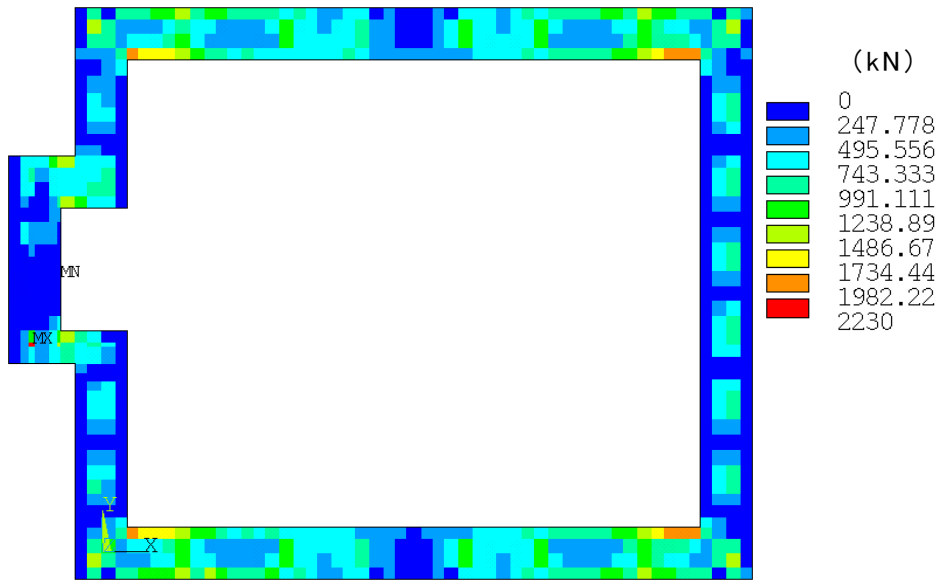
第 4.4.1-5 図 面外せん断力図 (包絡 Q_x )
