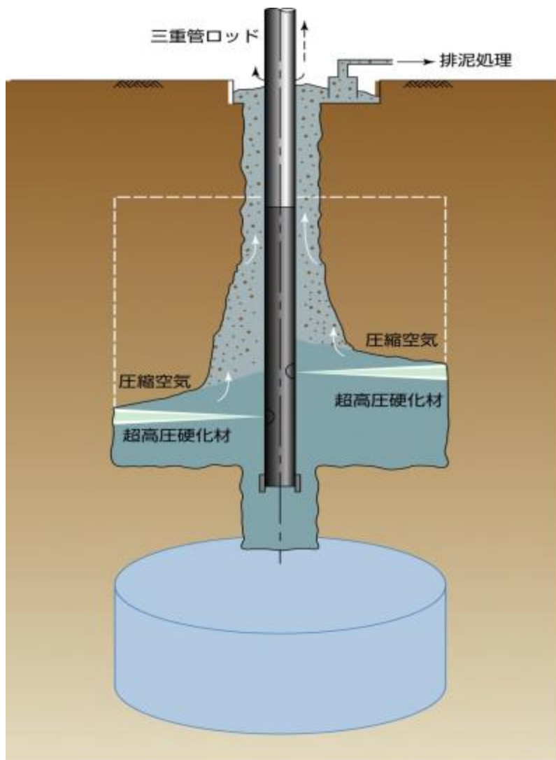
第 2.2-1 図 改良概要図
