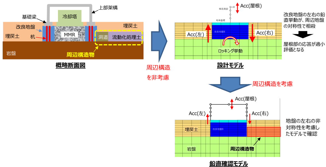
第 2.5.7-1 図 解析モデルと周辺構造物の関係による鉛直応答
