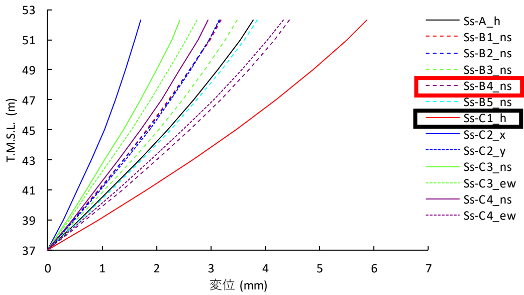
第 3-5 図 改良地盤の最大変位 (基本ケース, NS 方向, 全応力解析)
