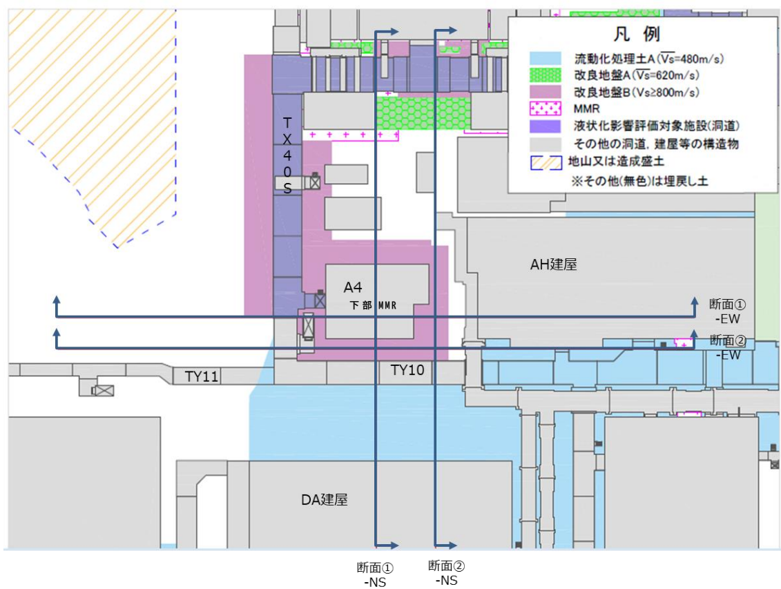
第 2.3.2-1 図 検証用モデルの検討断面
