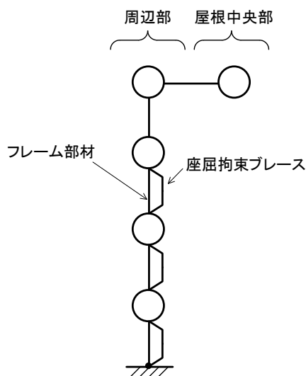
第 3.2.1-1 図 全応力/有効応力解析質点系モデル
