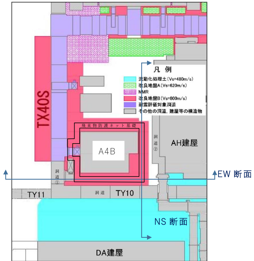
第 2.3.1-1 図 飛来物防護ネット近傍の平面図
