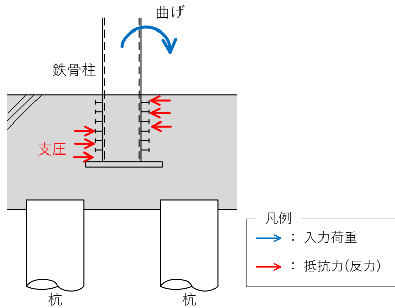
第4.2.3-1図 上部架構から基礎への水平力の伝達
