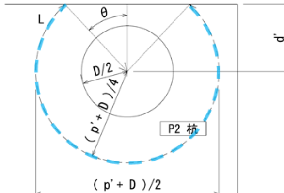
第 4.4.2-7 図 はしあきが小さい P2 における有効領域
