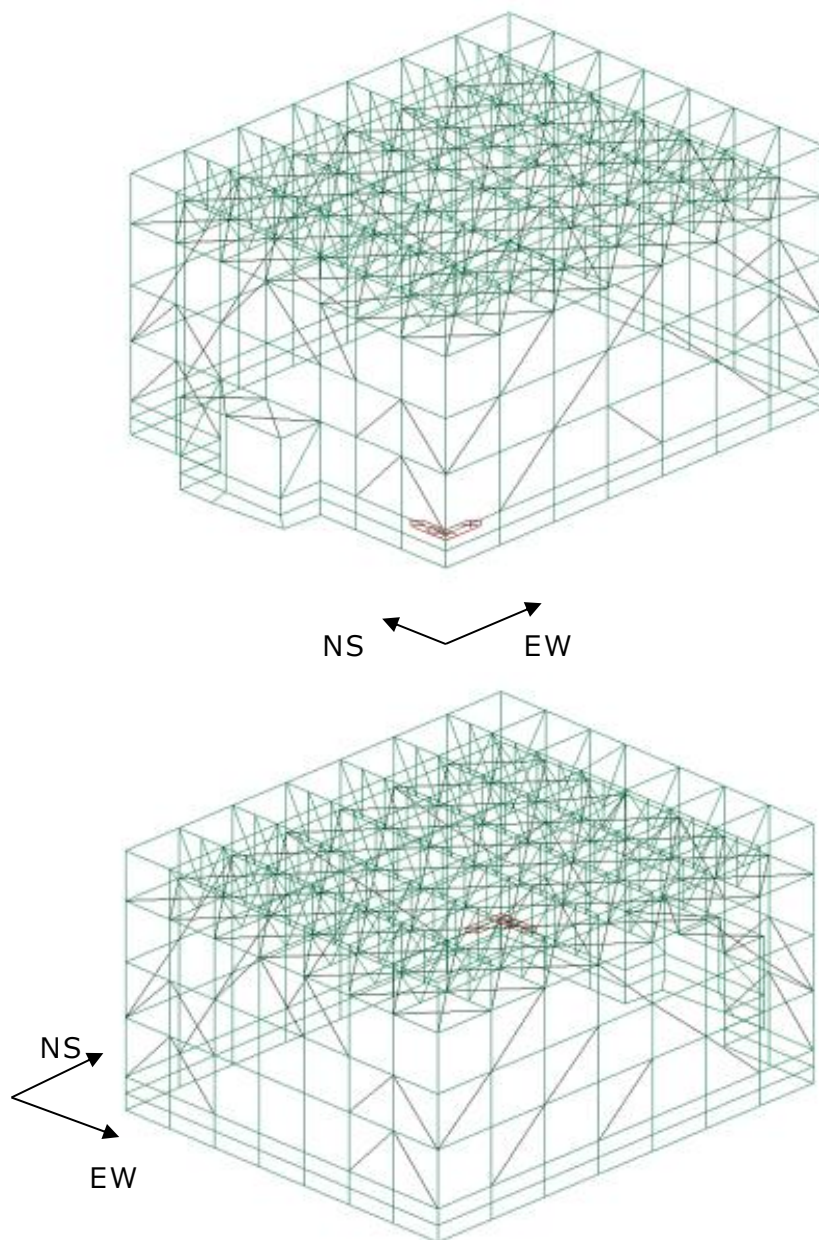
第3.2-1図 飛来物防護ネットの応力解析に用いる3次元フレームモデル
