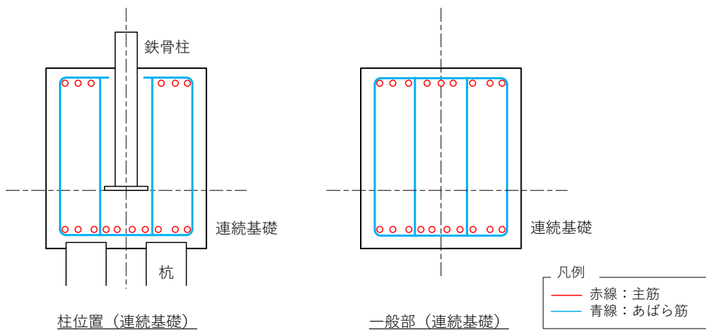
第 4.1.1-3 図 基礎配筋例 (2 / 2) : (短辺方向断面図)
