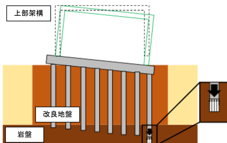
第3.5-1図 杭基礎の沈下イメージ
