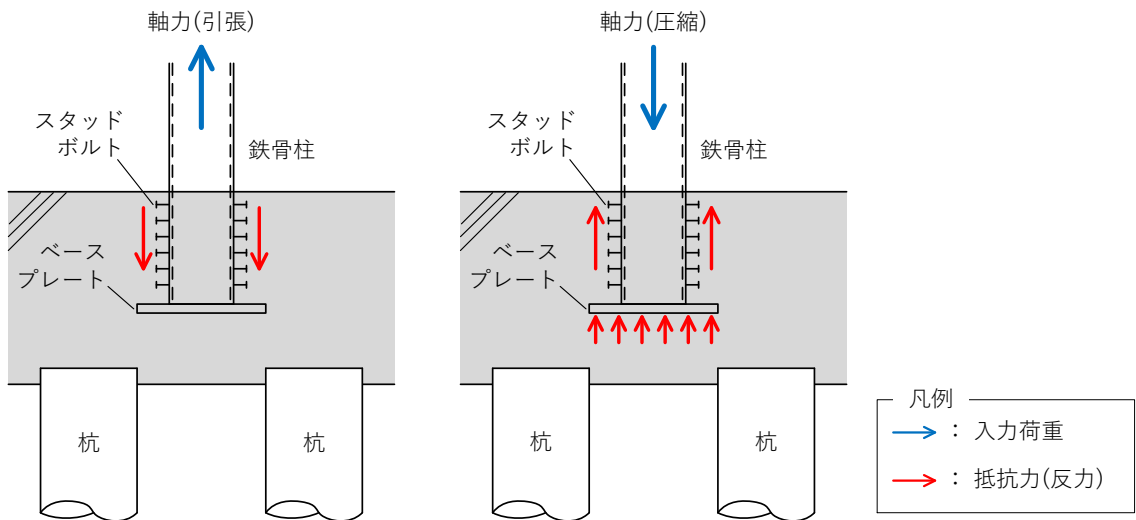
第4.2.2-1図 上部架構から基礎への軸力の伝達
