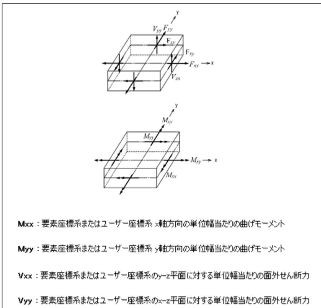
第 4.4.1-2 図 応力の向きと符号 (MIDAS マニュアルより)
