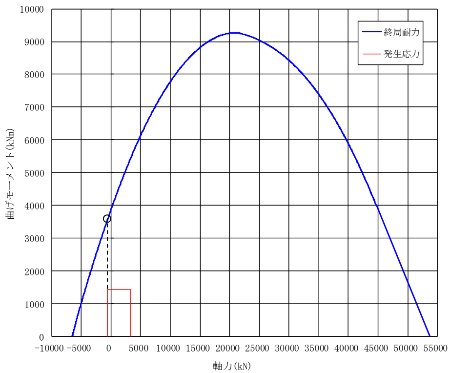
第 4.4.2-3 図 杭体の軸力及び曲げモーメントに対する評価結果
