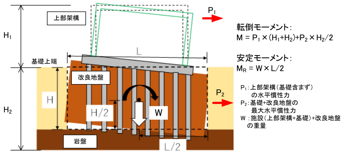
第 3.5-2 図 杭基礎の転倒イメージ
