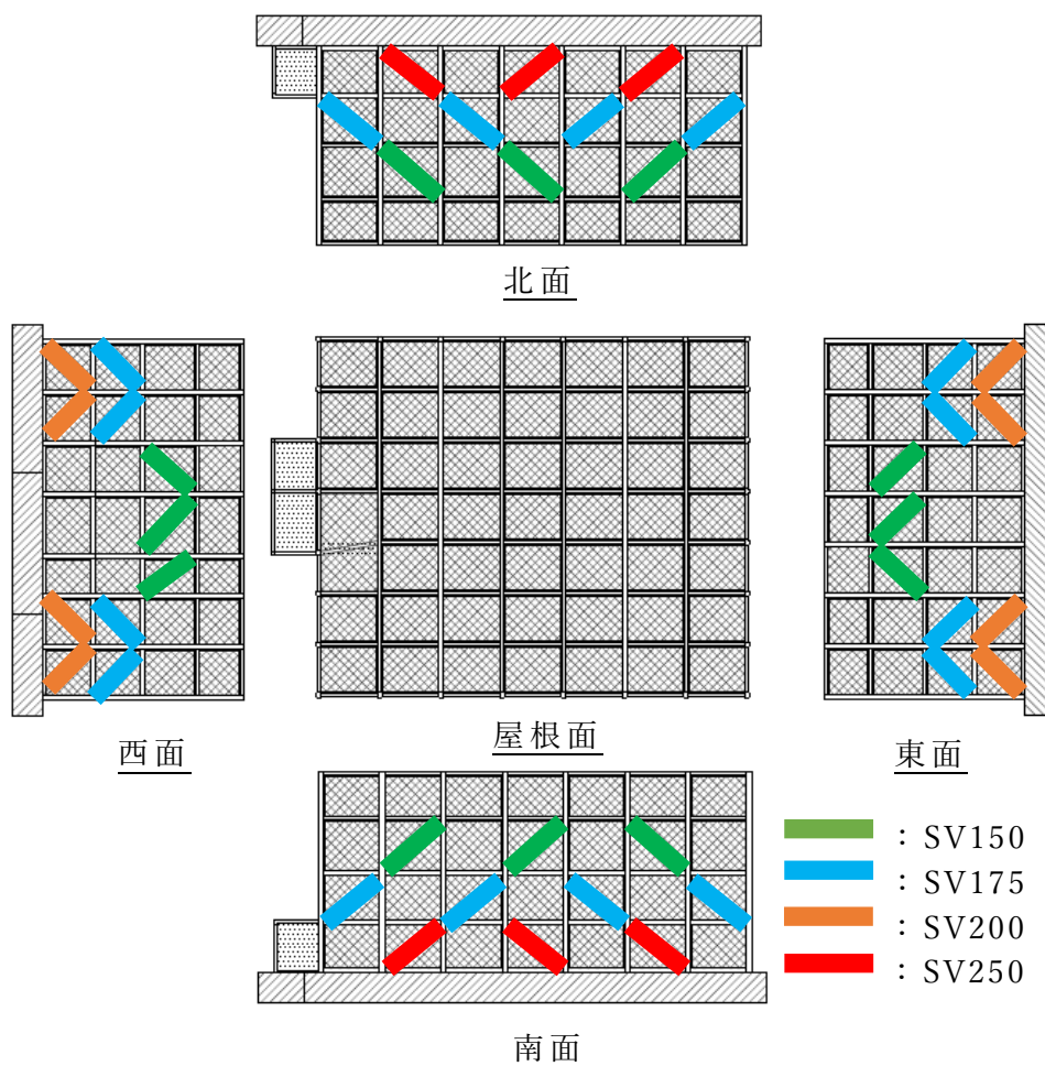
第 1.1.2-2 図 座屈拘束ブレースの設置状況
