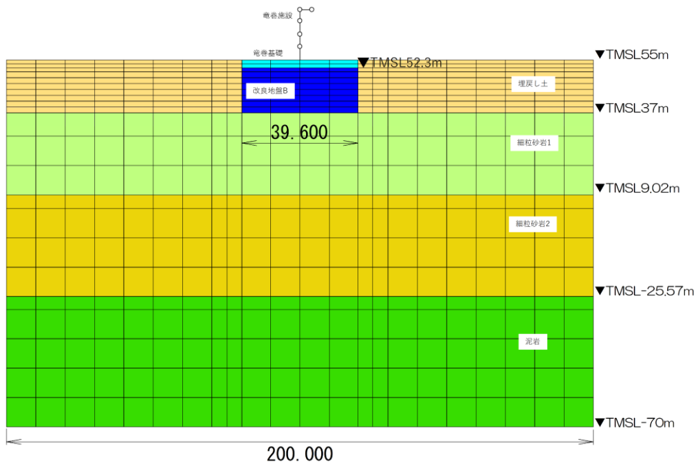
第 2.3.3-1 図 設計モデル NS 断面
