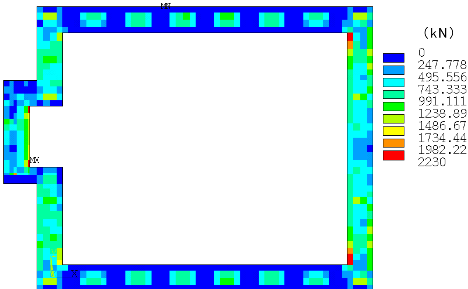
第 4.4.1-6 図 面外せん断力図 (包絡 Q_y )
