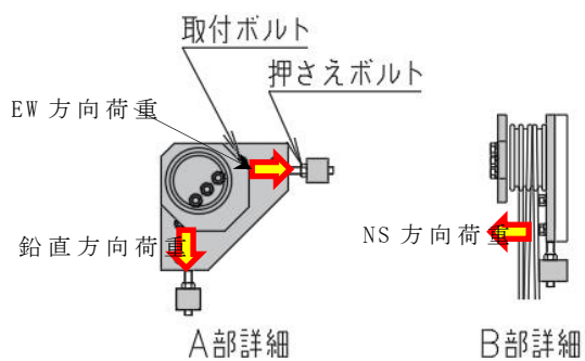
第 4-4 図 ケース④の荷重作用図
