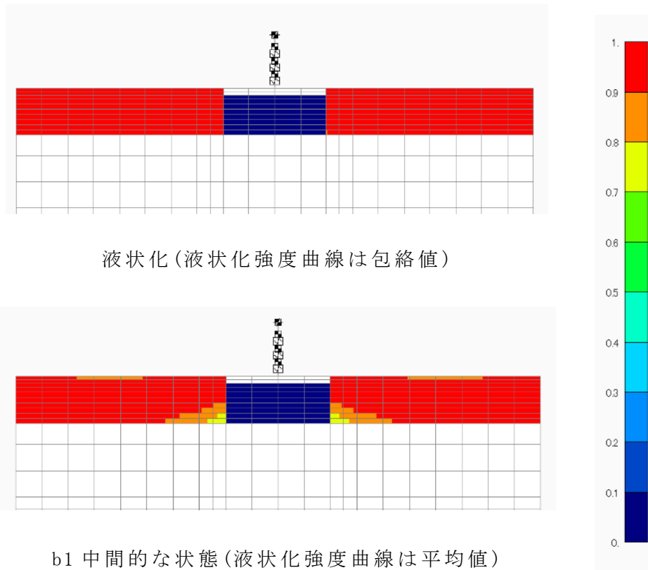
第 2.5.4-5 図 最終時刻の過剰間隙水圧比分布 ( S_s-A )
