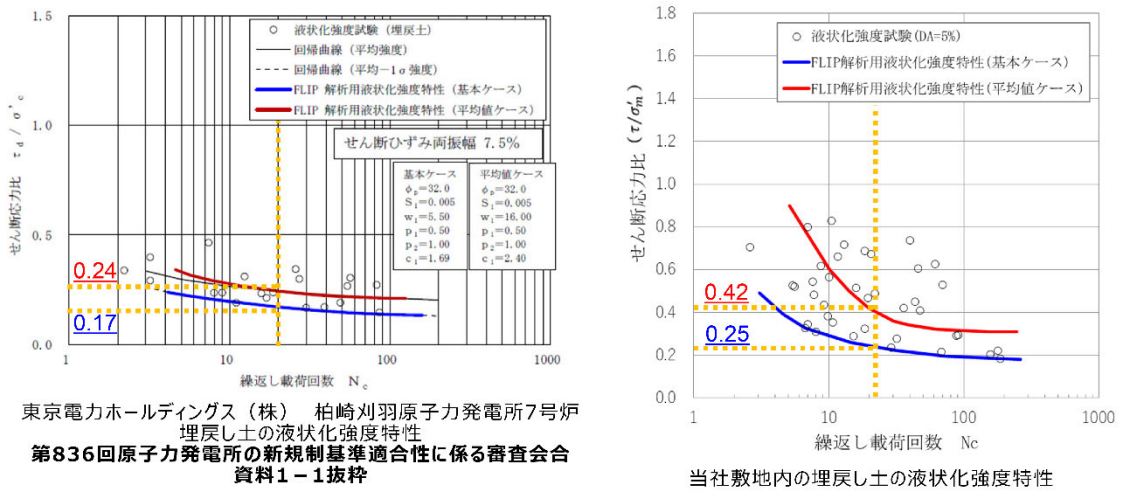
第2-1図 KK7の埋戻し土の液状化強度特性と当社との比較
