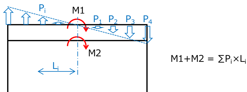
第3.2.2-4図 屋根トラスの付加曲げの分配方法
