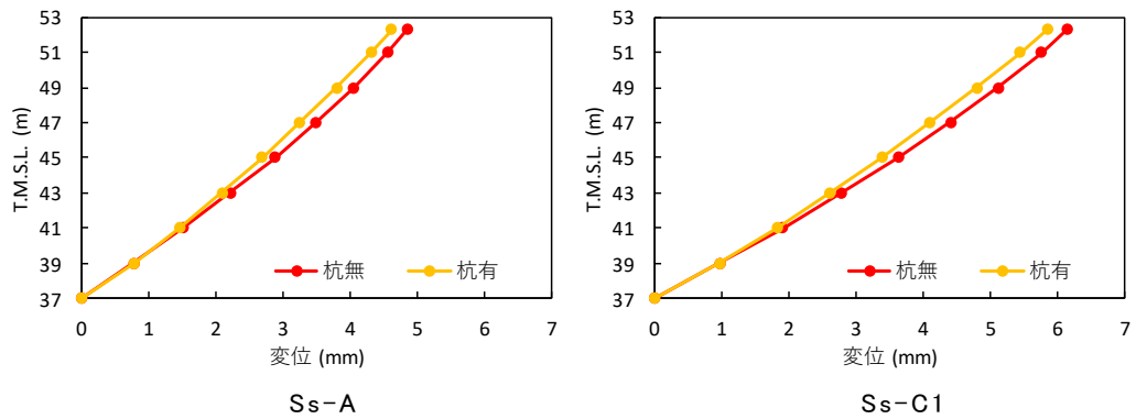
第 2.5.2-2 図 改良地盤の最大相対変位置
