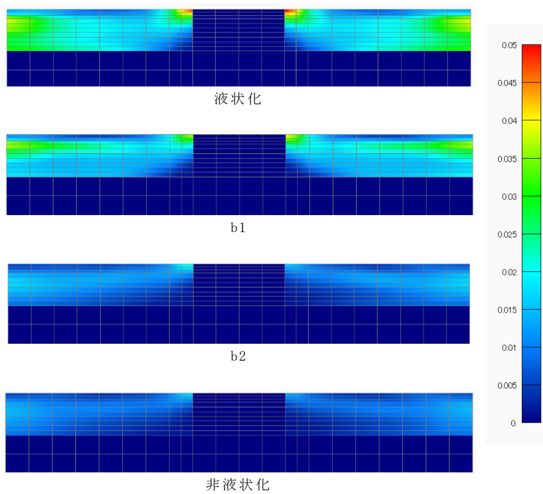
第 2.5.4-6 図 最大せん断ひずみの最大応答分布 (Ss-A)
