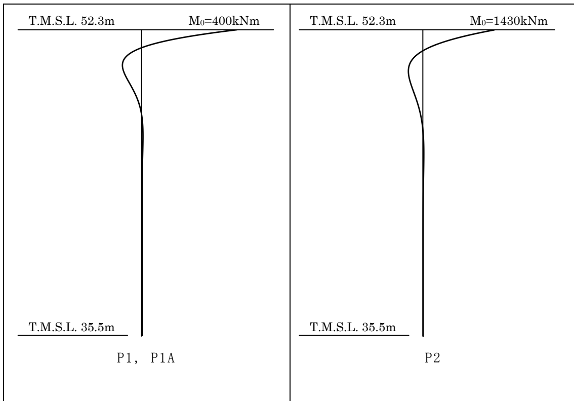
第 4.4.2-4 図 杭モーメント図
