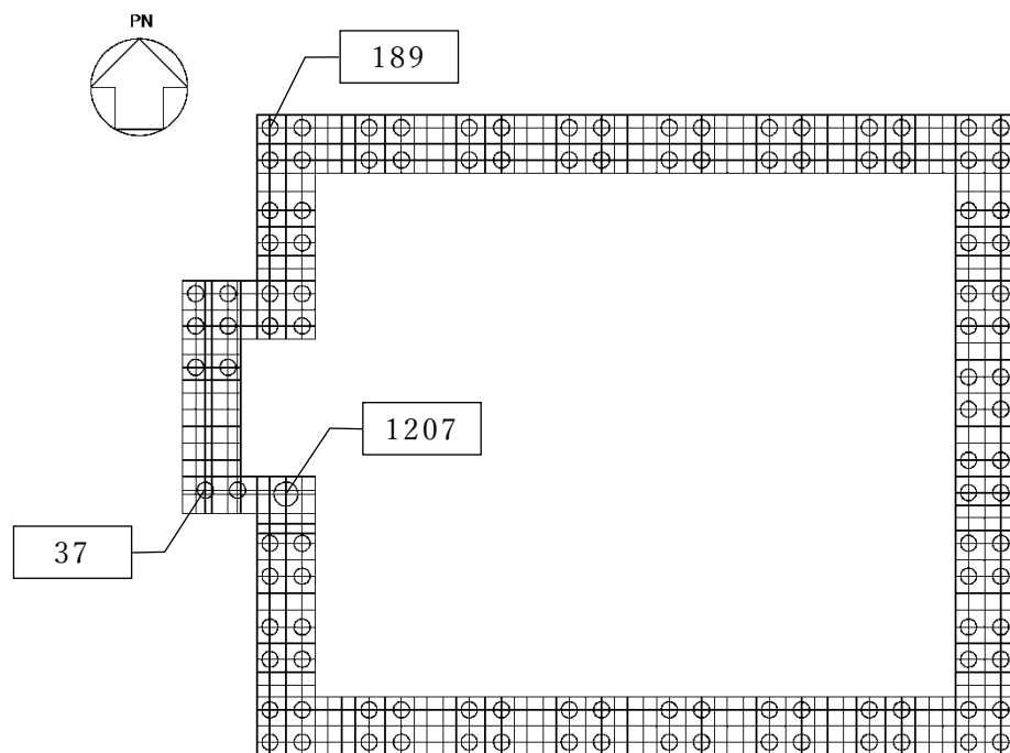
第 4.4.2-5 図 最大検定値発生位置（支持力及び引抜力）
