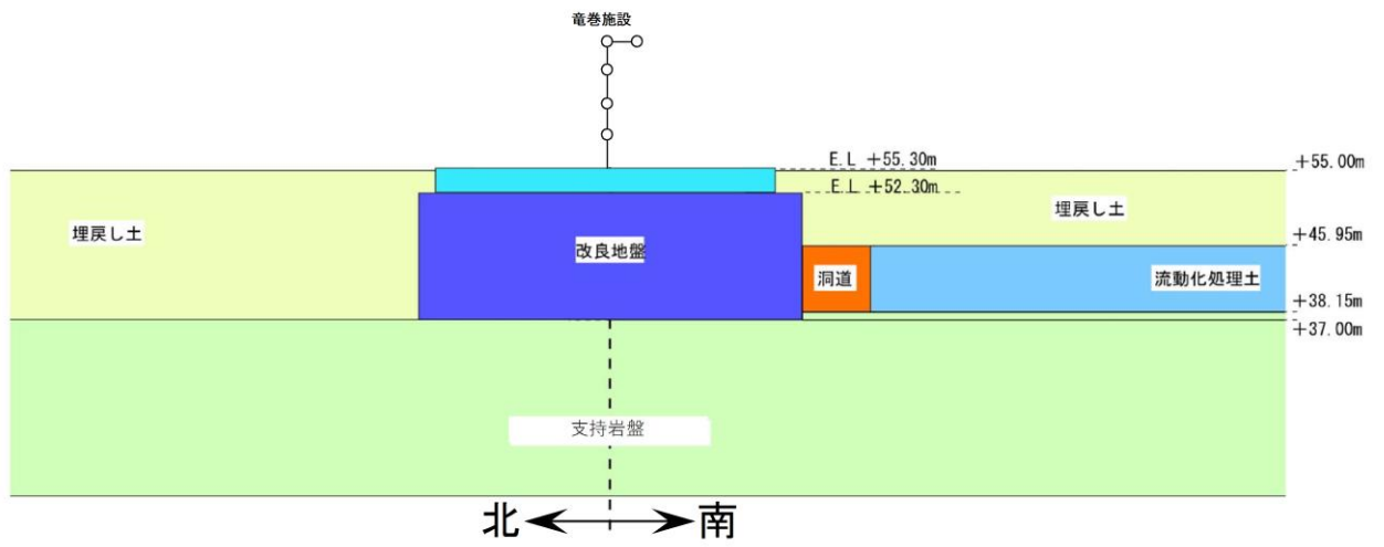
第 2.3.1-2 図 NS 断面
