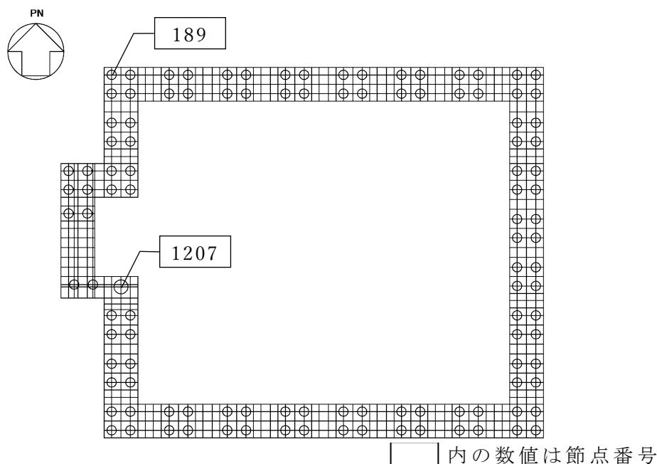
第 4.4.2-2 図 最大検定値発生位置（杭応力）
