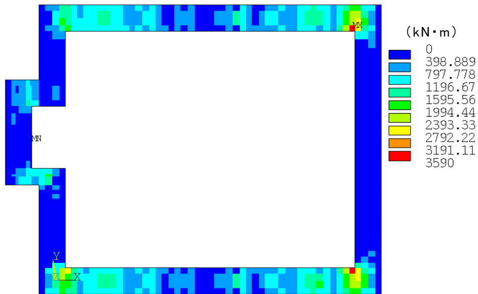
第 4.4.1-3 図 曲げモーメント図 (包絡 M_x )
