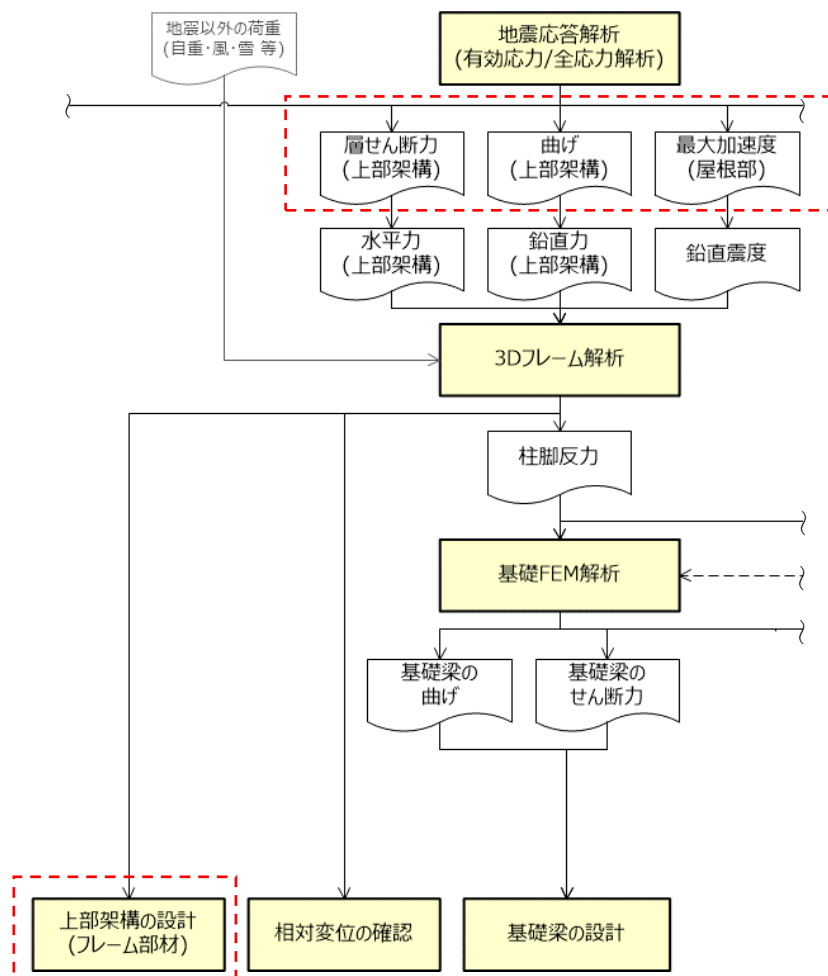
第2.5.6-1図 解析・設計フロー(抜粋)
