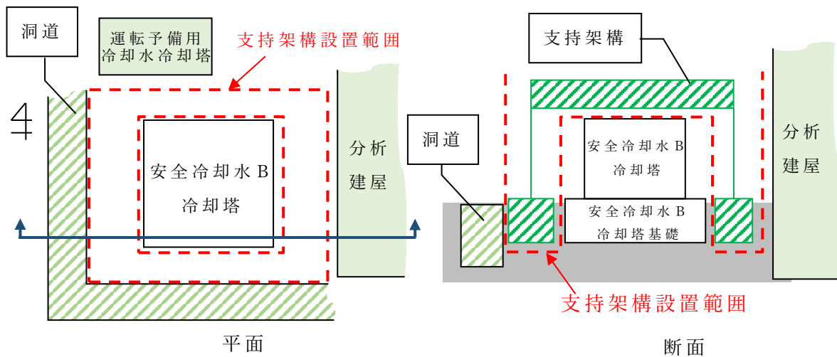
第 1.1.2-1 図 飛来物防護ネットの支持架構の配置制約
