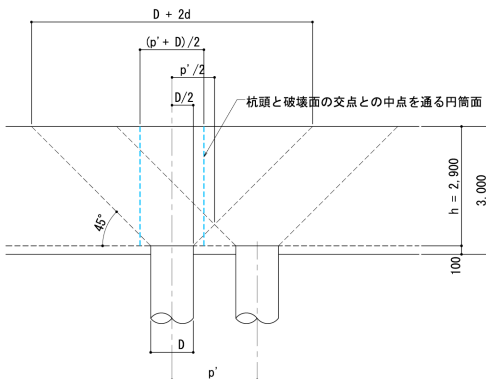
第4.4.2-6図 杭頭部構造図
