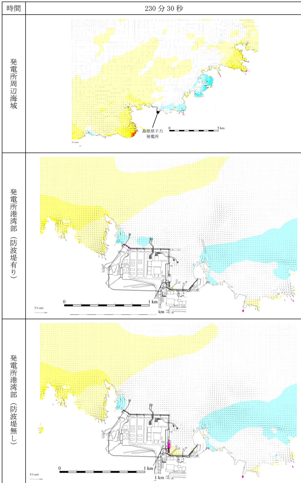
図 1-262 基準津波 1 の水位変動・流向ベクトル
