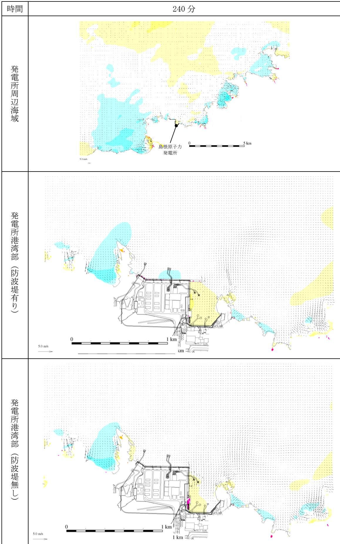
図 1-281 基準津波 1 の水位変動・流向ベクトル
