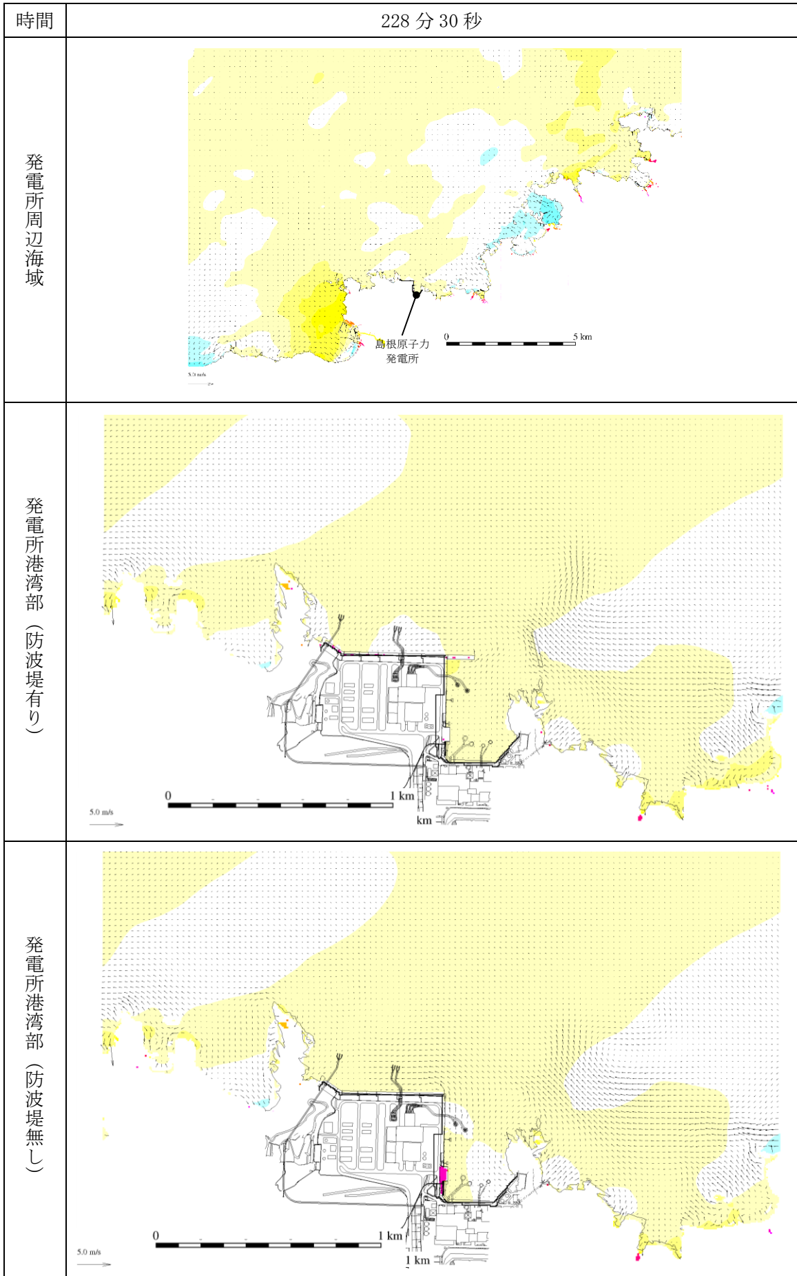
図 1-258 基準津波 1 の水位変動・流向ベクトル
