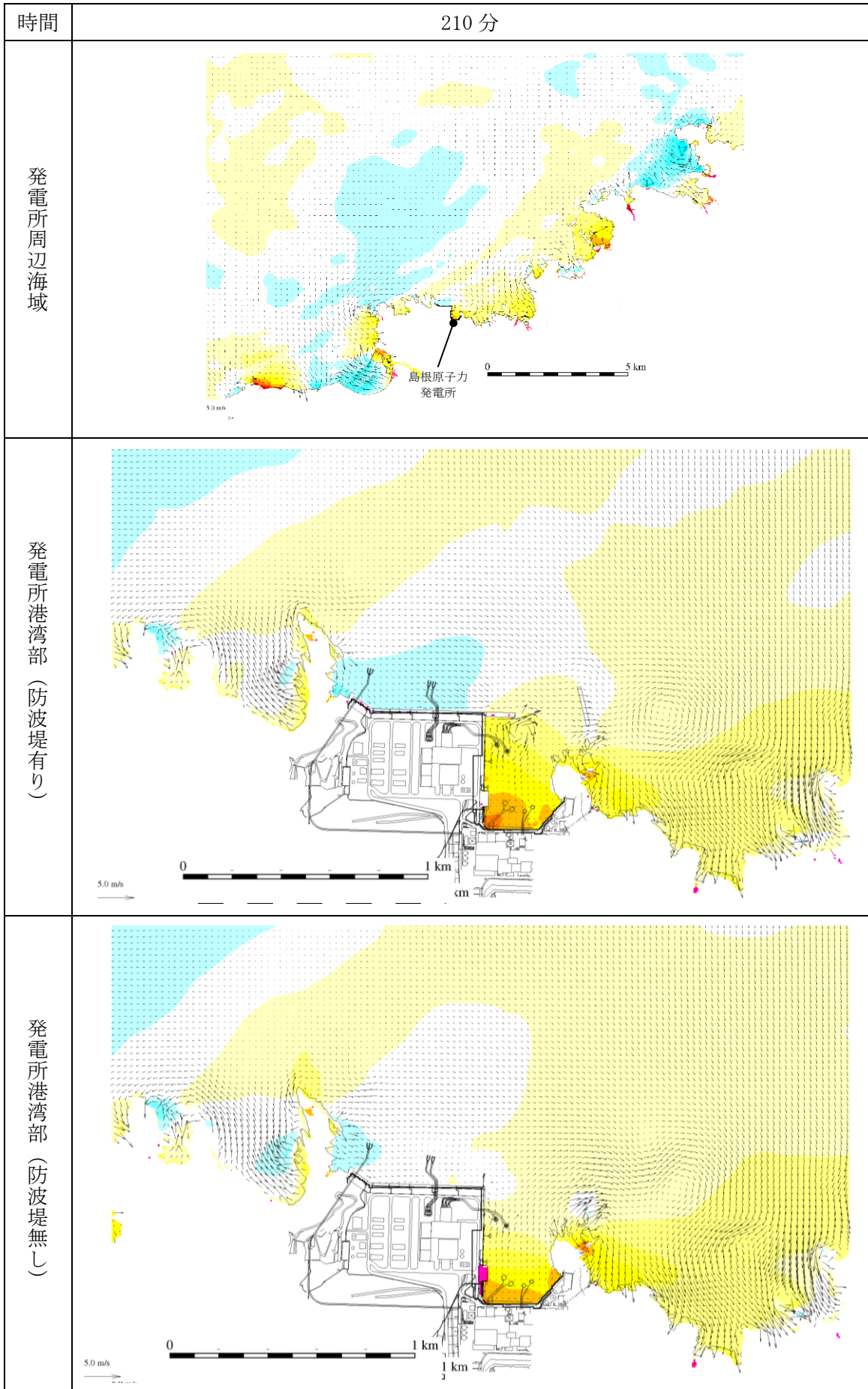
図 1-221 基準津波 1 の水位変動・流向ベクトル
