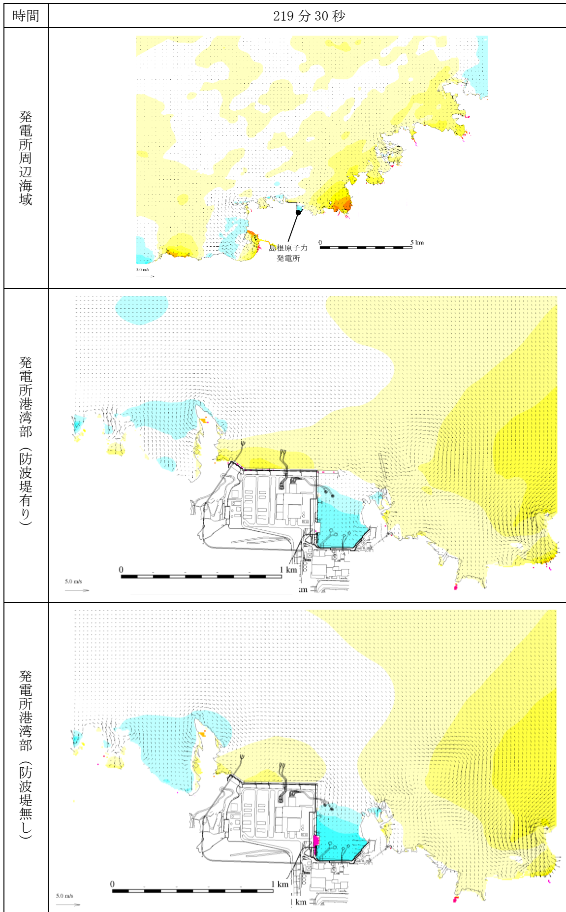
図 1-240 基準津波 1 の水位変動・流向ベクトル
