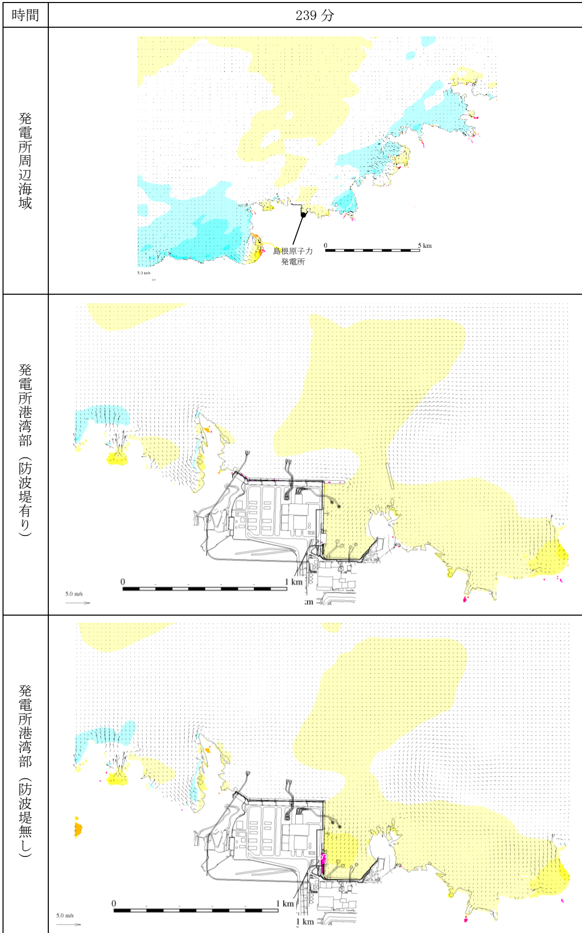
図 1-279 基準津波 1 の水位変動・流向ベクトル
