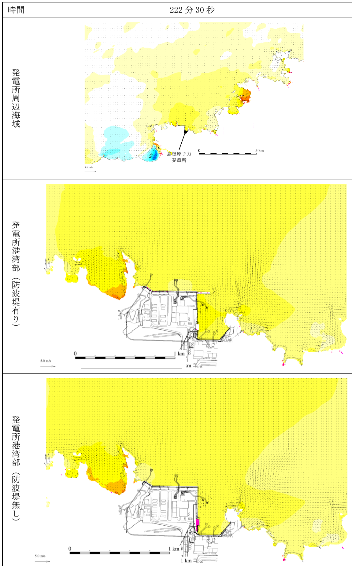
図 1-246 基準津波 1 の水位変動・流向ベクトル
