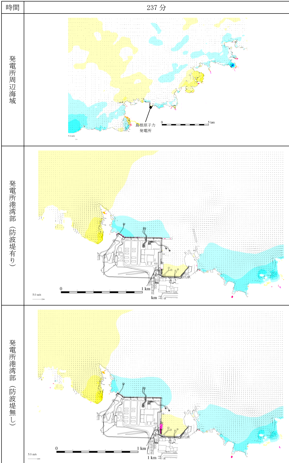
図 1-275 基準津波 1 の水位変動・流向ベクトル
