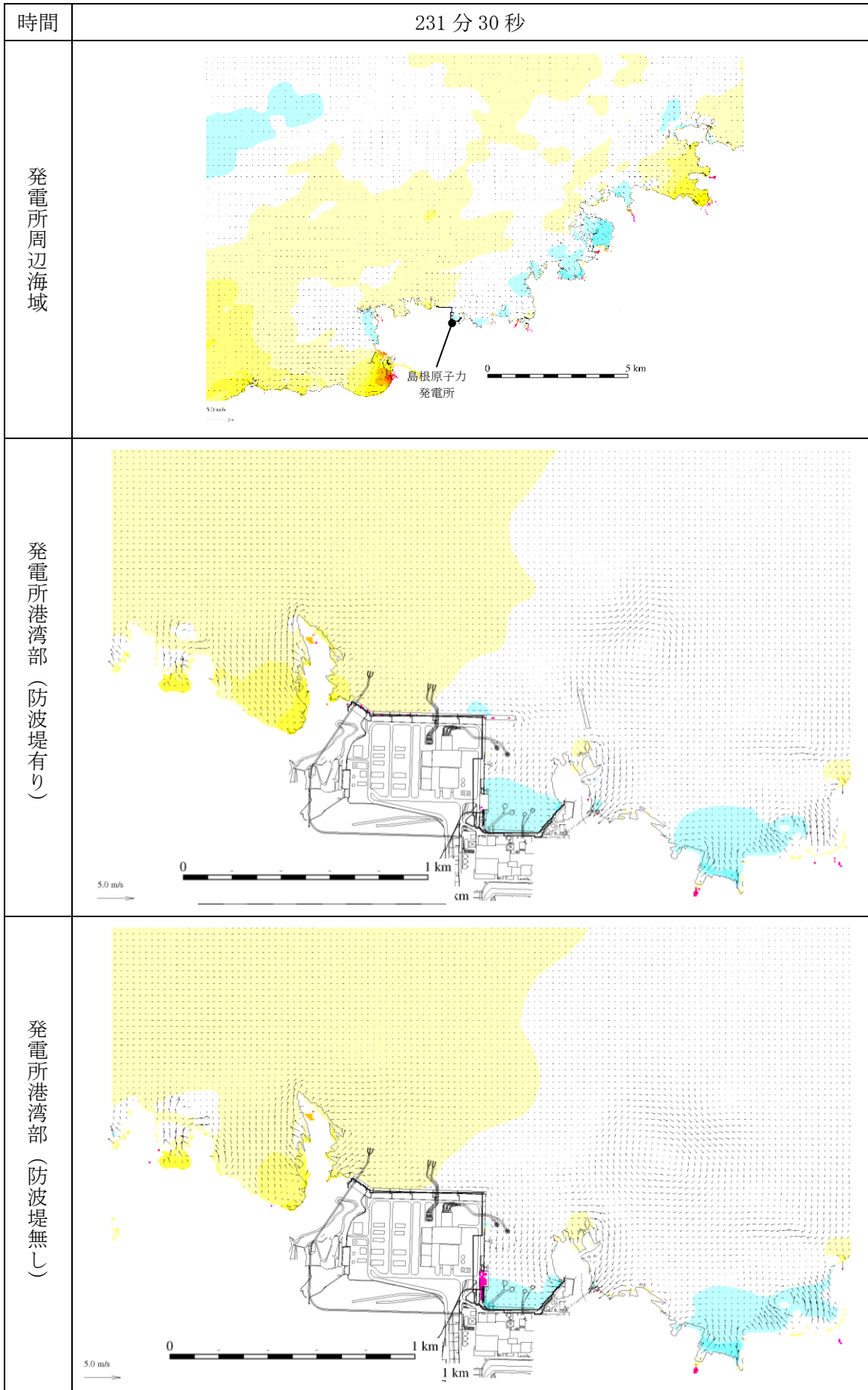
図 1-264 基準津波 1 の水位変動・流向ベクトル
