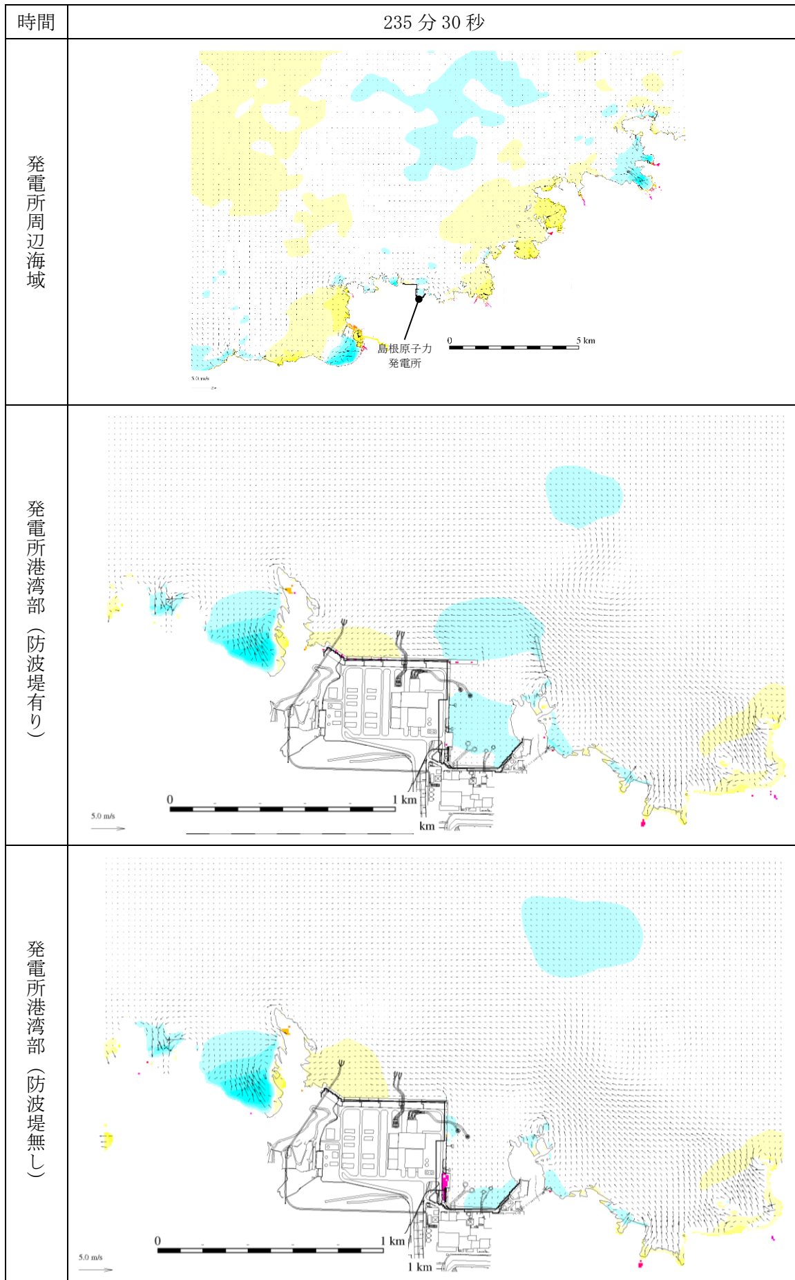
図 1-272 基準津波 1 の水位変動・流向ベクトル
