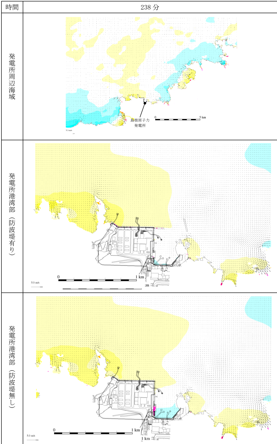
図 1-277 基準津波 1 の水位変動・流向ベクトル
