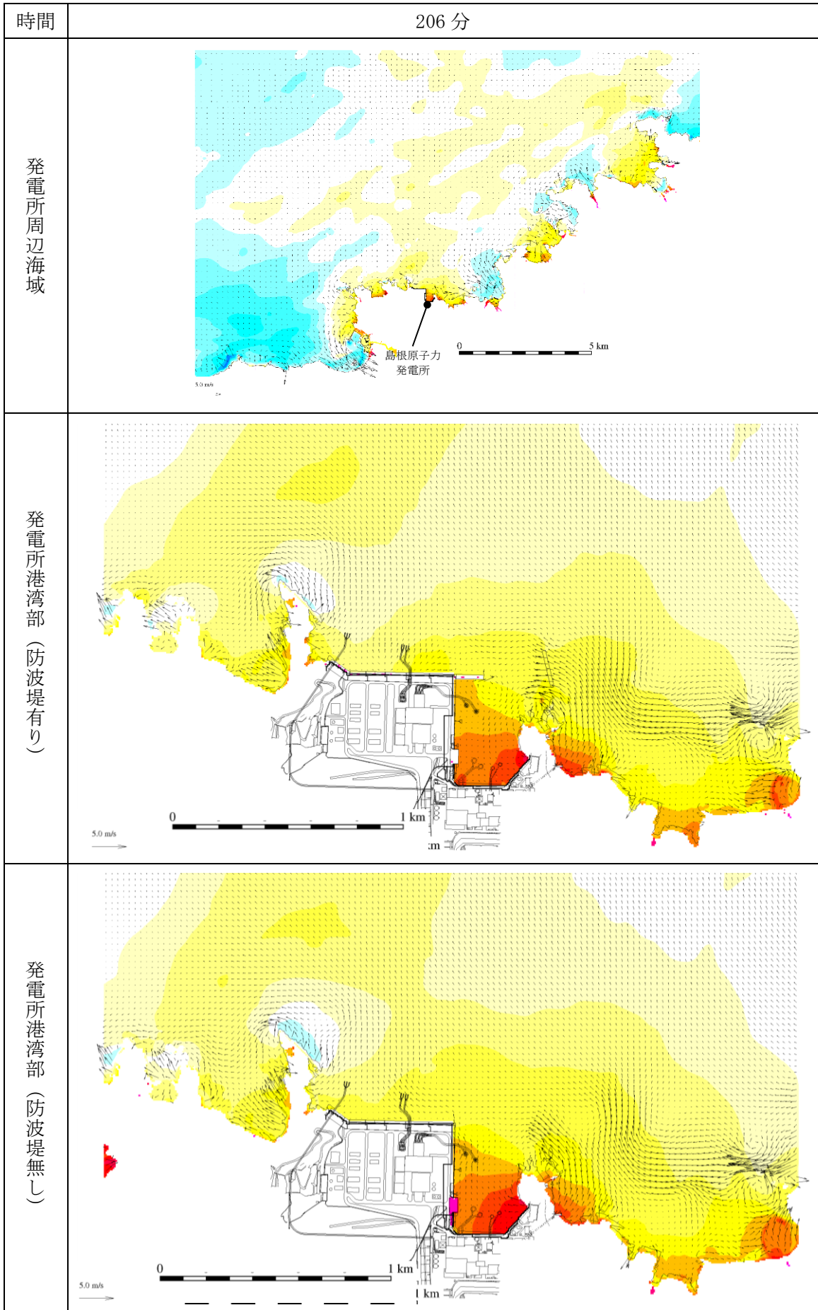
図 1-213 基準津波 1 の水位変動・流向ベクトル
