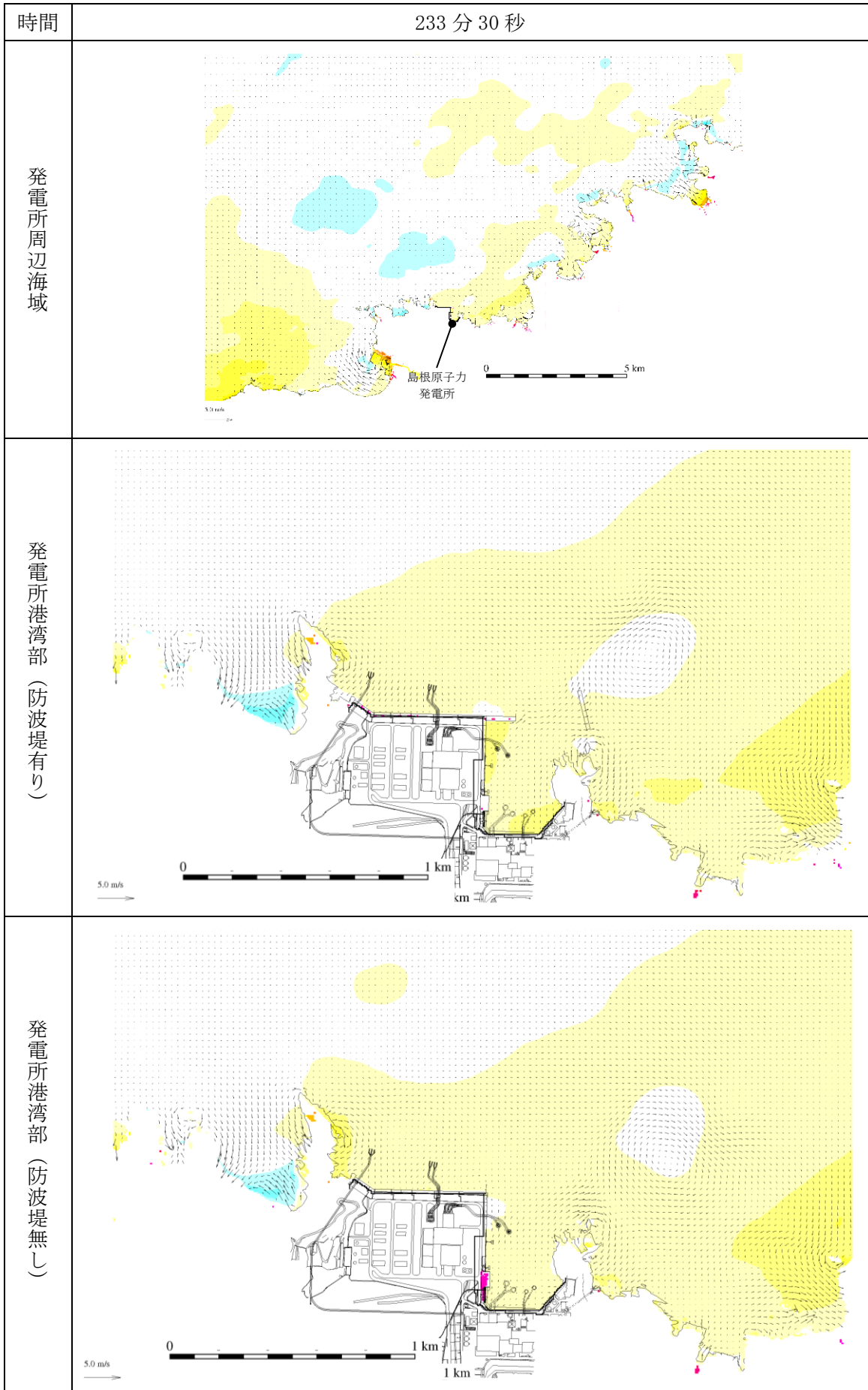
図 1-268 基準津波 1 の水位変動・流向ベクトル
