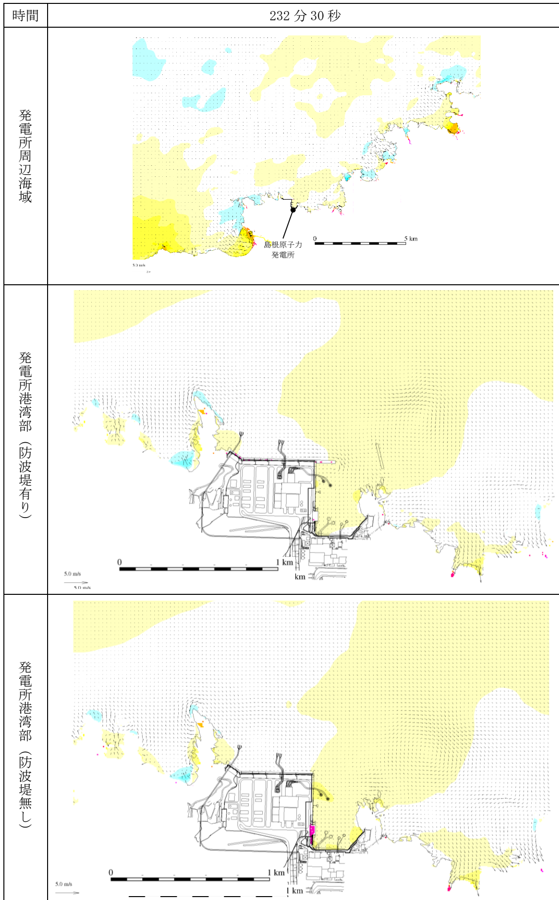
図 1-266 基準津波 1 の水位変動・流向ベクトル
