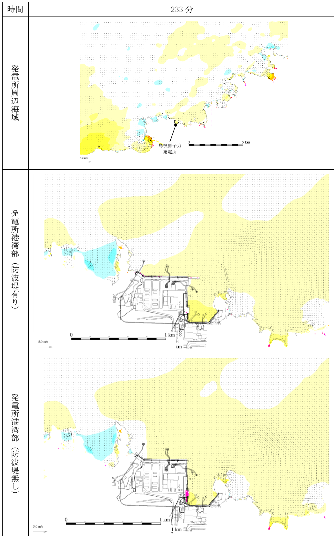
図 1-267 基準津波 1 の水位変動・流向ベクトル
