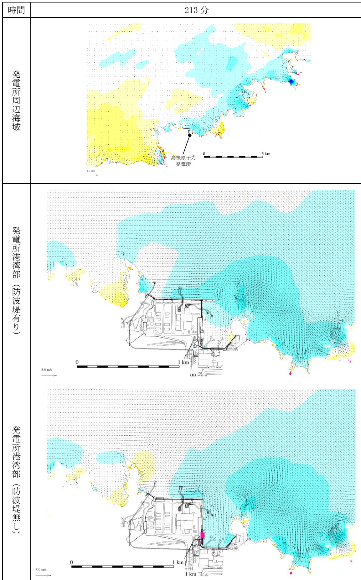
図 1-227 基準津波 1 の水位変動・流向ベクトル
