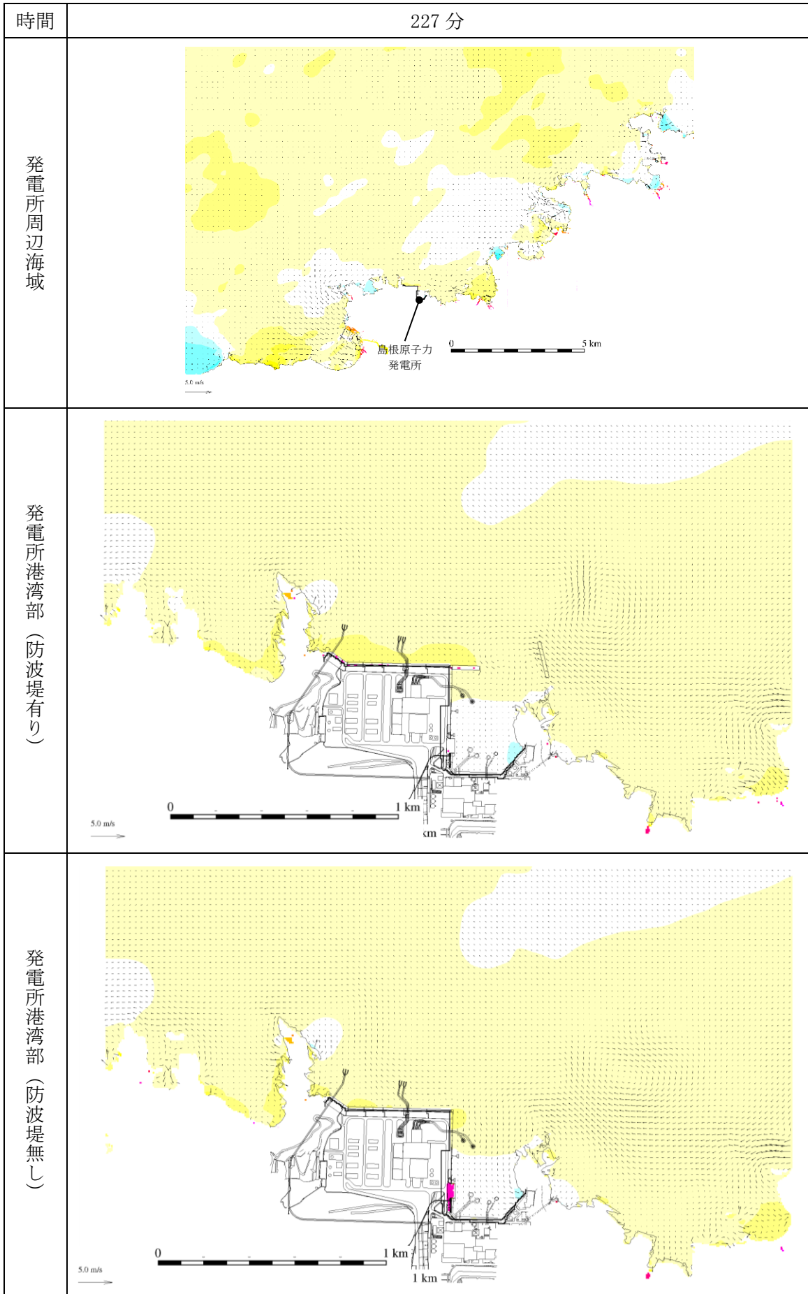
図 1-255 基準津波 1 の水位変動・流向ベクトル
