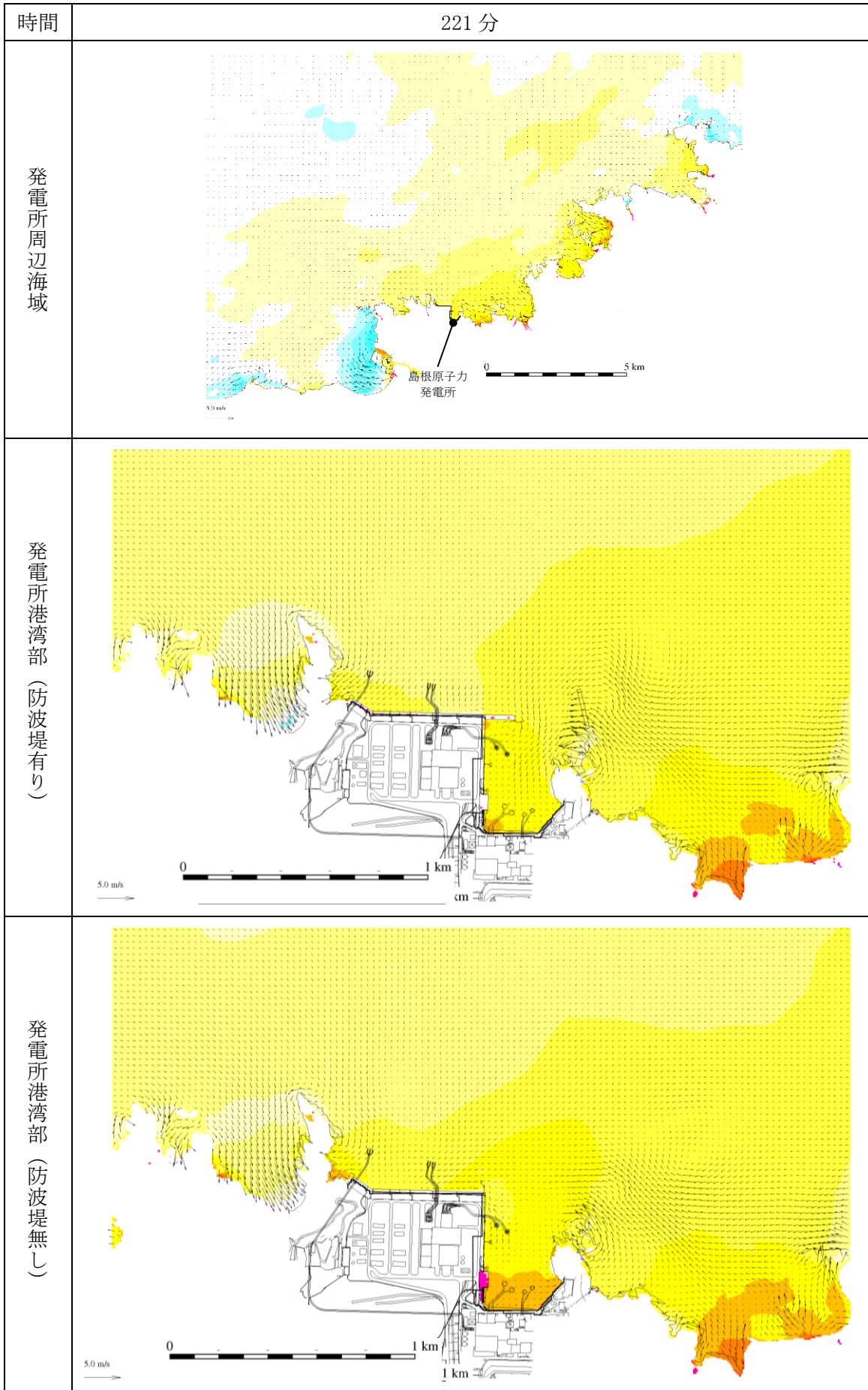
図 1-243 基準津波 1 の水位変動・流向ベクトル
