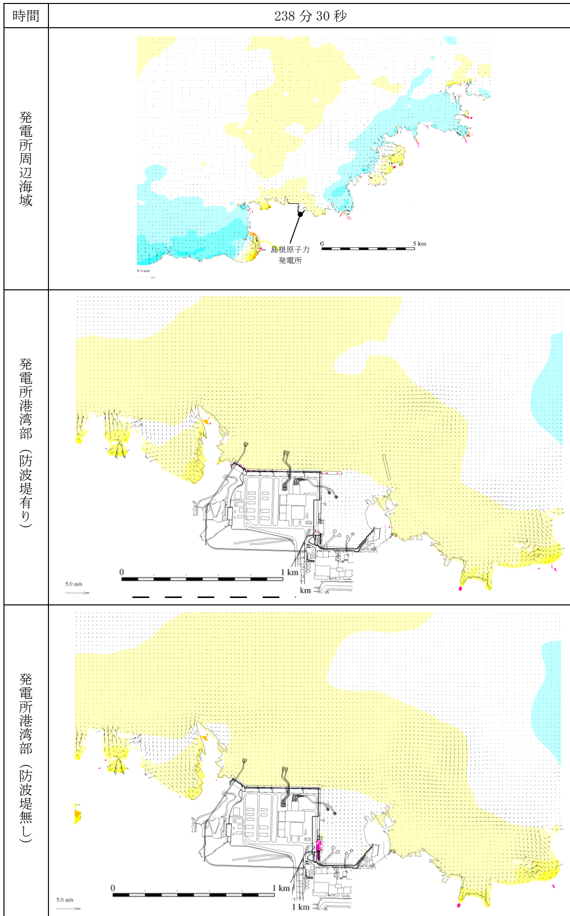
図 1-278 基準津波 1 の水位変動・流向ベクトル
