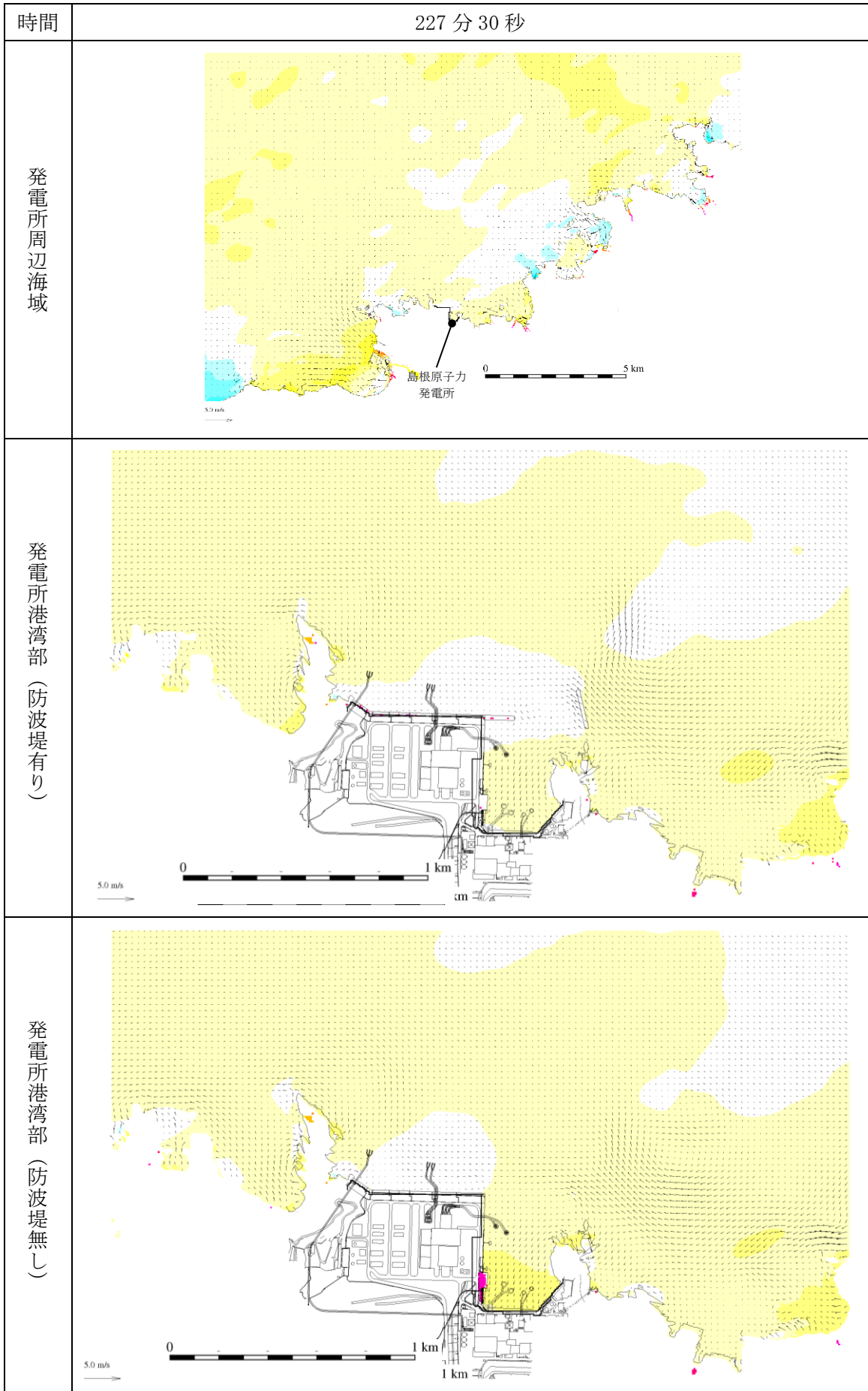
図 1-256 基準津波 1 の水位変動・流向ベクトル
