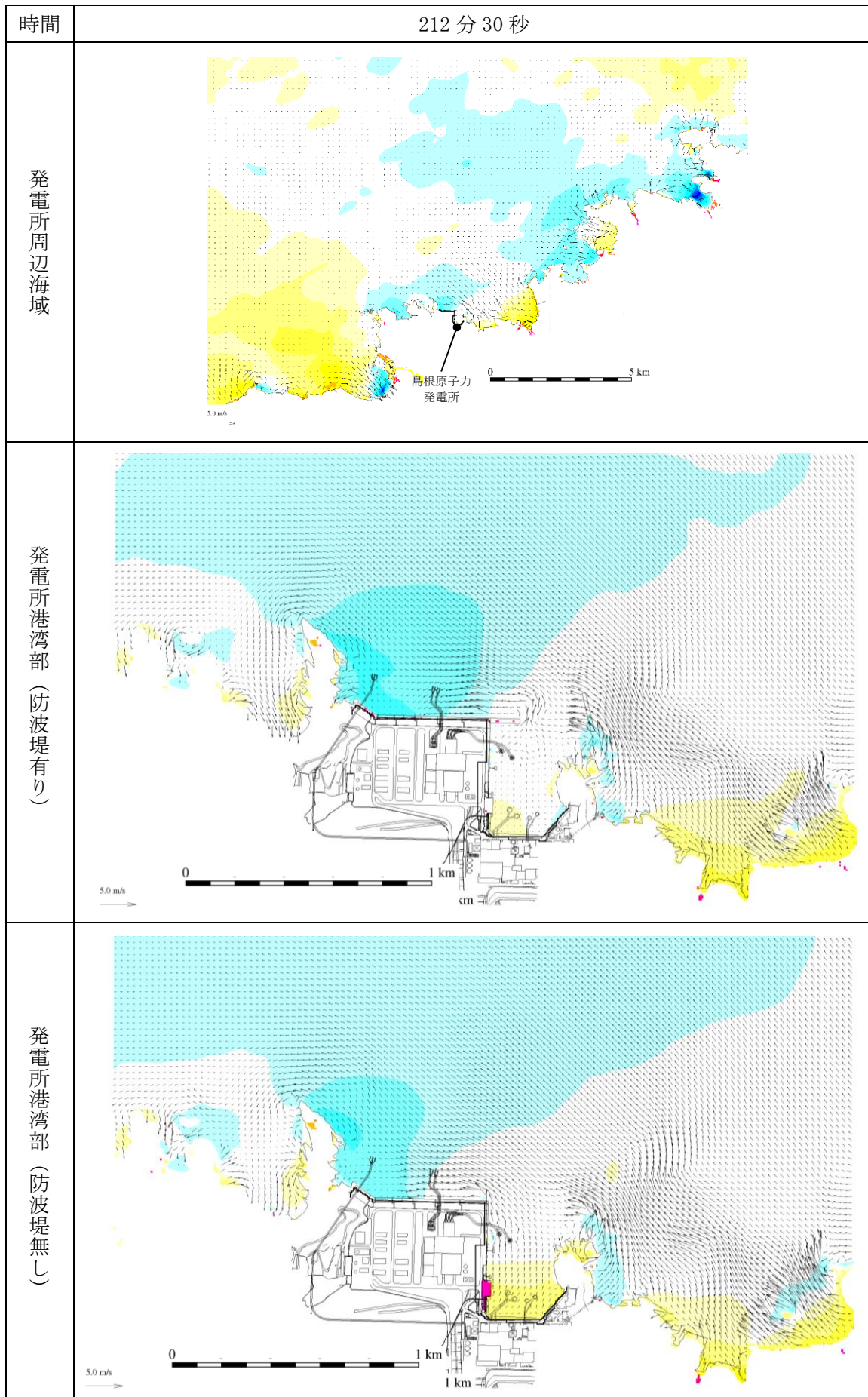
図 1-226 基準津波 1 の水位変動・流向ベクトル
