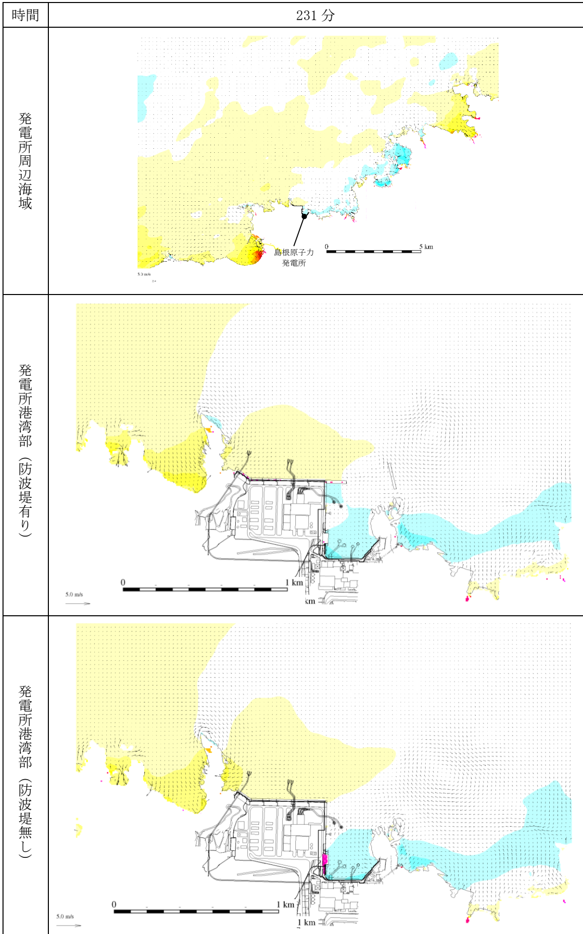
図 1-263 基準津波 1 の水位変動・流向ベクトル
