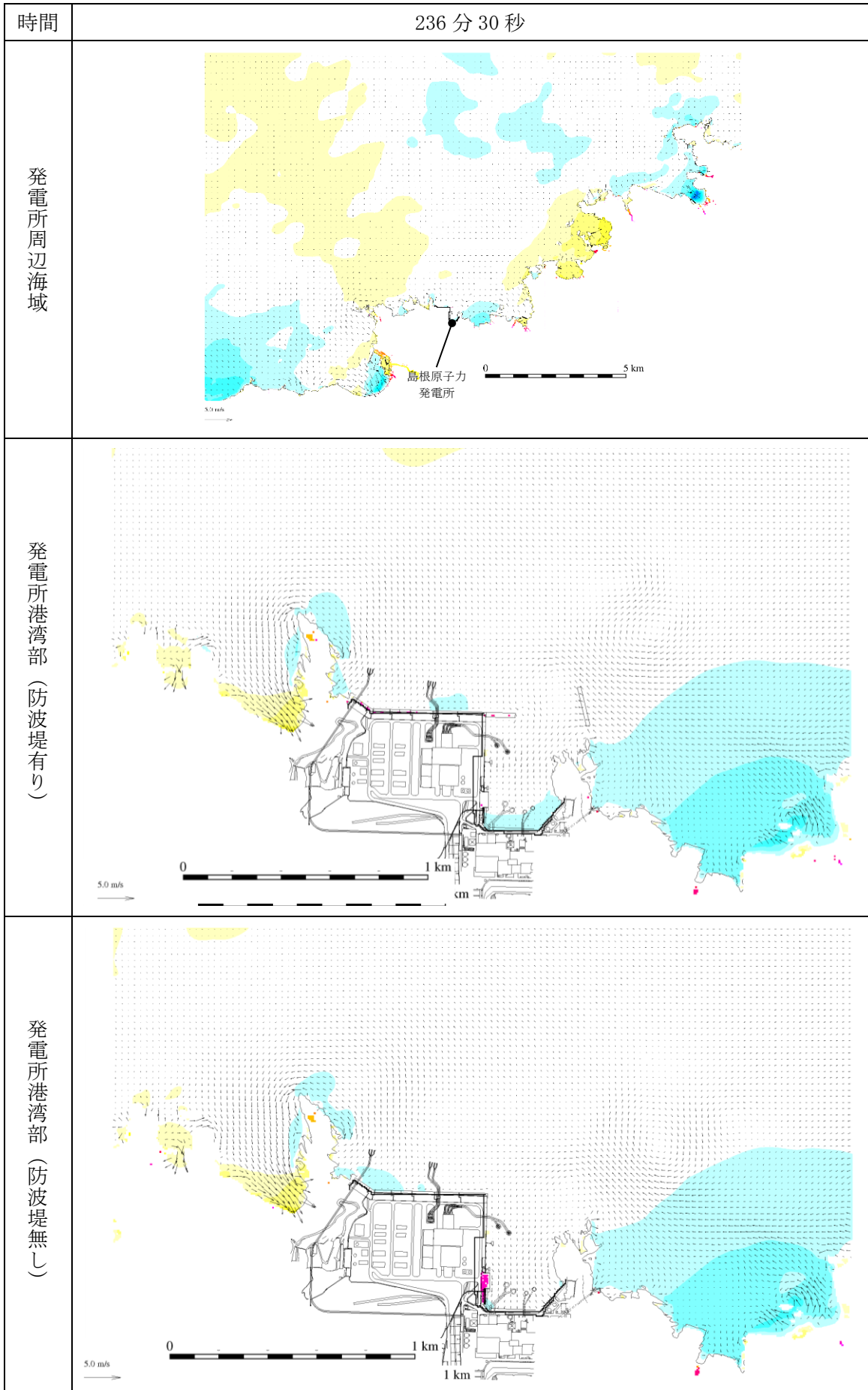
図 1-274 基準津波 1 の水位変動・流向ベクトル
