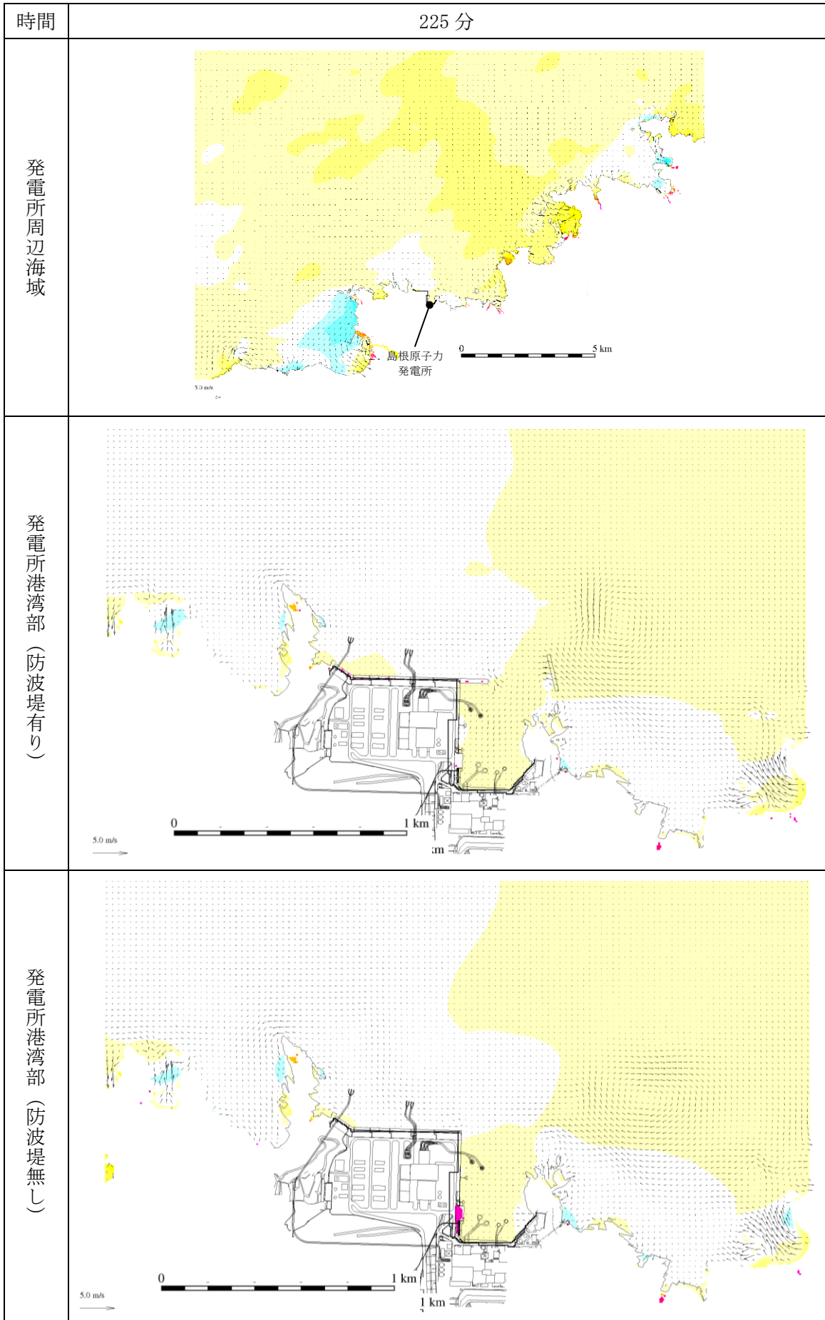
図 1-251 基準津波 1 の水位変動・流向ベクトル
