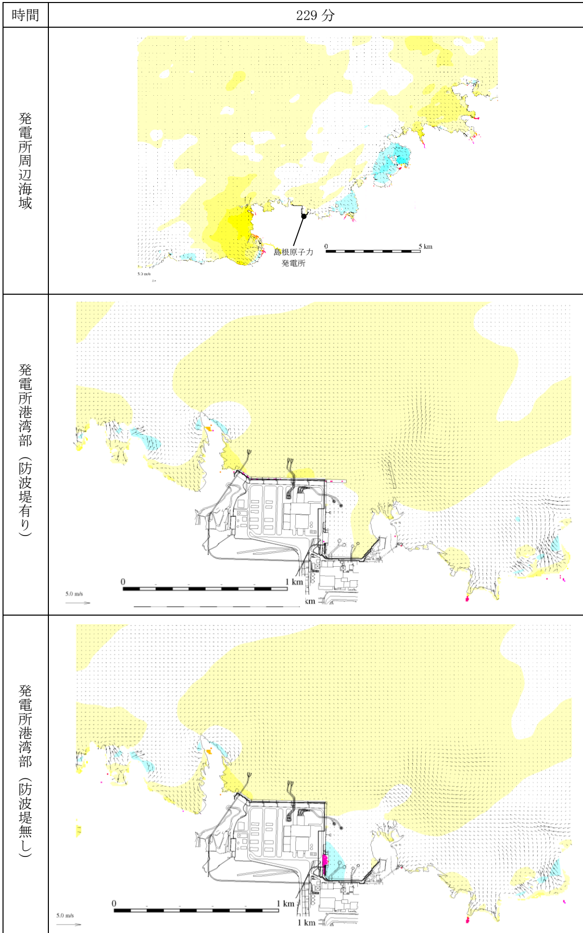
図 1-259 基準津波 1 の水位変動・流向ベクトル
