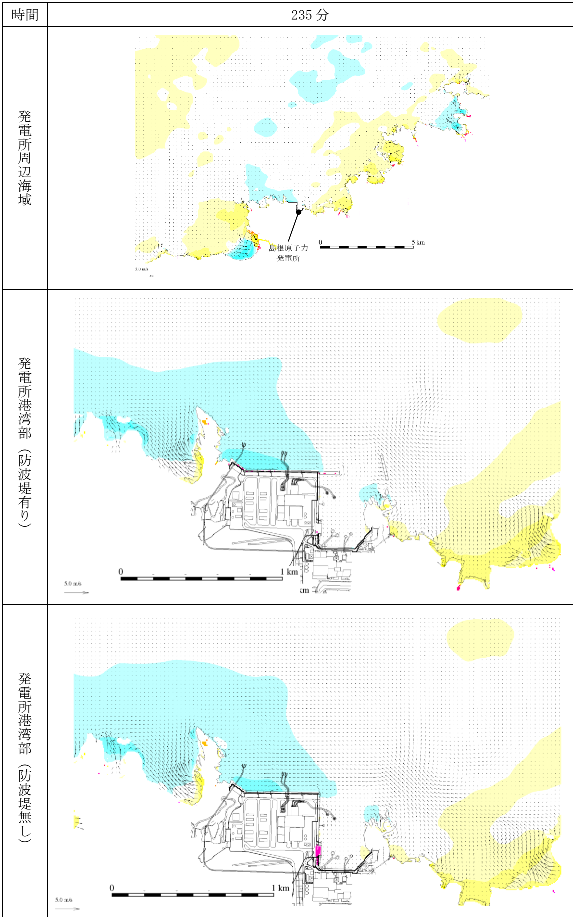
図 1-271 基準津波 1 の水位変動・流向ベクトル
