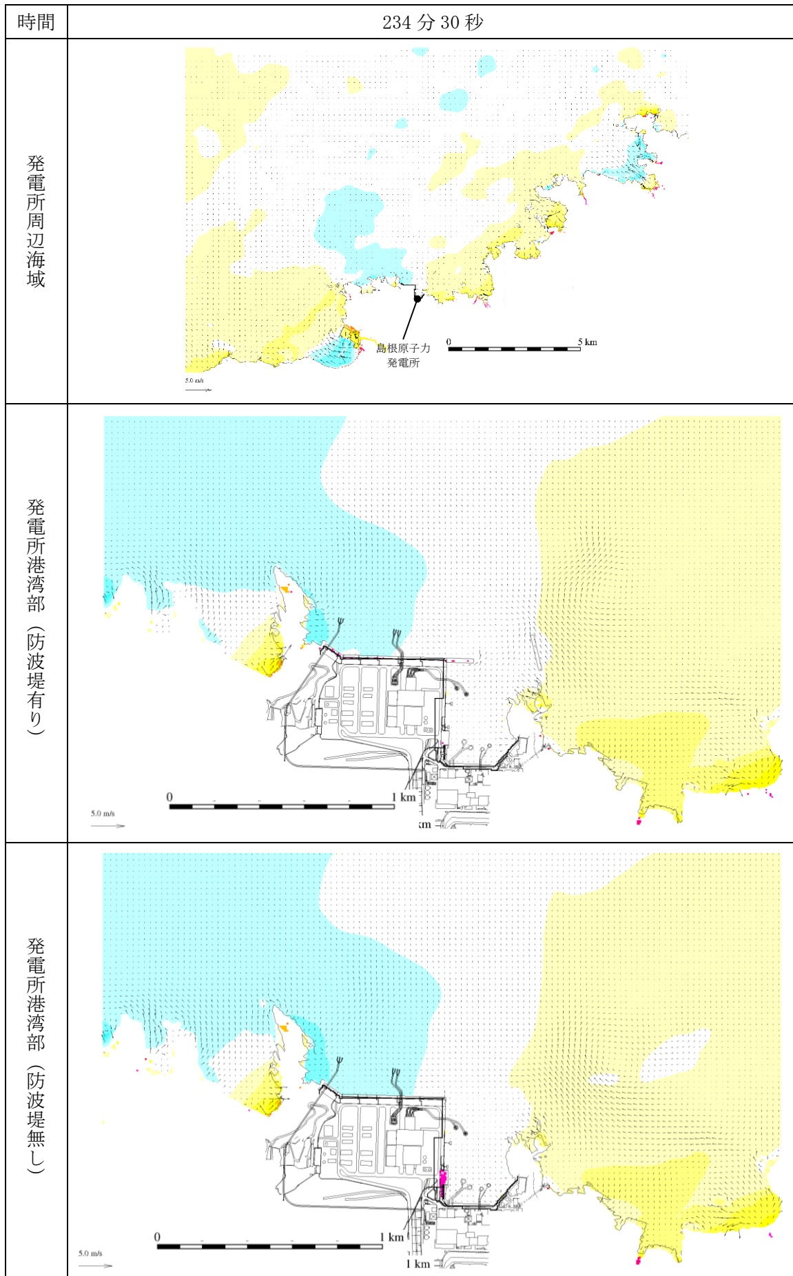
図 1-270 基準津波 1 の水位変動・流向ベクトル
