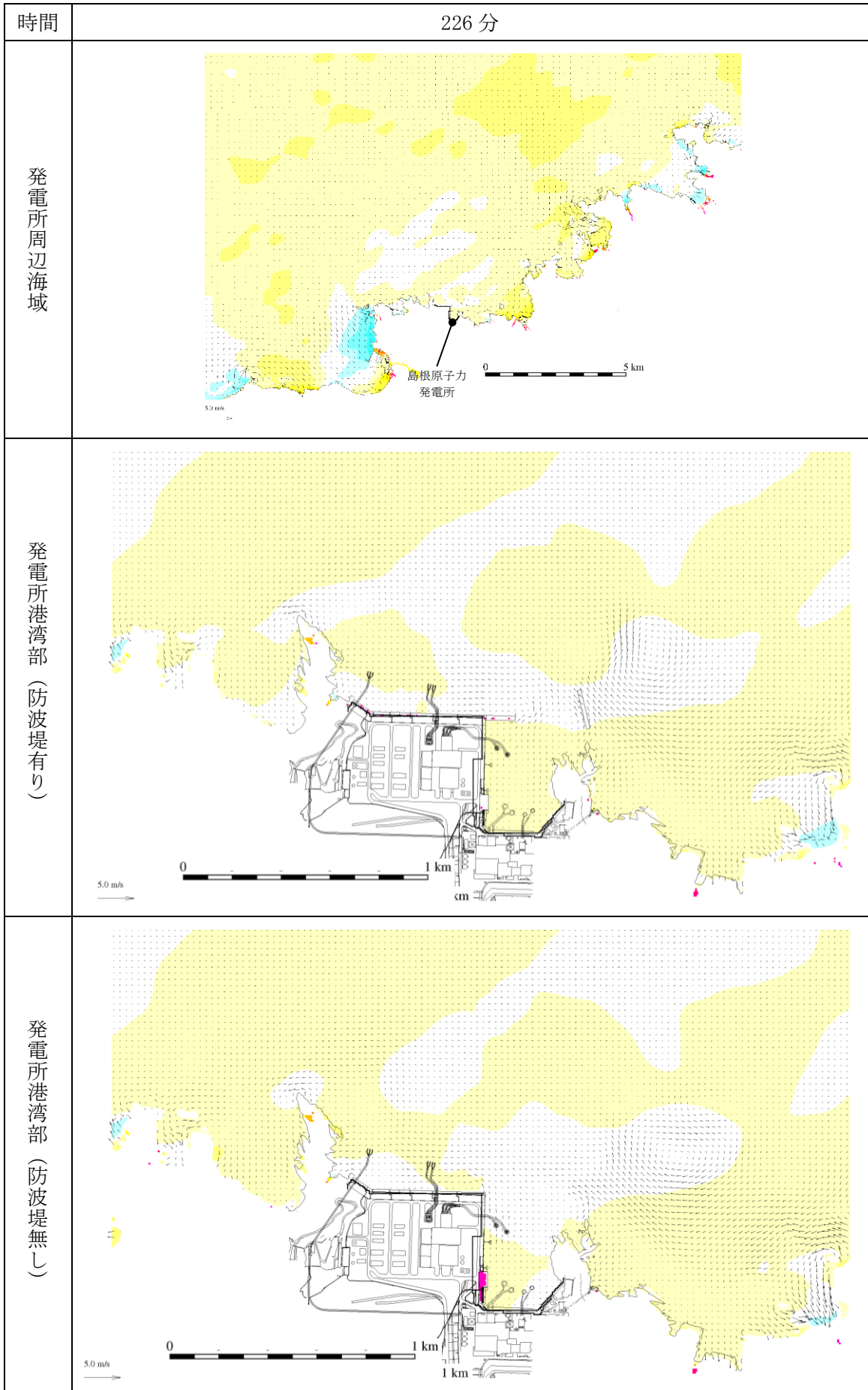
図 1-253 基準津波 1 の水位変動・流向ベクトル
