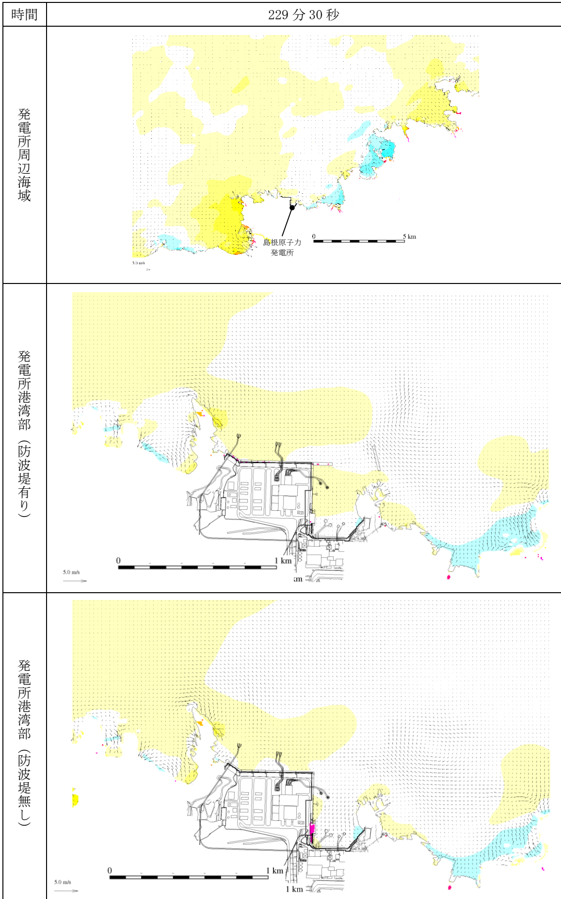
図 1-260 基準津波 1 の水位変動・流向ベクトル
