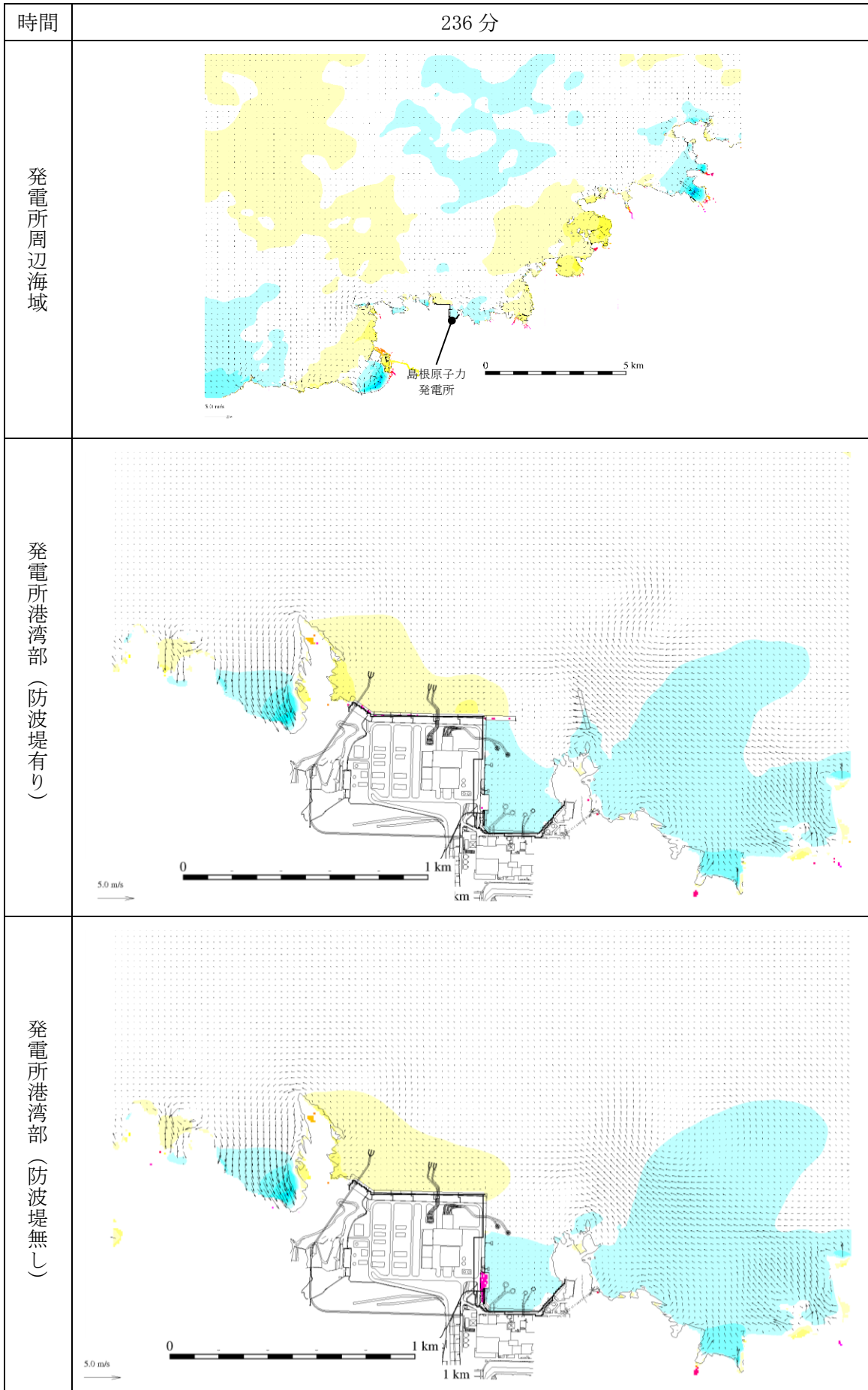
図 1-273 基準津波 1 の水位変動・流向ベクトル
