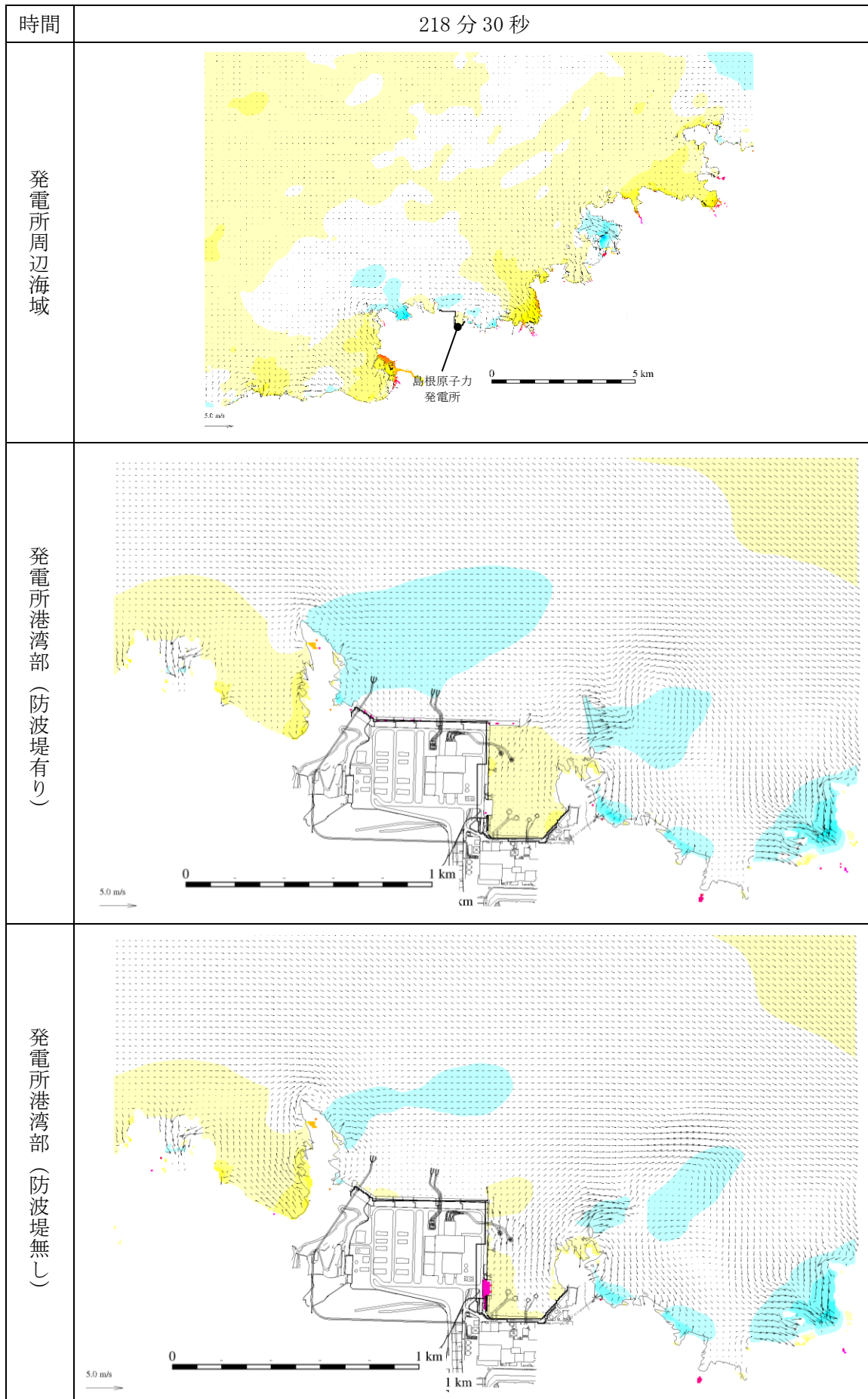
図 1-238 基準津波 1 の水位変動・流向ベクトル
