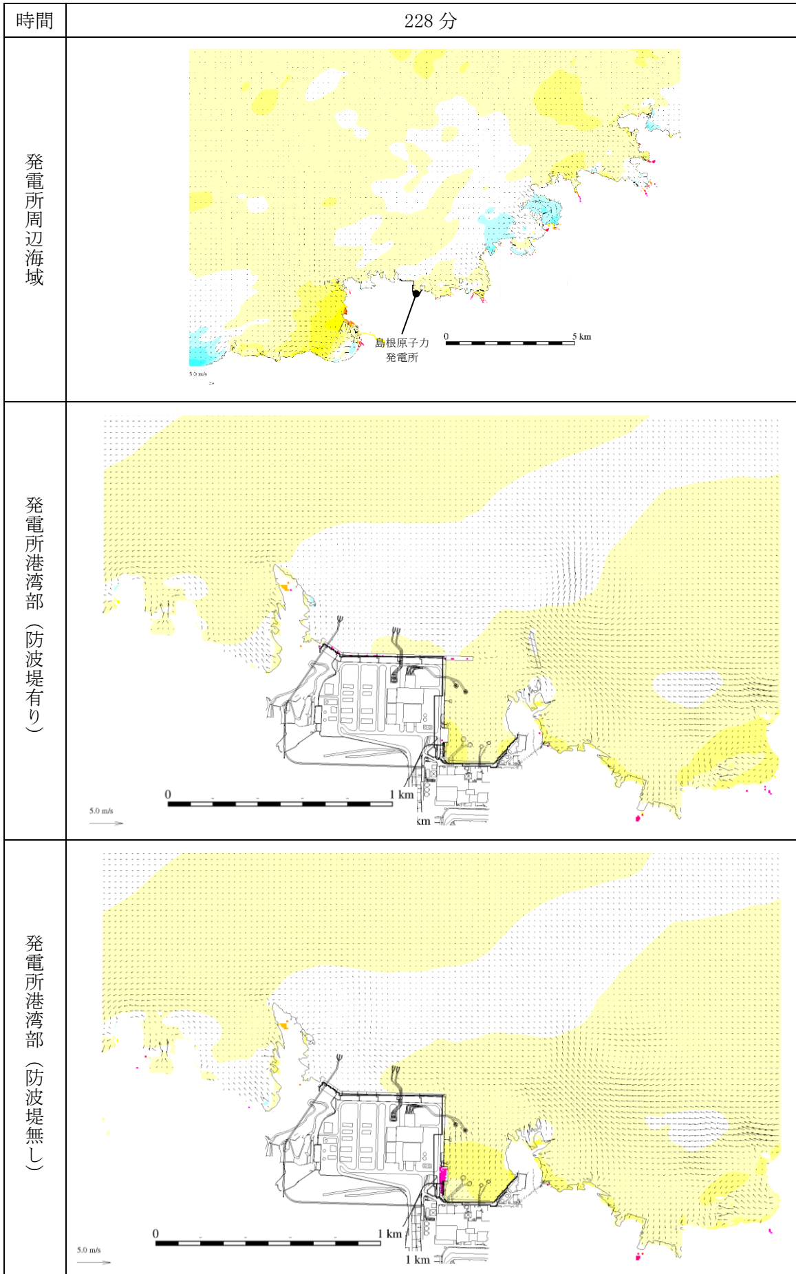
図 1-257 基準津波 1 の水位変動・流向ベクトル
