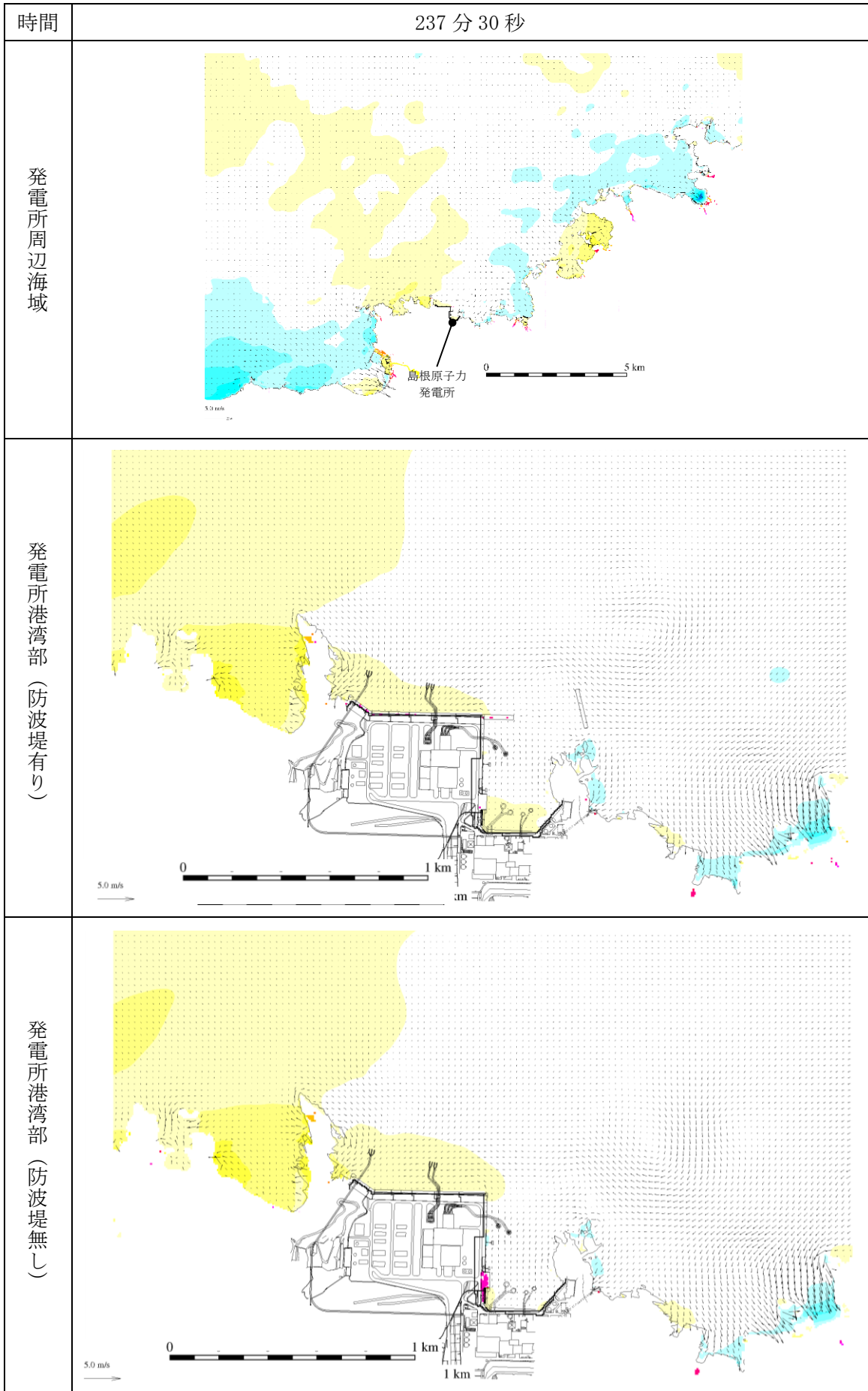
図 1-276 基準津波 1 の水位変動・流向ベクトル
