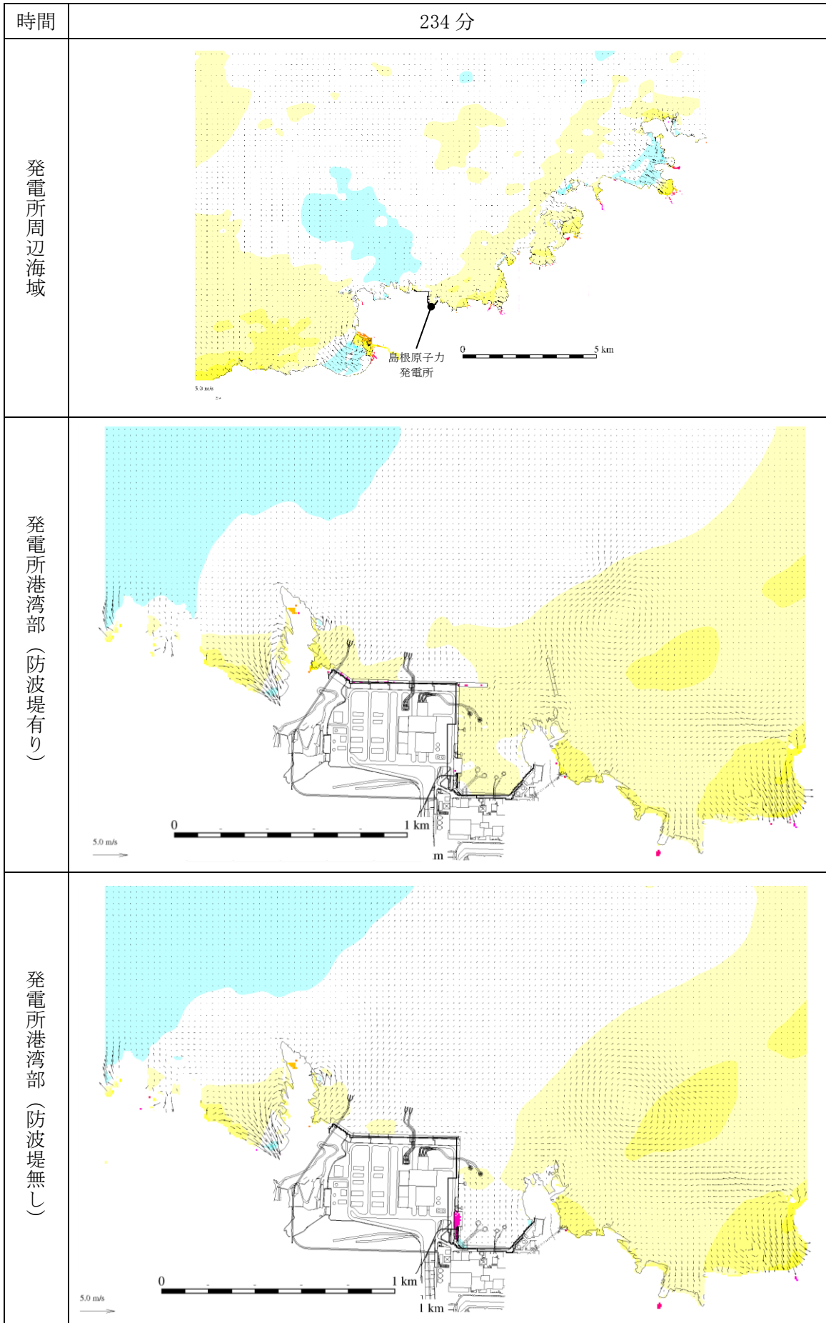
図 1-269 基準津波 1 の水位変動・流向ベクトル
