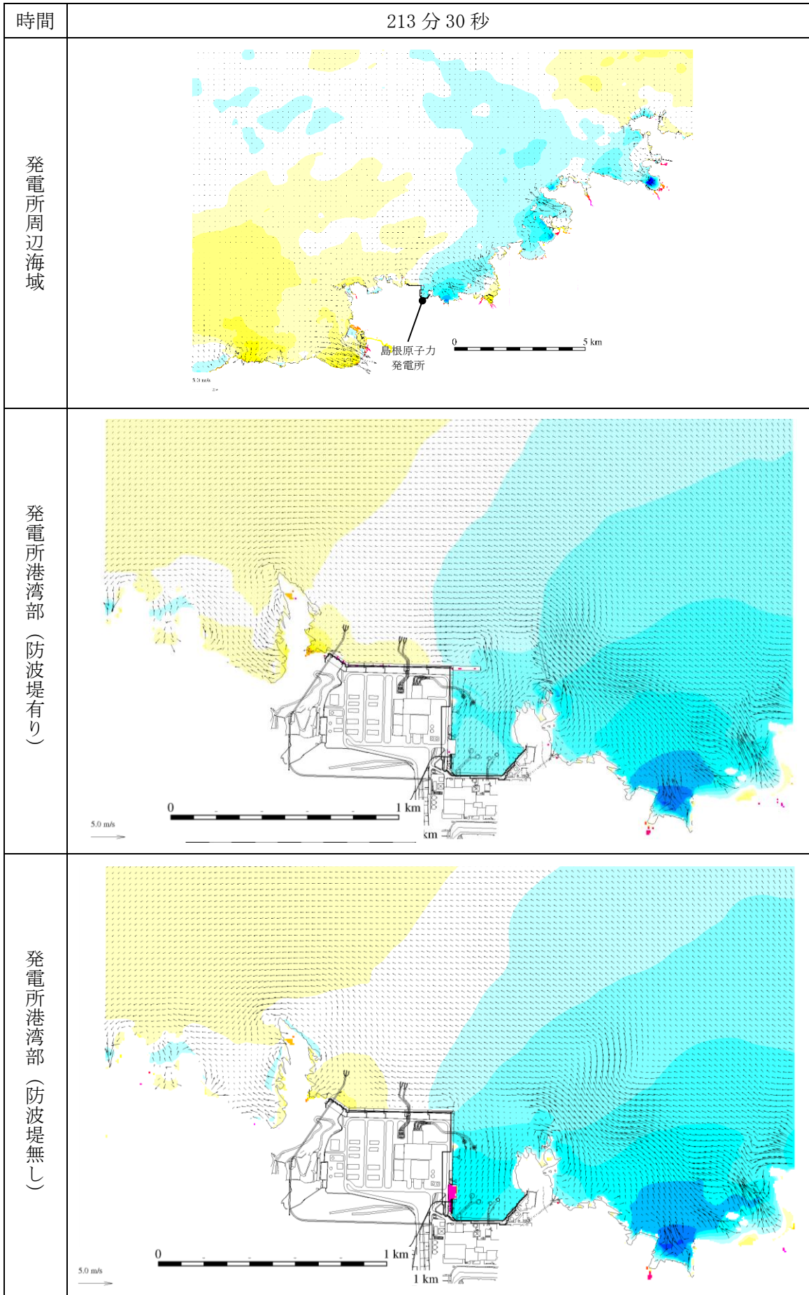
図 1-228 基準津波 1 の水位変動・流向ベクトル
