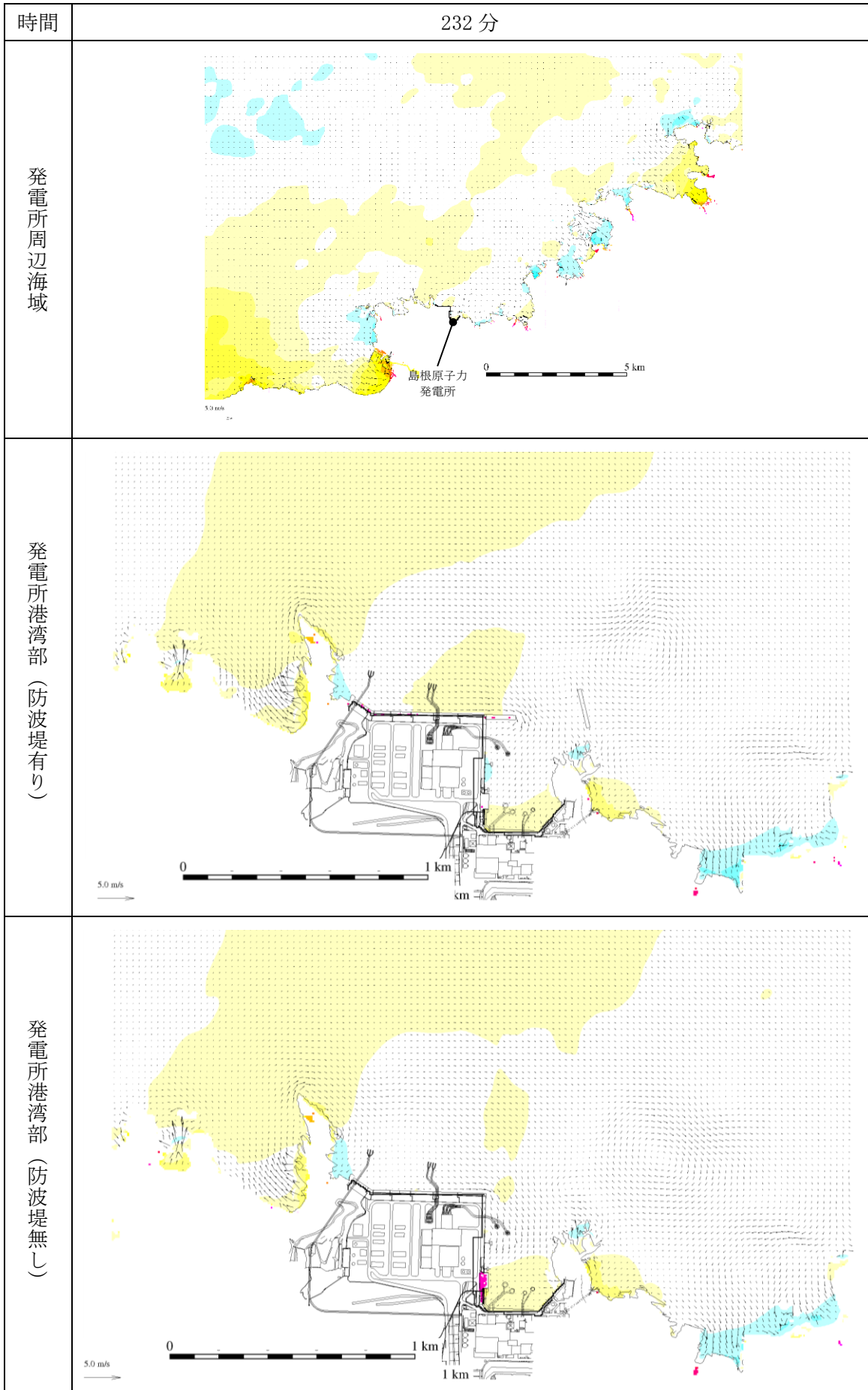
図 1-265 基準津波 1 の水位変動・流向ベクトル
