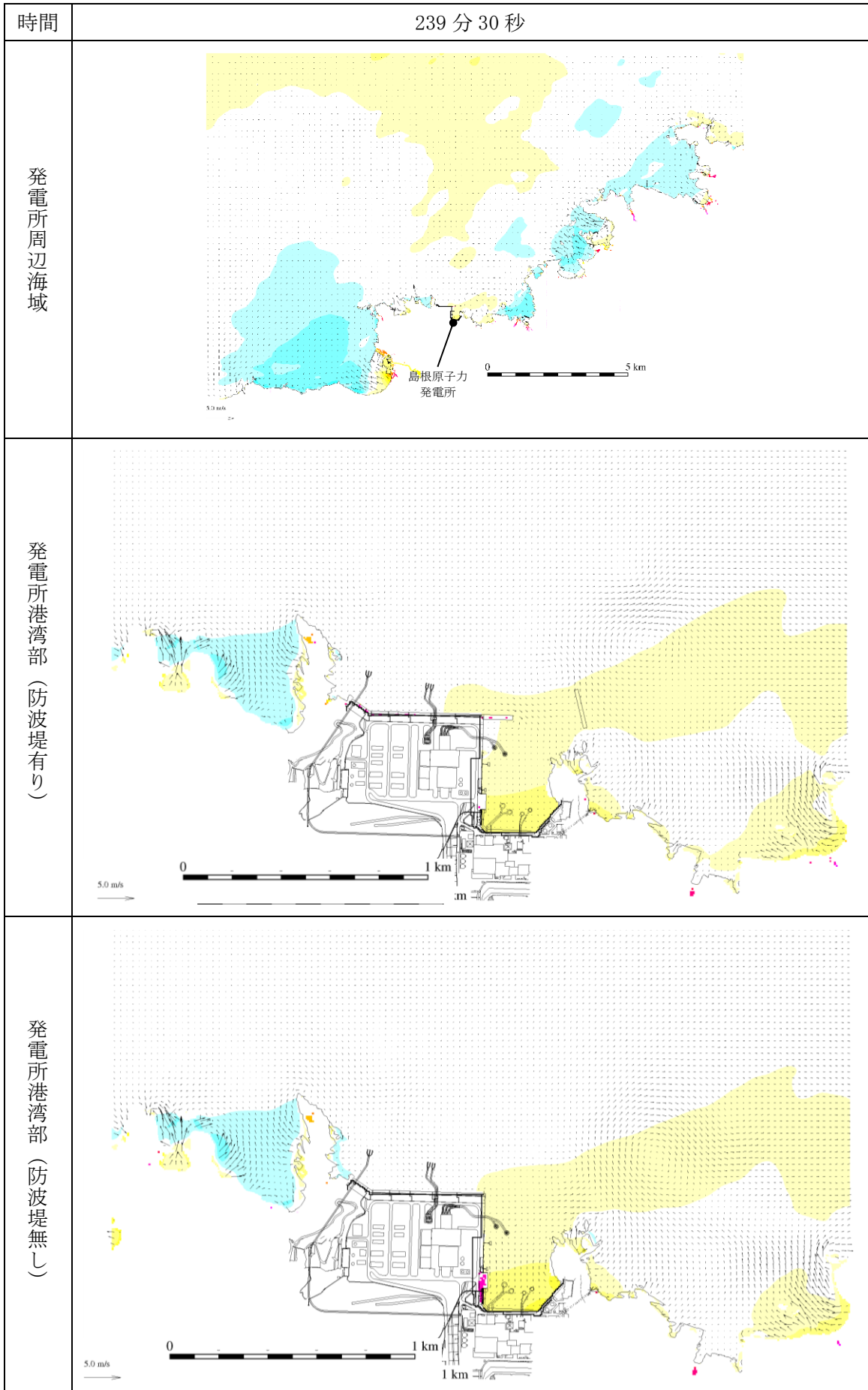
図 1-280 基準津波 1 の水位変動・流向ベクトル
