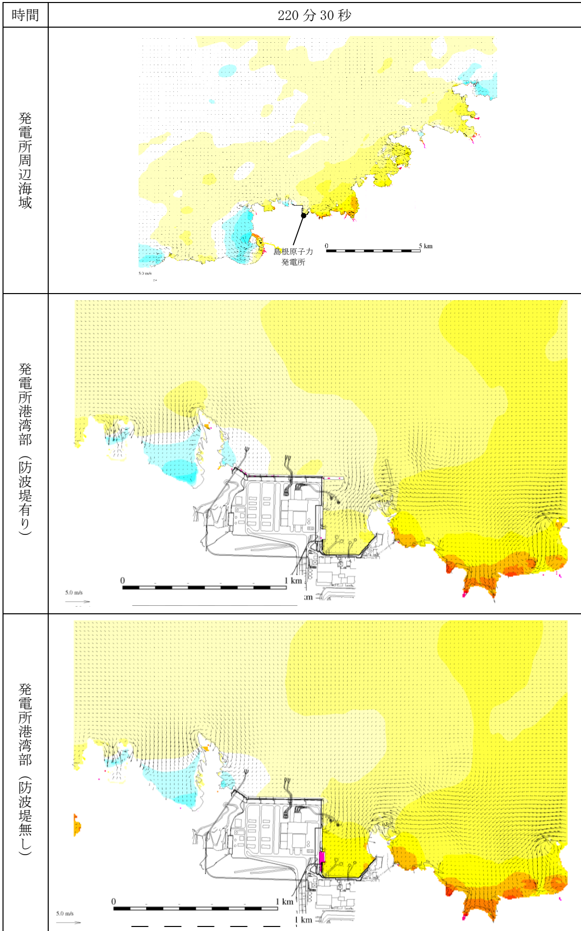
図 1-242 基準津波 1 の水位変動・流向ベクトル
