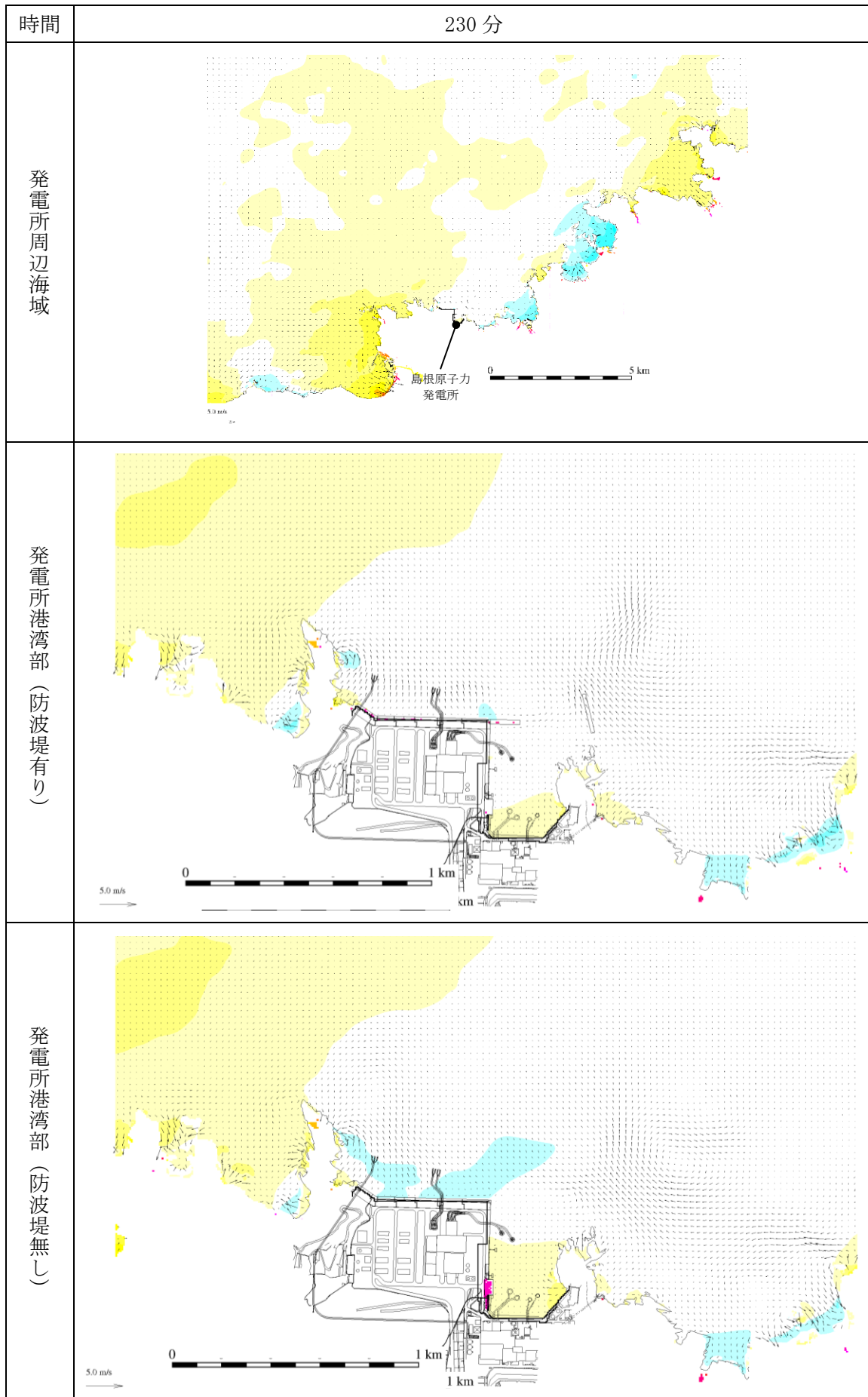
図 1-261 基準津波 1 の水位変動・流向ベクトル
