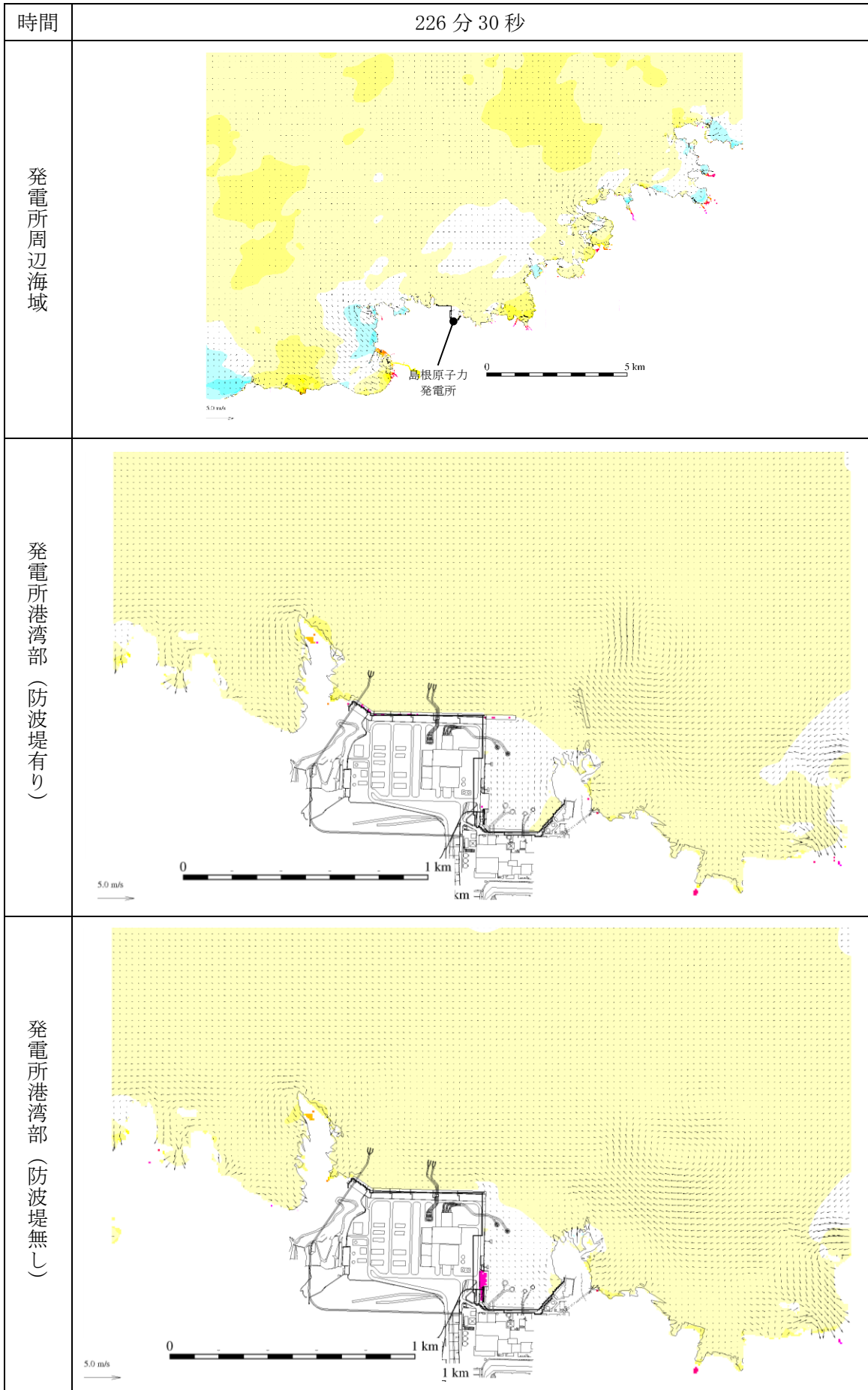
図 1-254 基準津波 1 の水位変動・流向ベクトル
