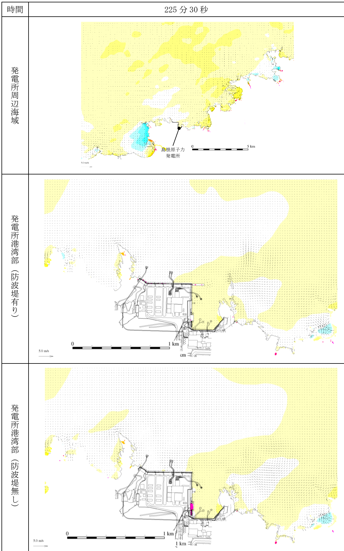
図 1-252 基準津波 1 の水位変動・流向ベクトル
