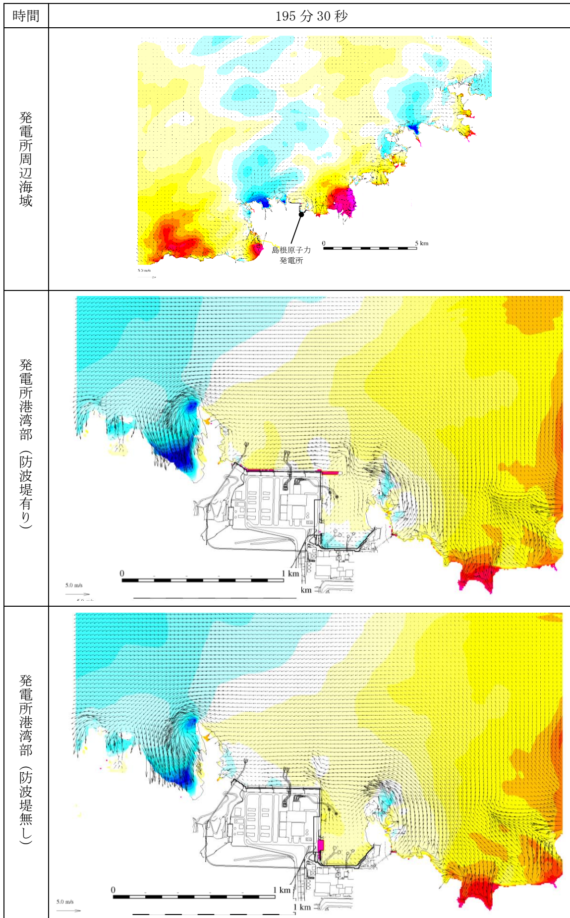
図 1-192 基準津波 1 の水位変動・流向ベクトル
