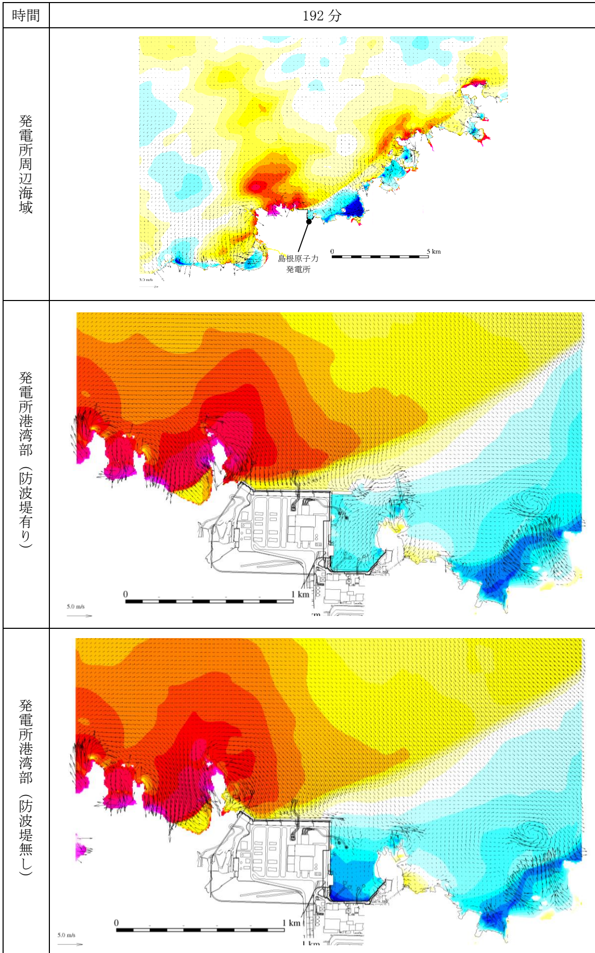
図 1-185 基準津波 1 の水位変動・流向ベクトル
