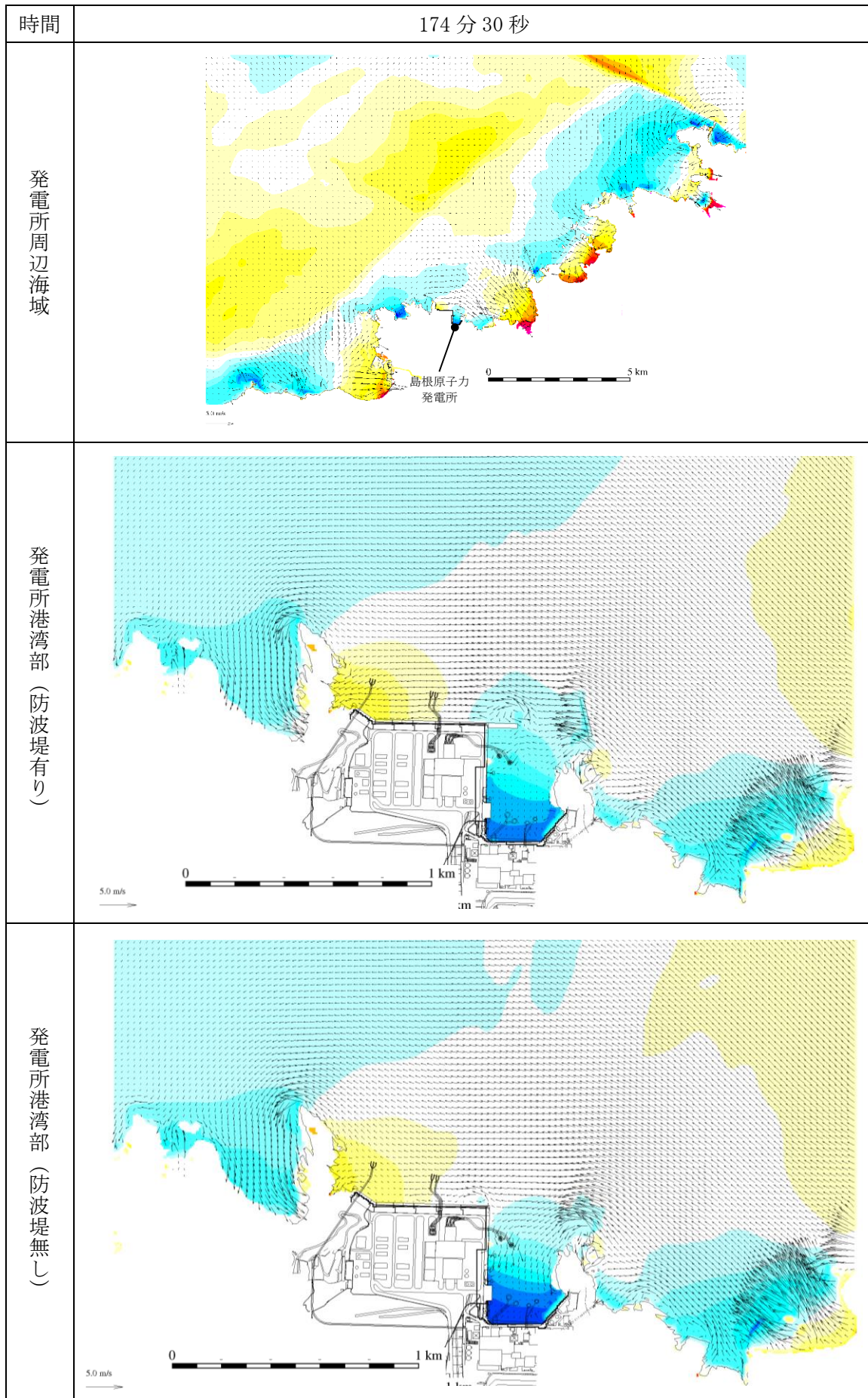
図 1-150 基準津波 1 の水位変動・流向ベクトル
