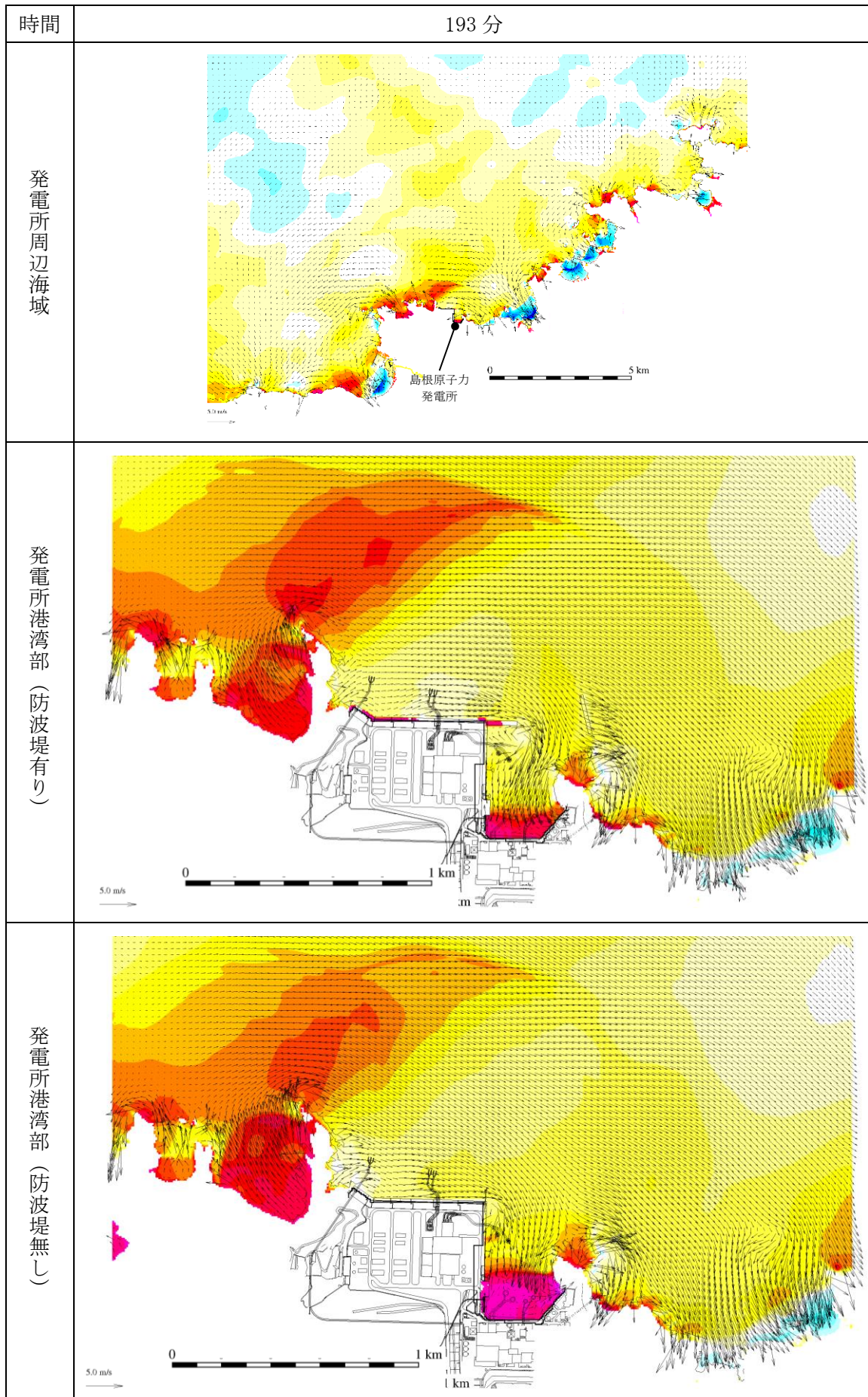
図 1-187 基準津波 1 の水位変動・流向ベクトル
