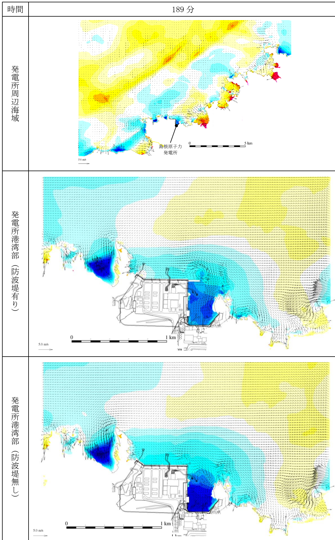
図 1-179 基準津波 1 の水位変動・流向ベクトル
