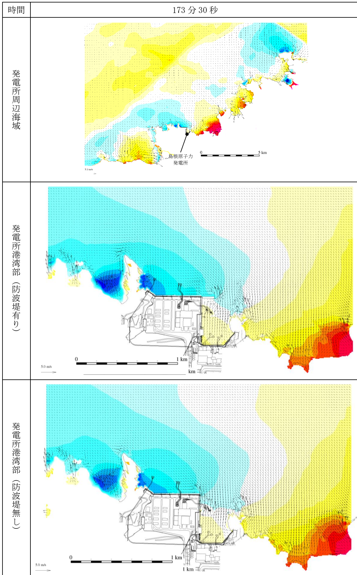
図 1-148 基準津波 1 の水位変動・流向ベクトル
