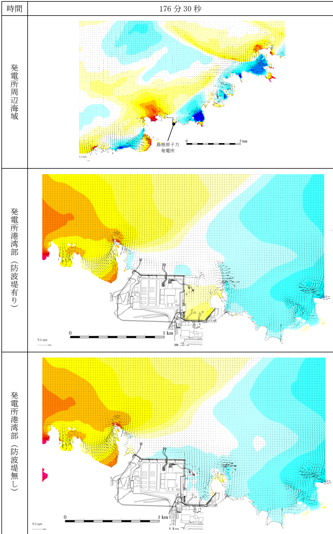
図 1-154 基準津波 1 の水位変動・流向ベクトル
