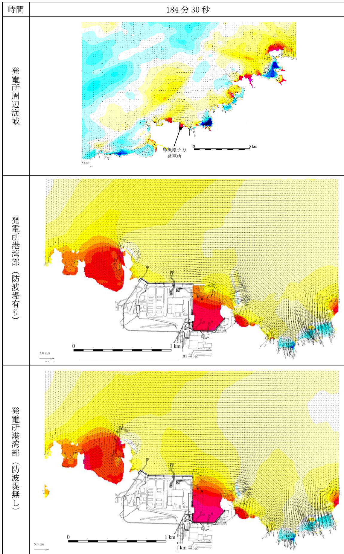
図 1-170 基準津波 1 の水位変動・流向ベクトル
