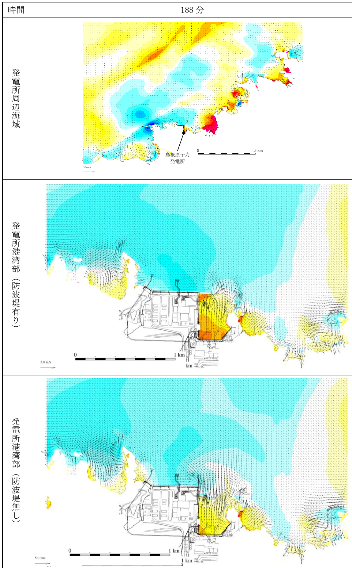
図 1-177 基準津波 1 の水位変動・流向ベクトル
