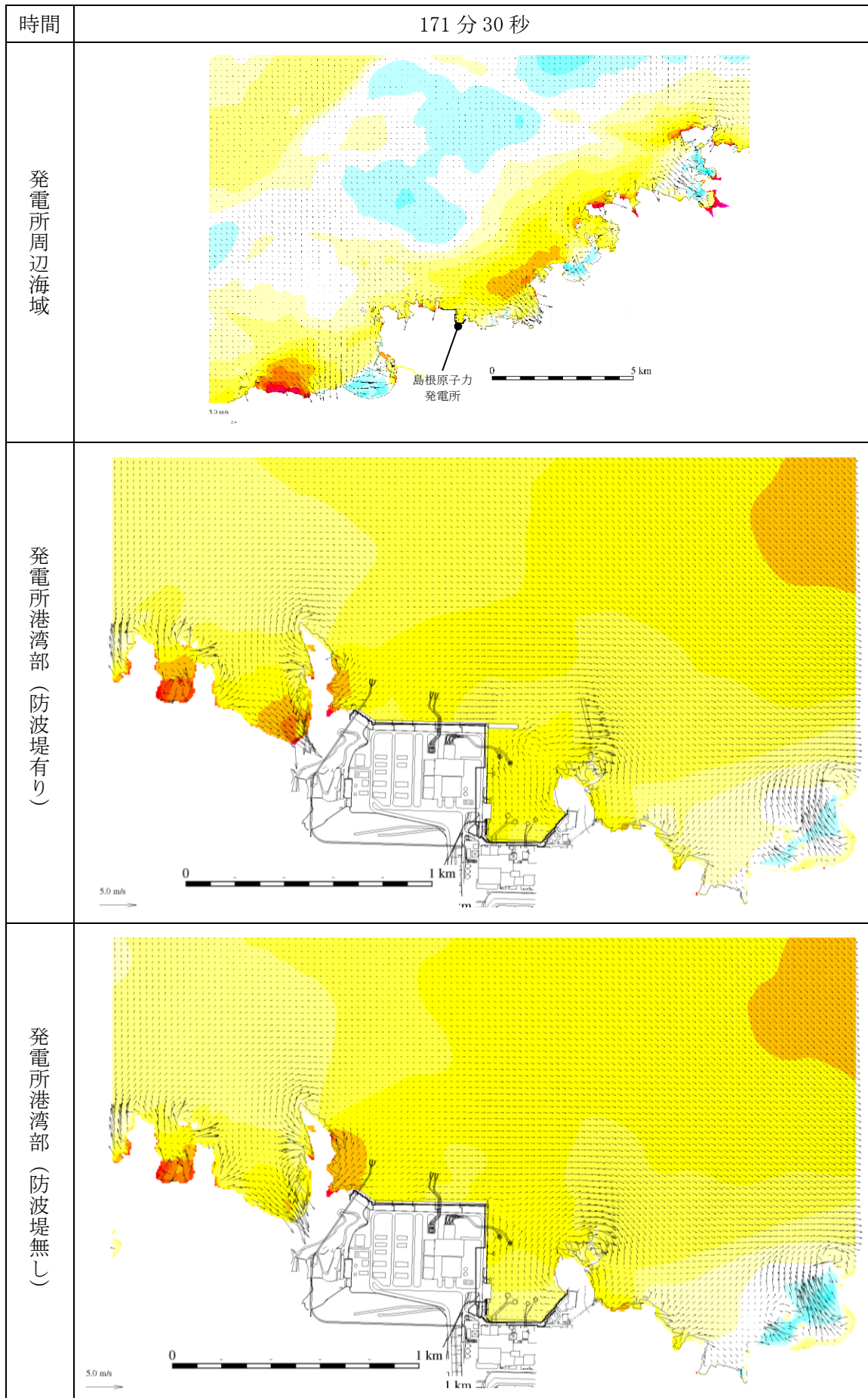
図 1-144 基準津波 1 の水位変動・流向ベクトル
