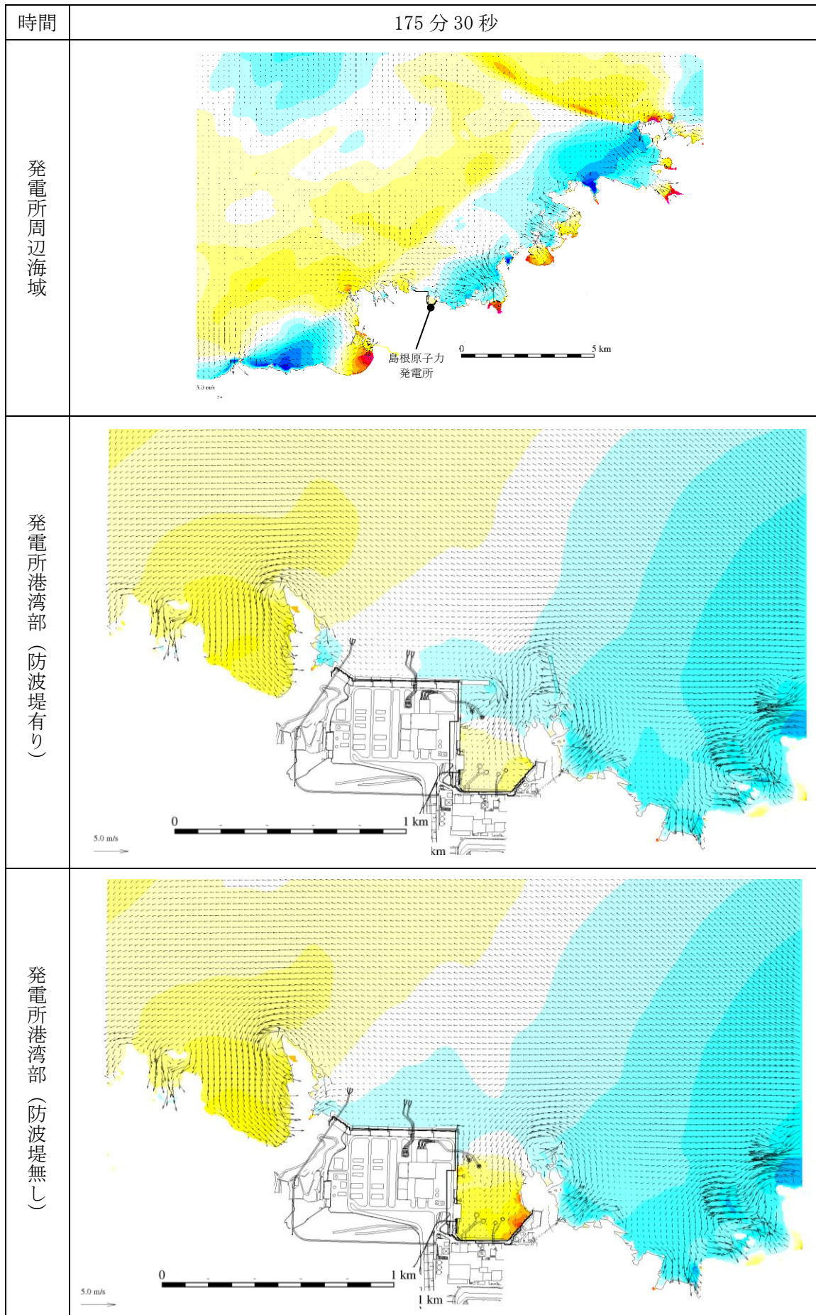
図 1-152 基準津波 1 の水位変動・流向ベクトル
