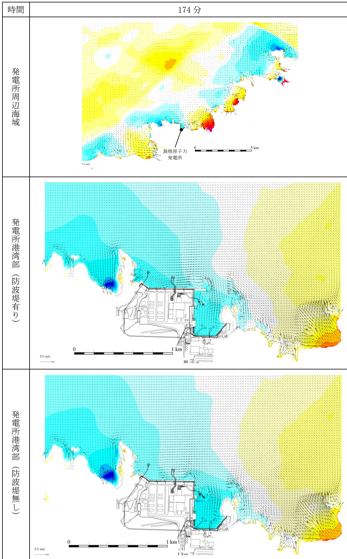
図 1-149 基準津波 1 の水位変動・流向ベクトル
