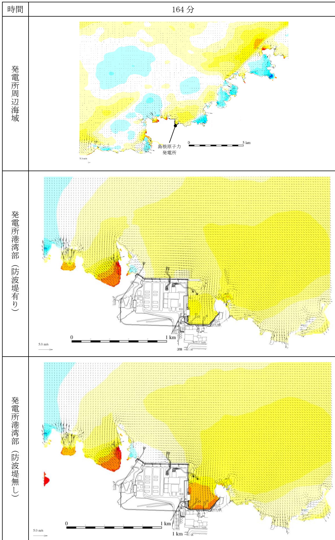
図 1-129 基準津波 1 の水位変動・流向ベクトル
