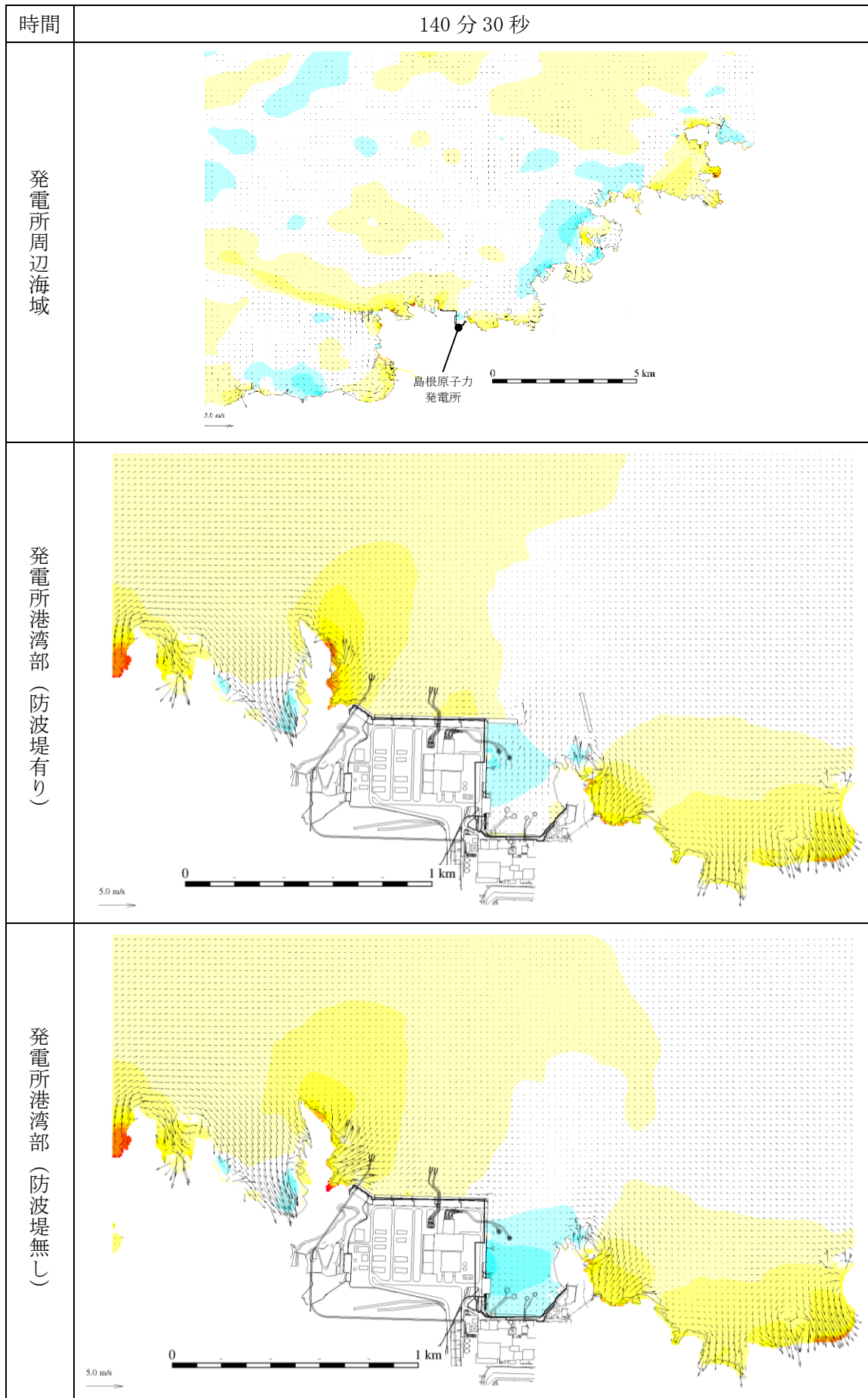
図 1-82 基準津波 1 の水位変動・流向ベクトル
