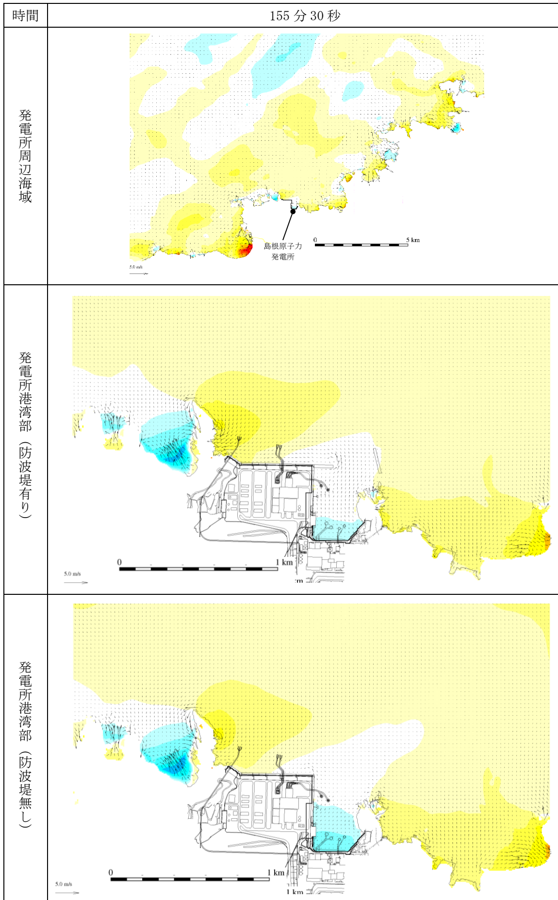
図 1-112 基準津波 1 の水位変動・流向ベクトル
