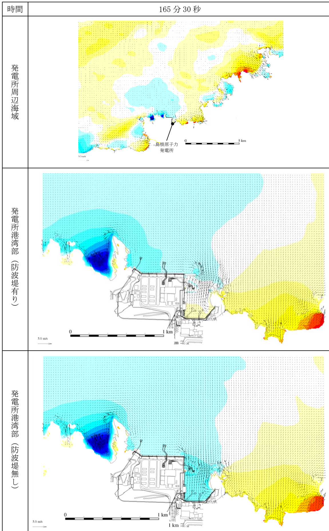
図 1-132 基準津波 1 の水位変動・流向ベクトル
