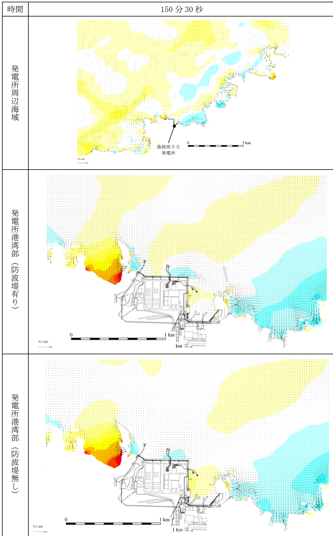
図 1-102 基準津波 1 の水位変動・流向ベクトル
