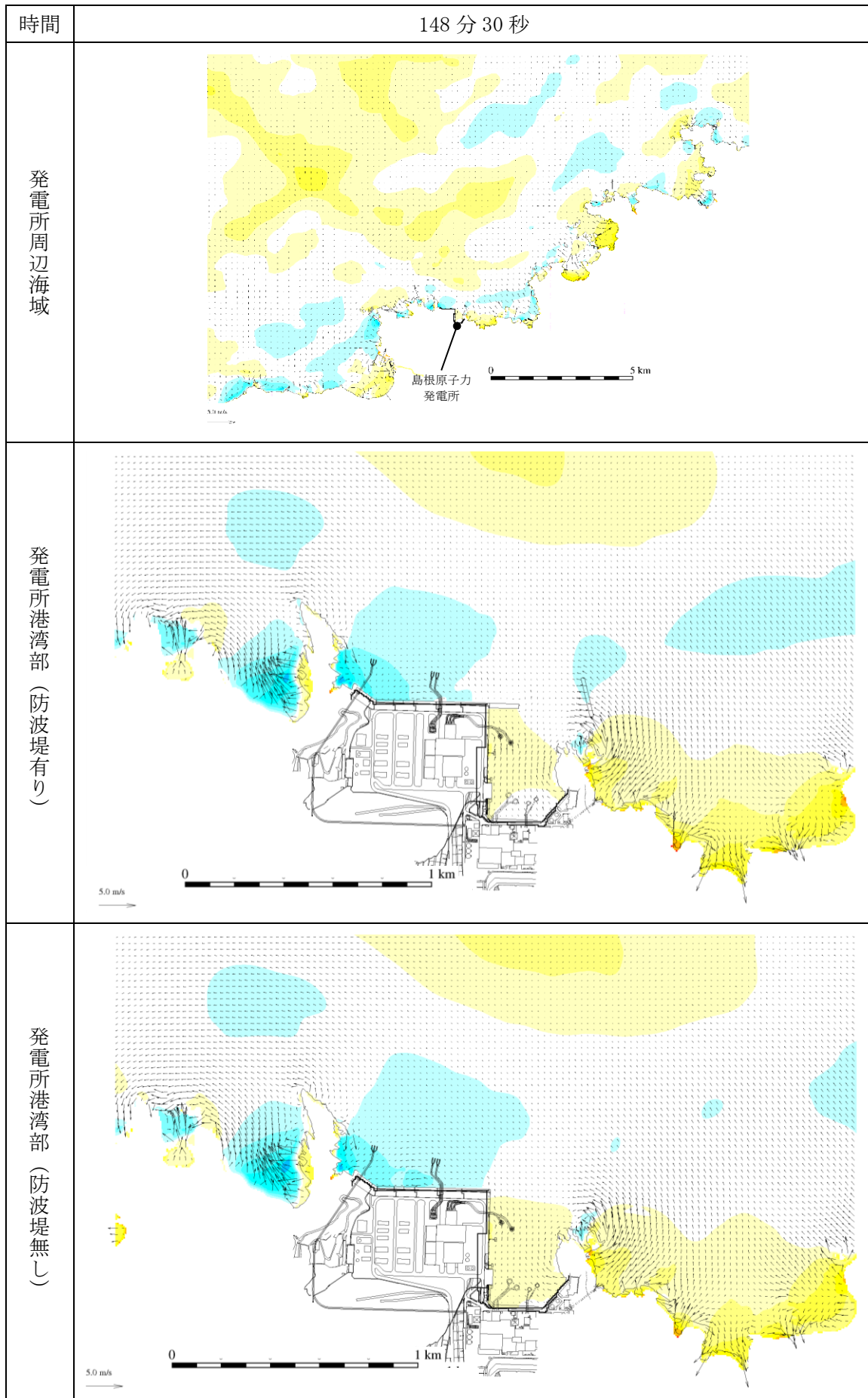
図 1-98 基準津波 1 の水位変動・流向ベクトル
