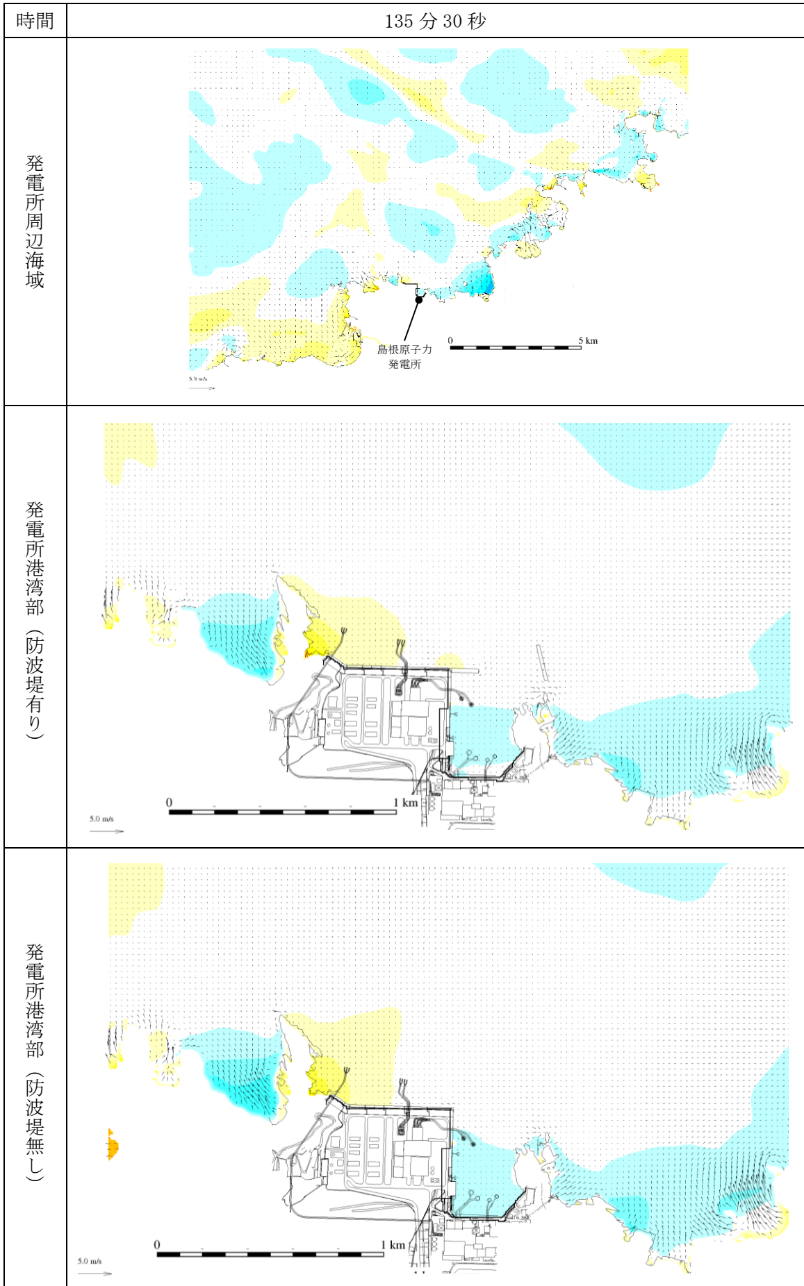
図 1-72 基準津波 1 の水位変動・流向ベクトル
