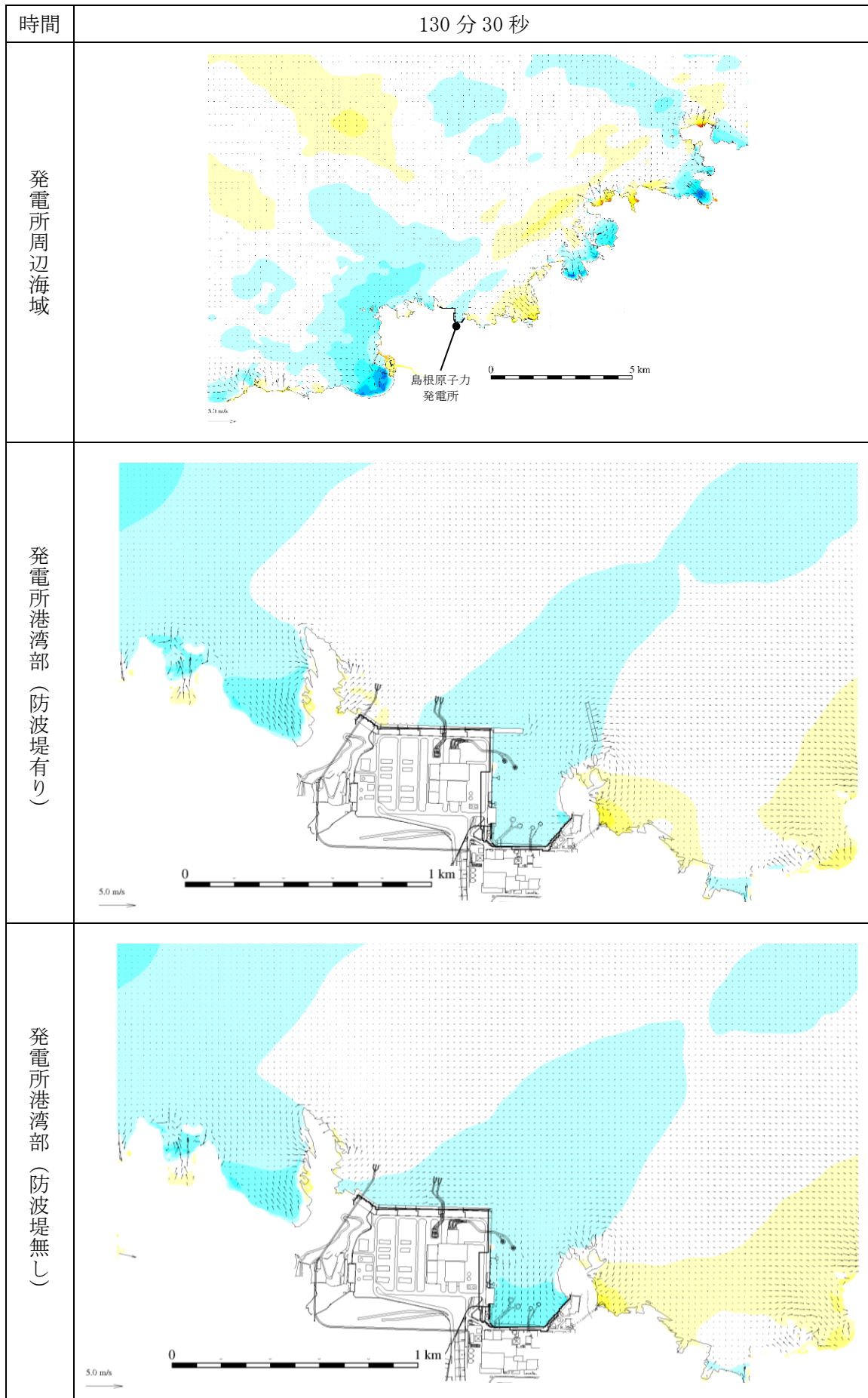
図 1-62 基準津波 1 の水位変動・流向ベクトル
