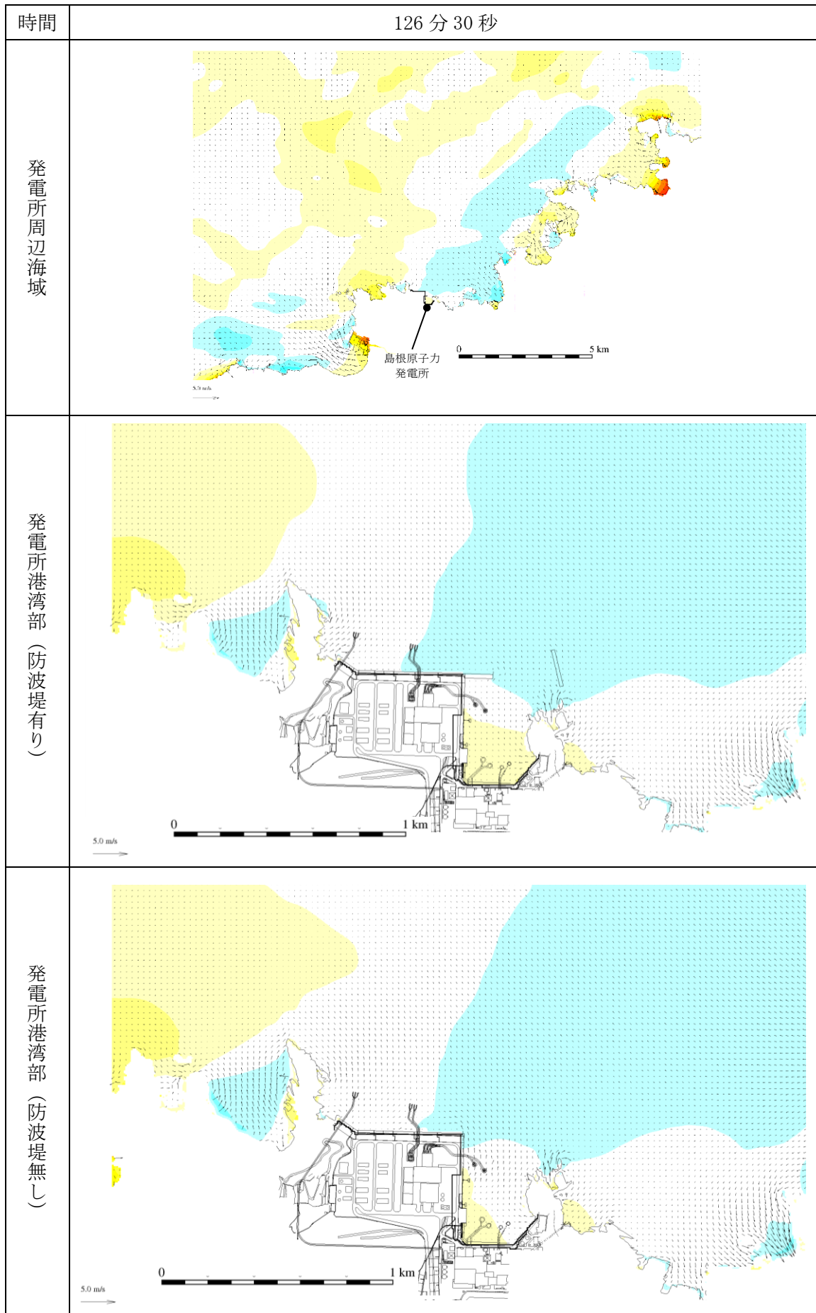
図 1-54 基準津波 1 の水位変動・流向ベクトル
