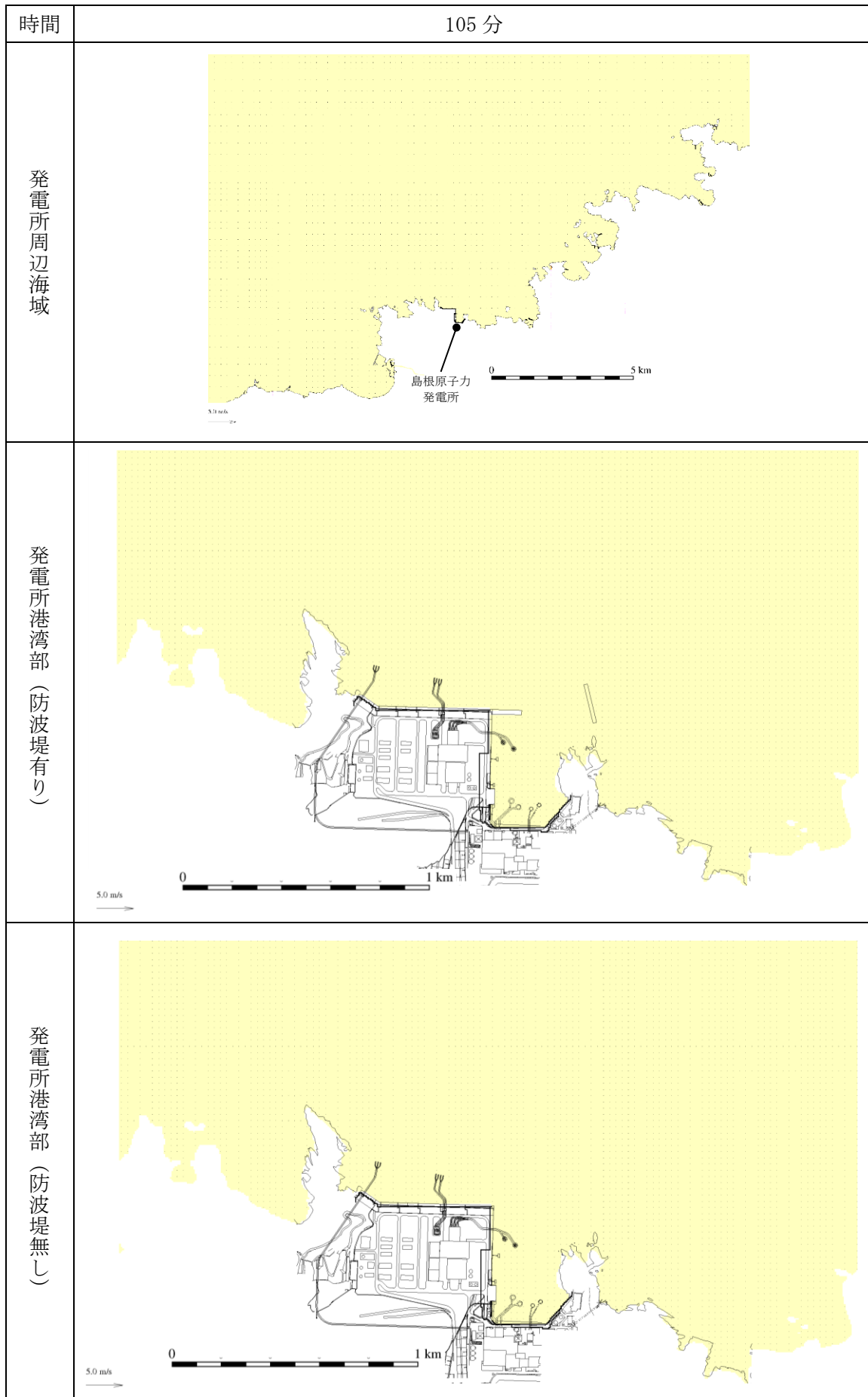
図 1-11 基準津波 1 の水位変動・流向ベクトル
