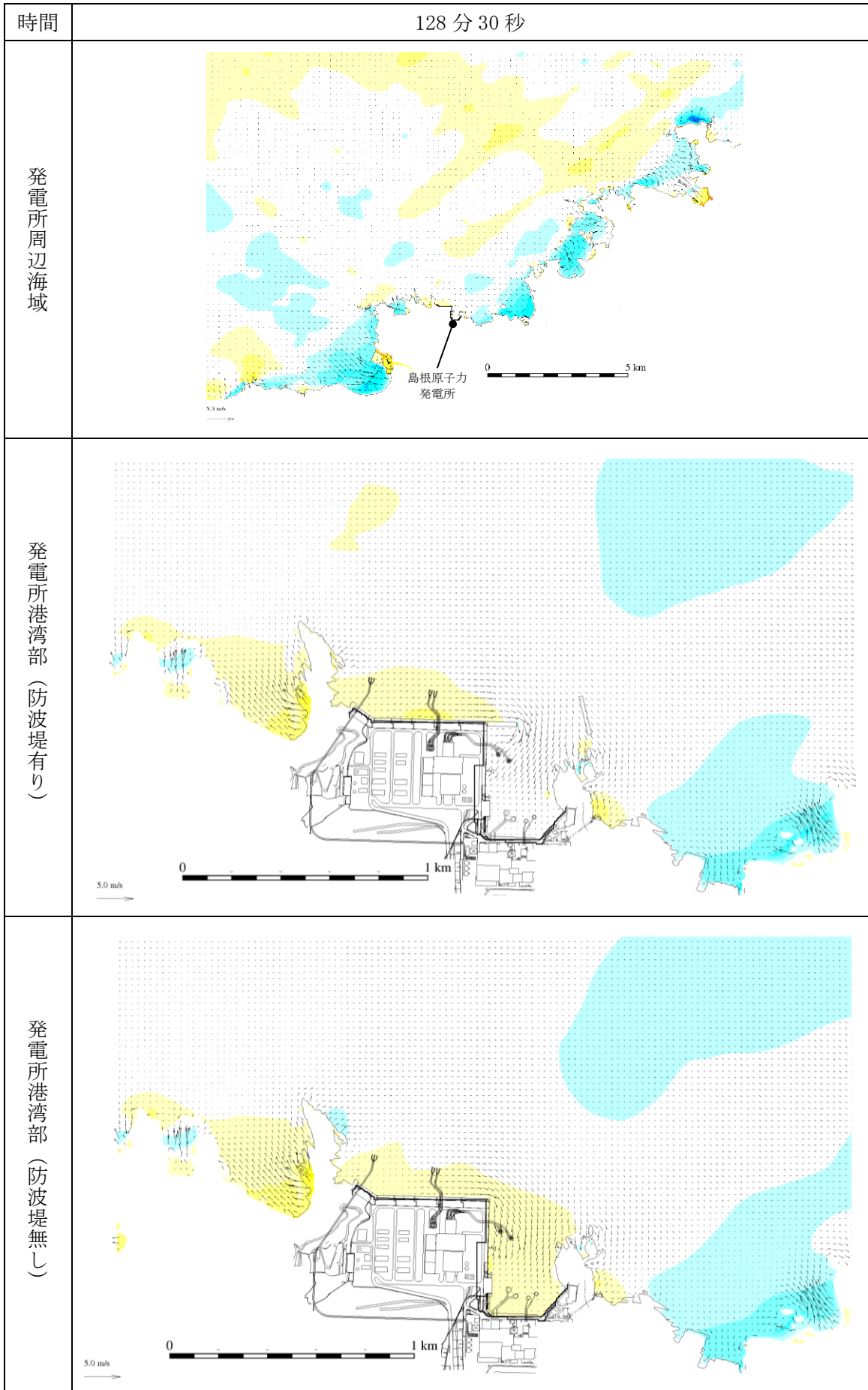
図 1-58 基準津波 1 の水位変動・流向ベクトル
