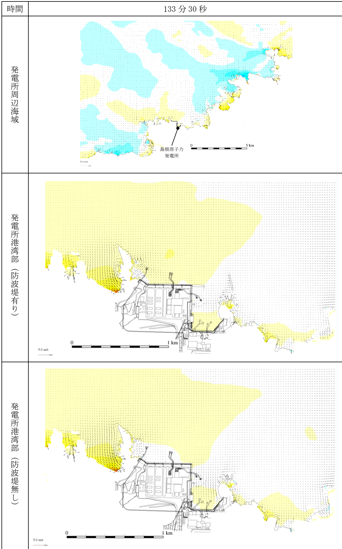
図 1-68 基準津波 1 の水位変動・流向ベクトル
