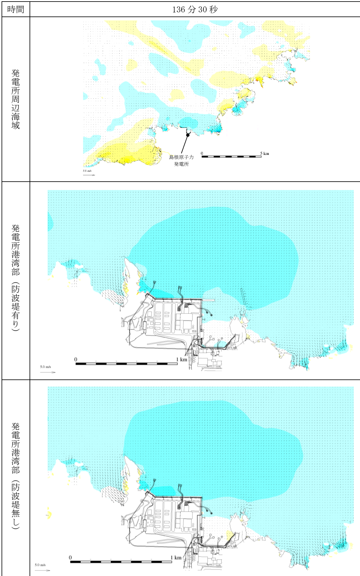
図 1-74 基準津波 1 の水位変動・流向ベクトル
