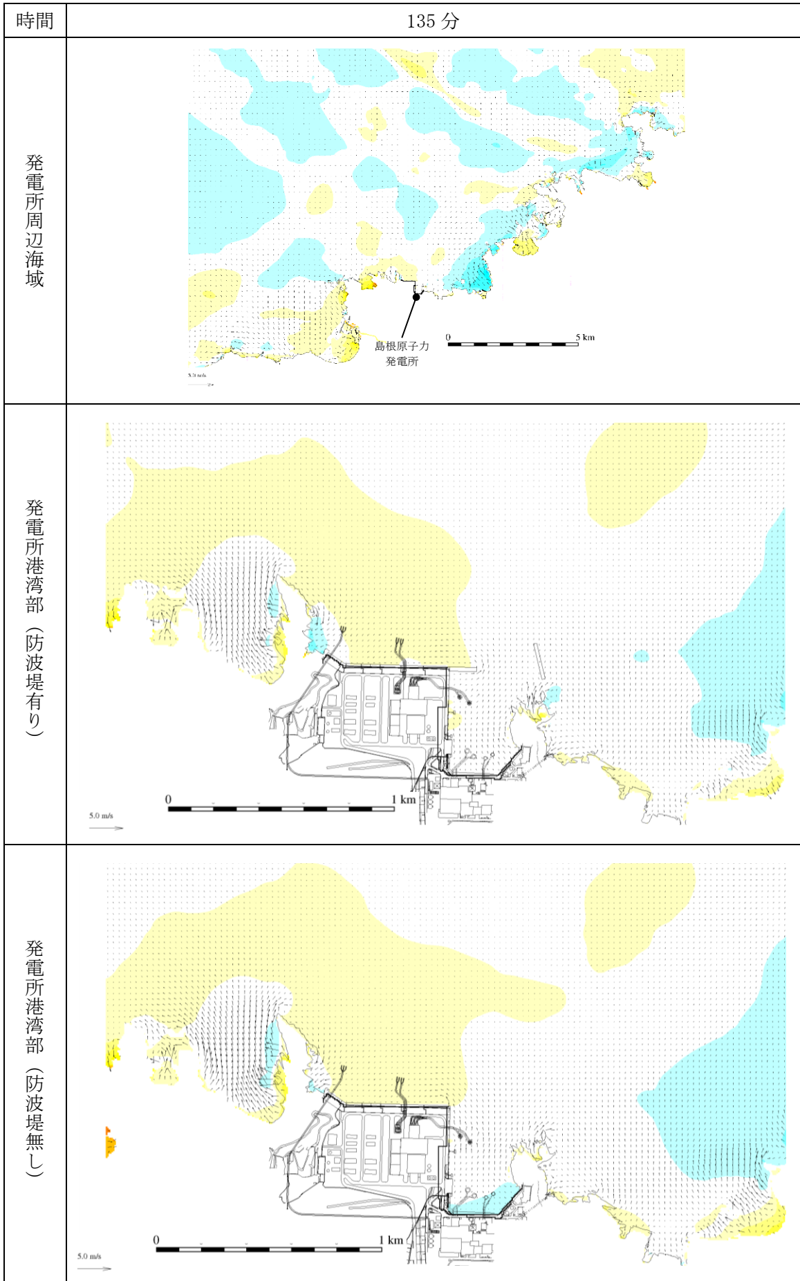
図 1-71 基準津波 1 の水位変動・流向ベクトル
