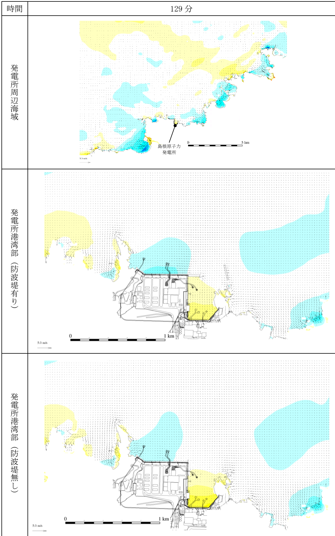
図 1-59 基準津波 1 の水位変動・流向ベクトル
