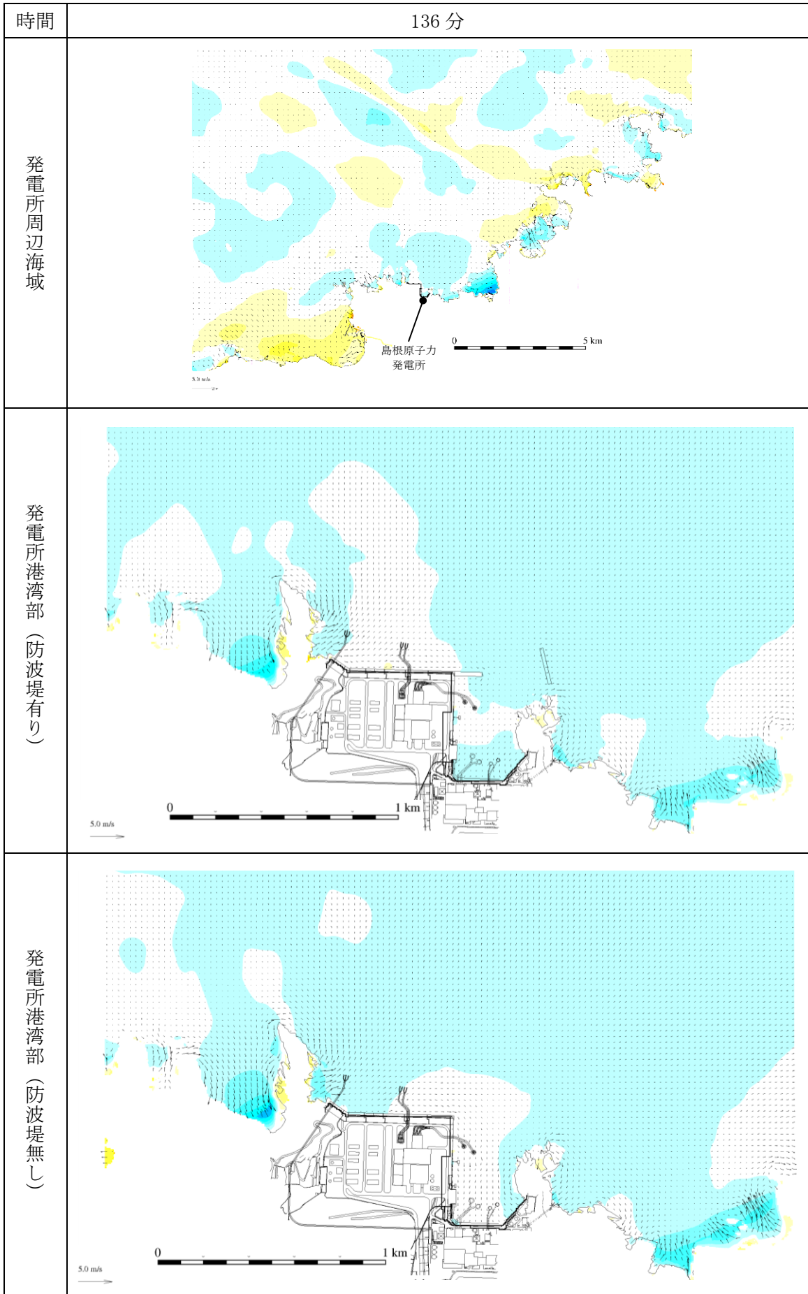
図 1-73 基準津波 1 の水位変動・流向ベクトル
