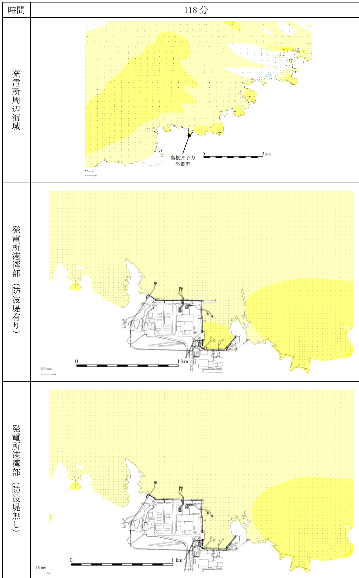
図 1-37 基準津波 1 の水位変動・流向ベクトル
