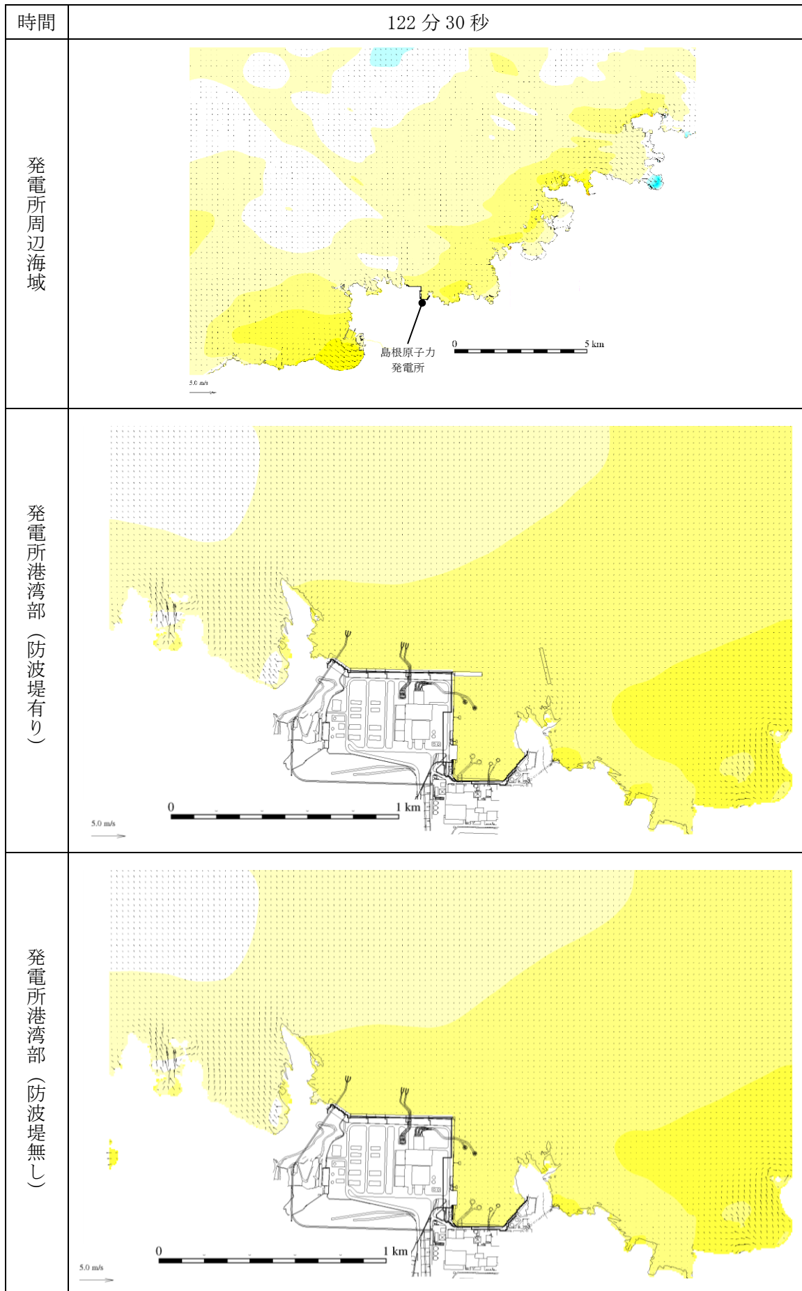
図 1-46 基準津波 1 の水位変動・流向ベクトル
