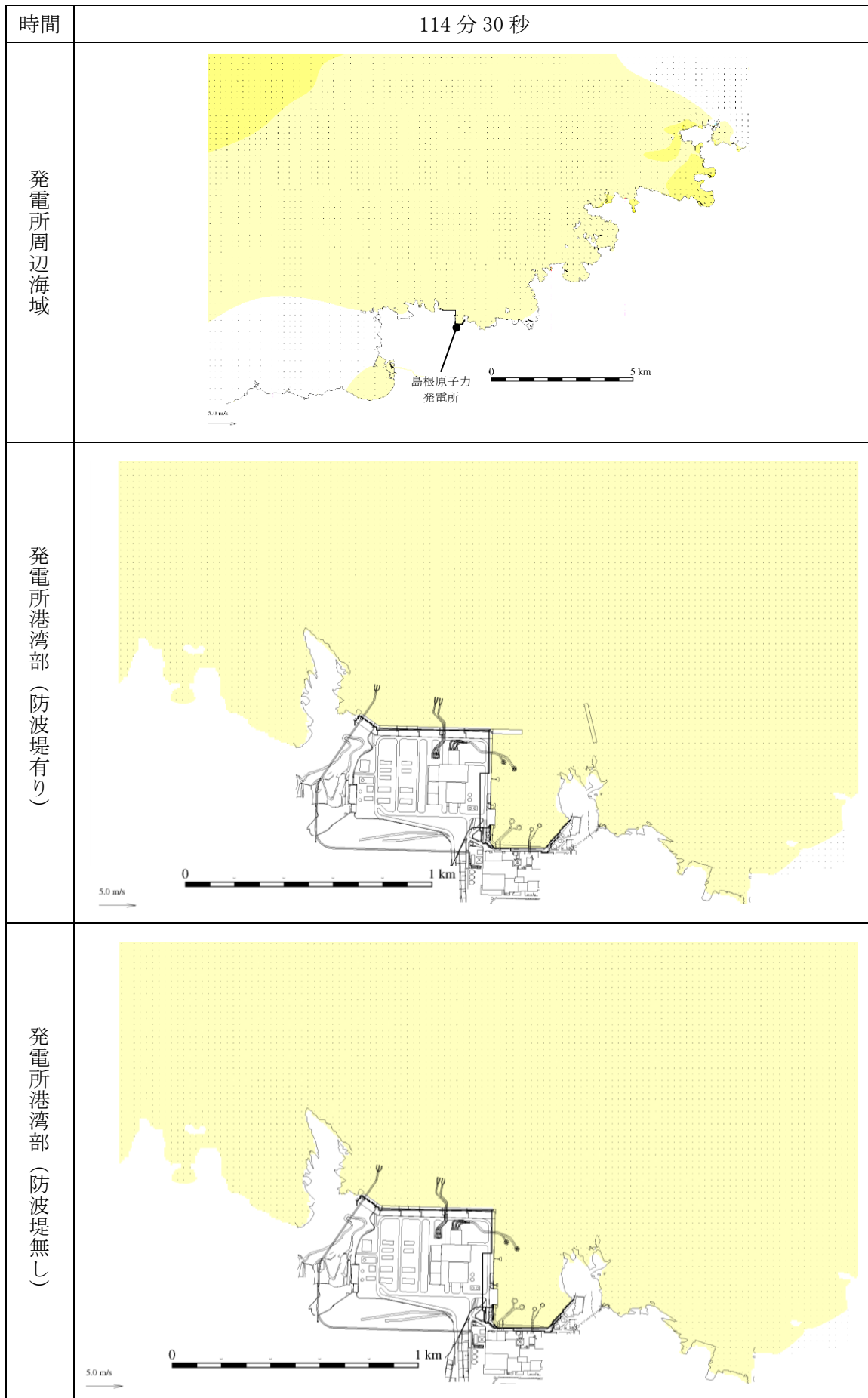
図 1-30 基準津波 1 の水位変動・流向ベクトル
