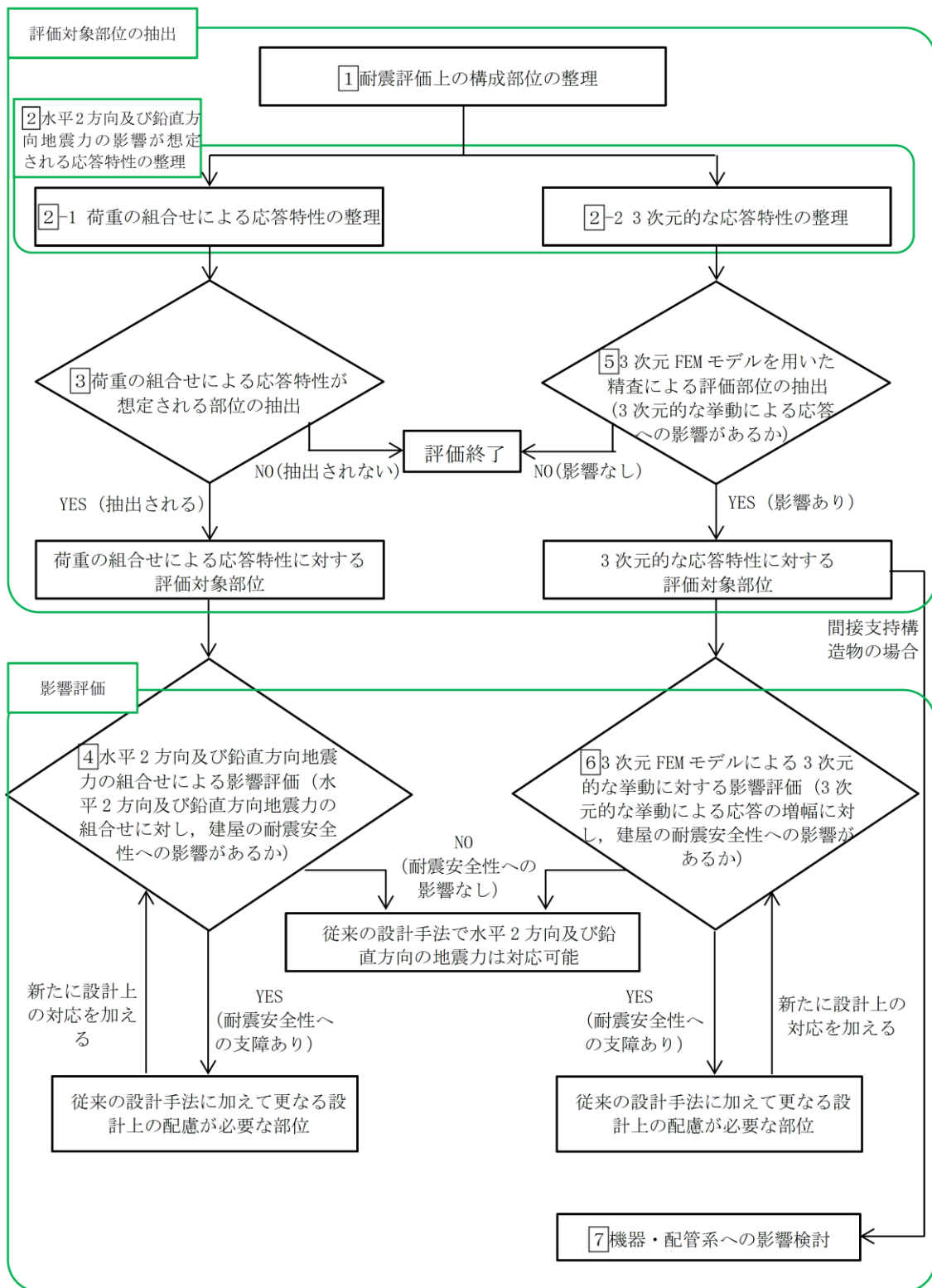
第 3.3-1 図 水平 2 方向及び鉛直方向地震力の組合せによる影響検討フロー
