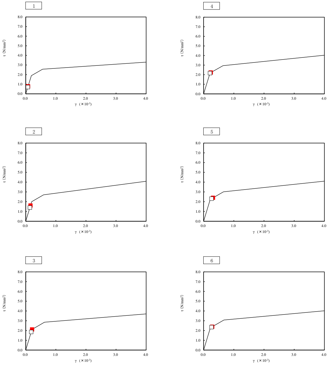
第 4.3-10 図 せん断スケルトンカーブ上の最大応答値 (2/2)
