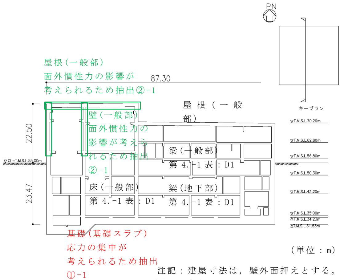
第 1. -2 図 燃料加工建屋の概略断面図 (1/2)
