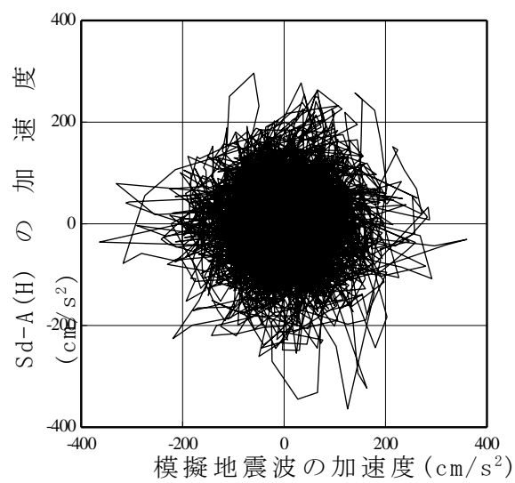
第 3.4-5 図 Sd-A のオービット
