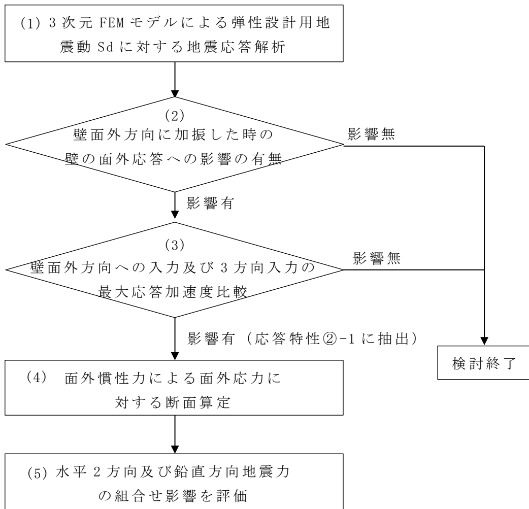
第 2.2-1 図 検討フロー
