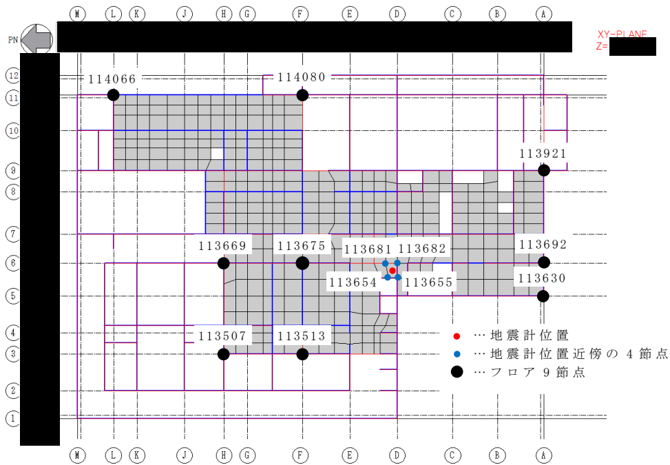
第 3.3.3-1 図 地上 4 階のモデル図
