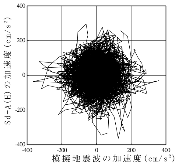
第 4.2-4 図 Sd-A のオービット
