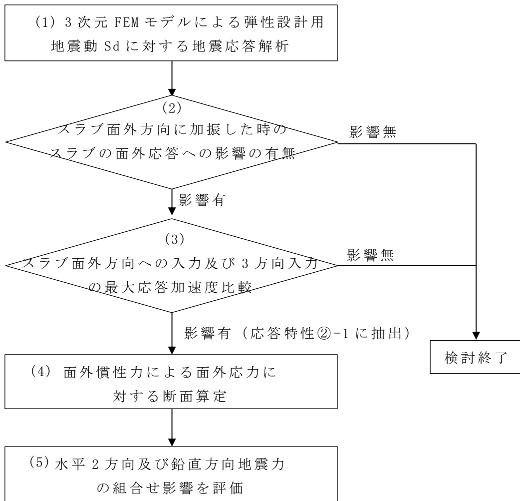
第 3.2-1 図 検討フロー
