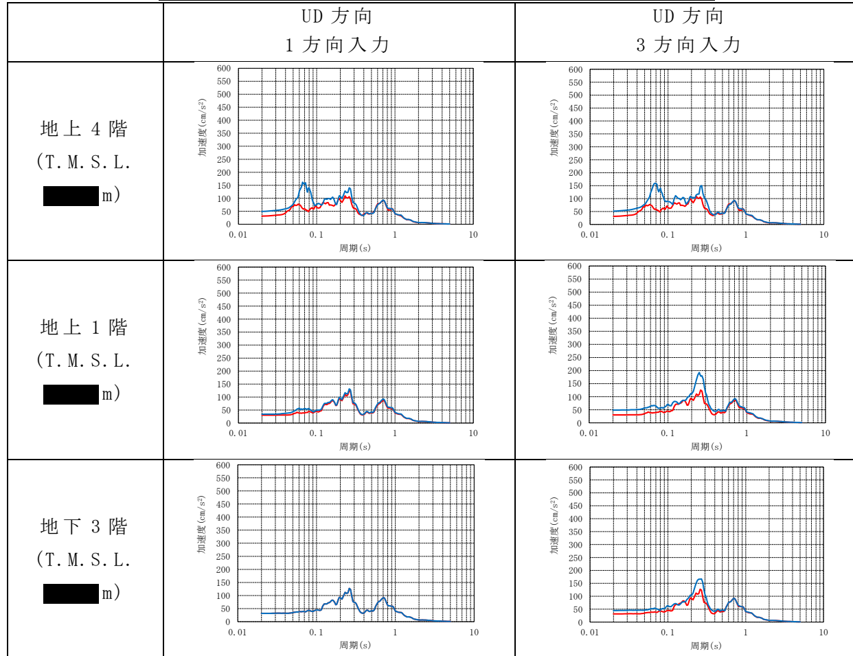
第 3.3.2-2 表 UD 方向の加速度応答スペクトルの比較
