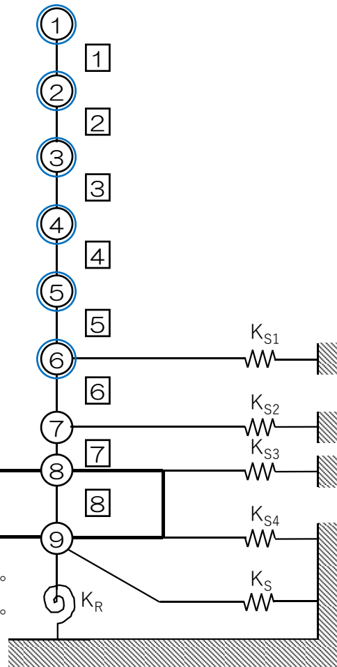
第 4.3-7 図 質点系モデルでの評価節点
