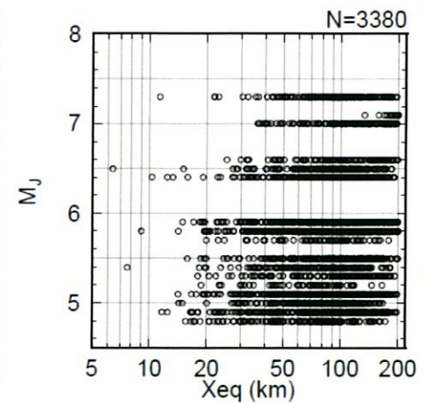
Xeq-Mjの分布
