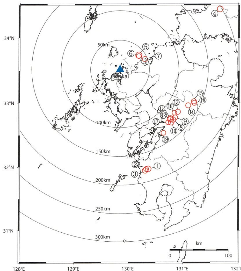
伝達関数による地盤減衰の同定に用いた地震の震央位置 (計19地震)
