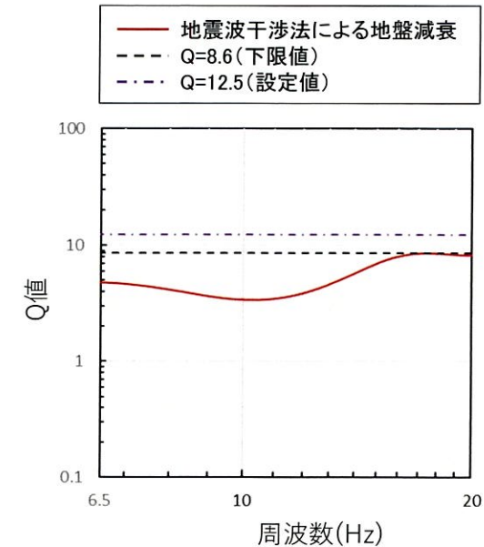
地震波干渉法により推定された地盤減衰(EL.11.0m~EL.-90.0m)
