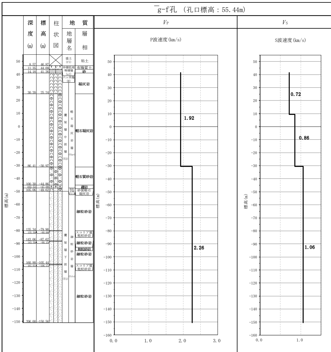
参考 2-1 図 燃料加工建屋の速度構造データ (3/8)
