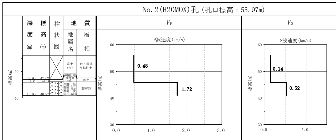
参考 2-1 図 燃料加工建屋の速度構造データ (7/8)
