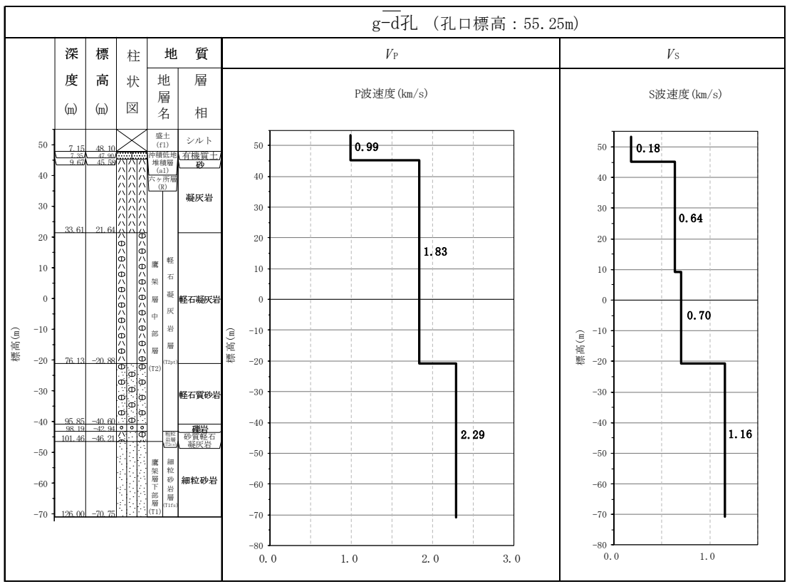
参考 2-1 図 燃料加工建屋の速度構造データ (4/8)
