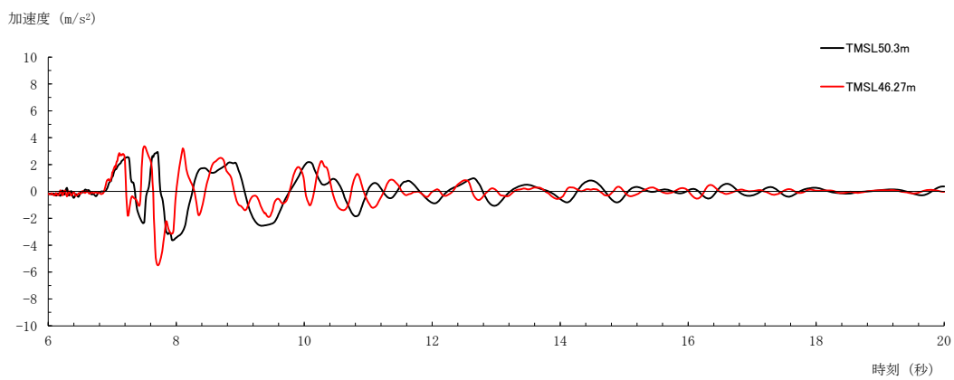
第 5.5-13 図 加速度時刻歴波形 ( S_S -C1, -\sigma , 水平方向, 逐次非線形解析)
