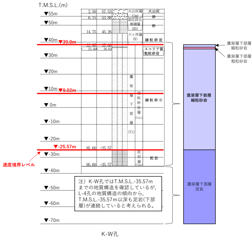
第 2.2-1 図 地質柱状図
