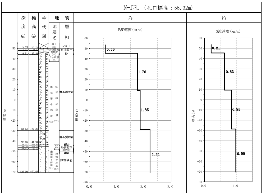
参考 2-1 図 燃料加工建屋の速度構造データ (2/8)
