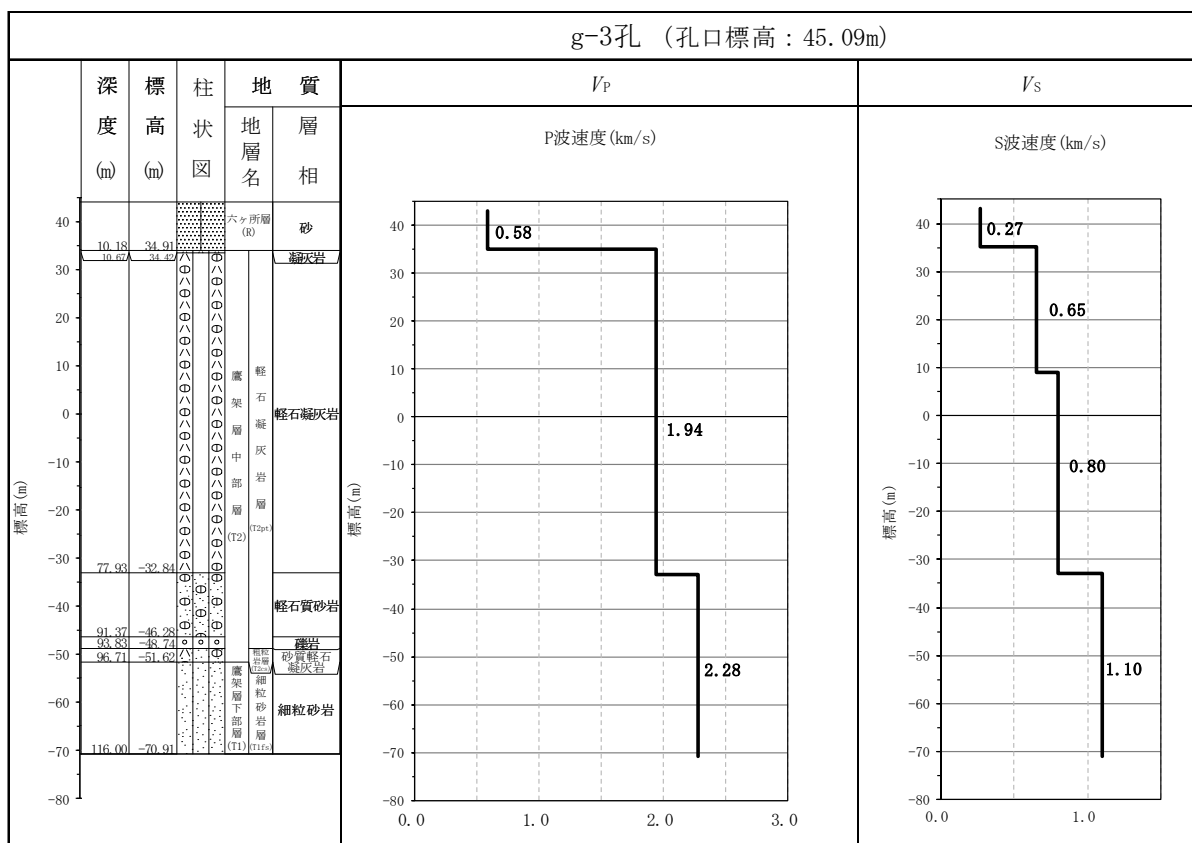
参考 2-1 図 燃料加工建屋の速度構造データ (1/8)
