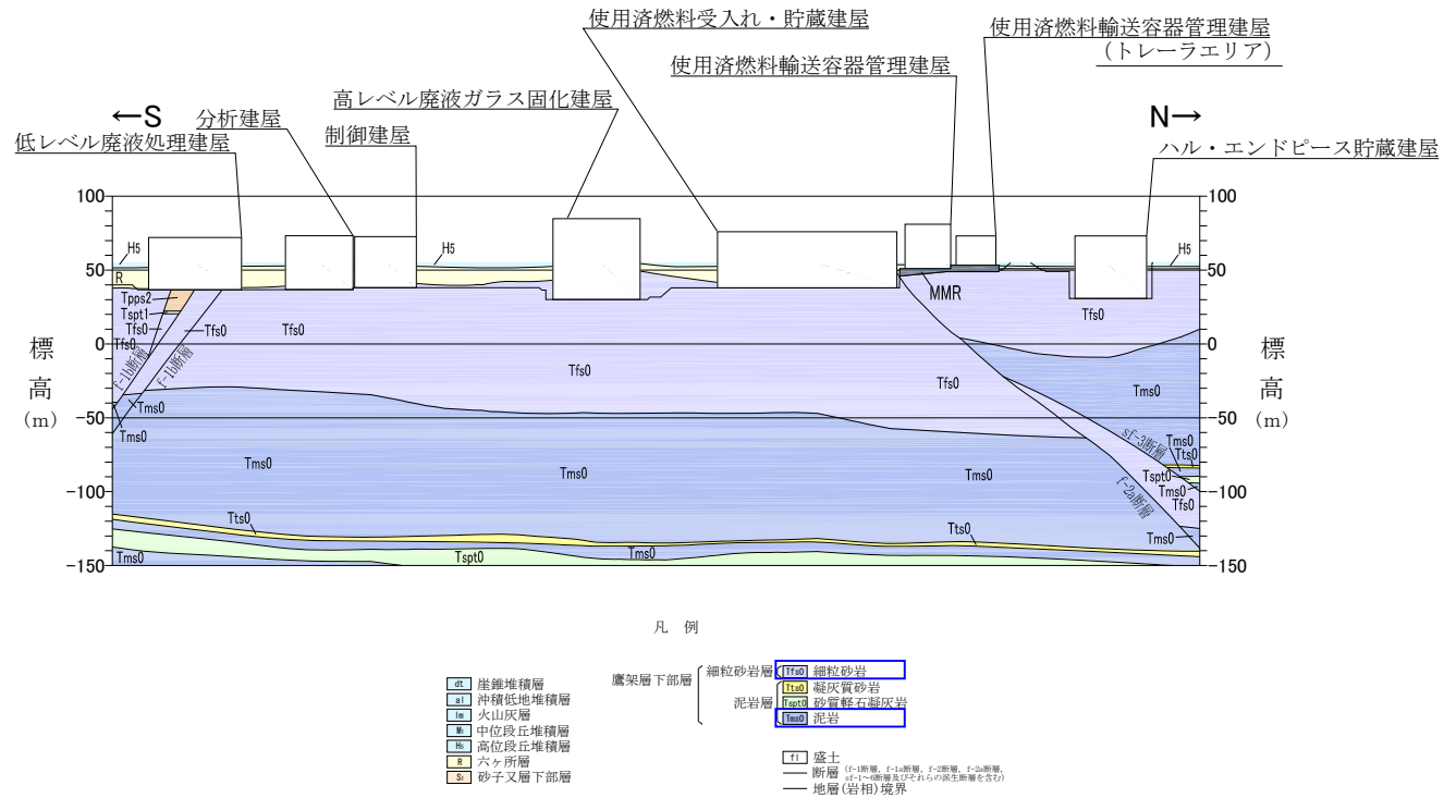
第 2.3-1 図 (2) 中央地盤エリアの地質断面図
