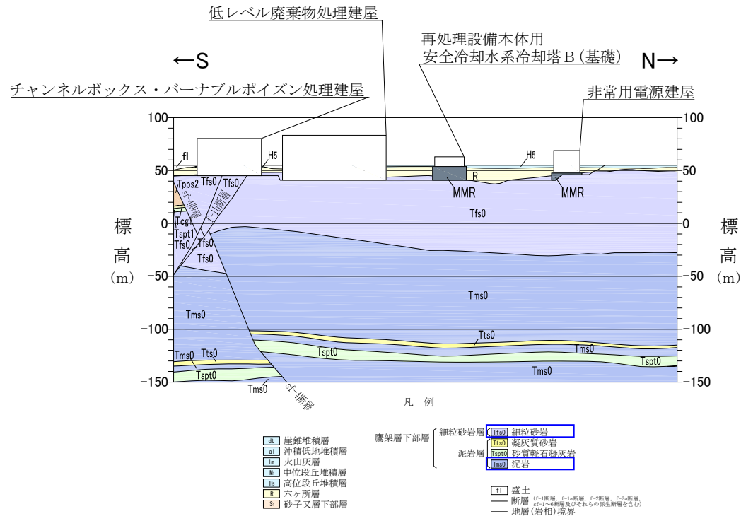
第 2.3-1 図 (1) 中央地盤エリアの地質断面図
