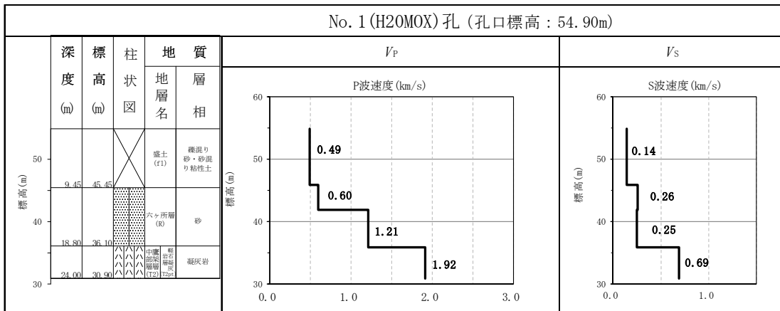
参考 2-1 図 燃料加工建屋の速度構造データ (6/8)
