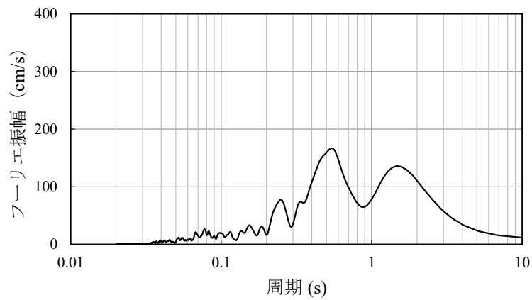
第 5.5-12 図 フーリエ振幅スペクトル ( S_S -C1) (Perzen ウィンドウ 0.5Hz)
