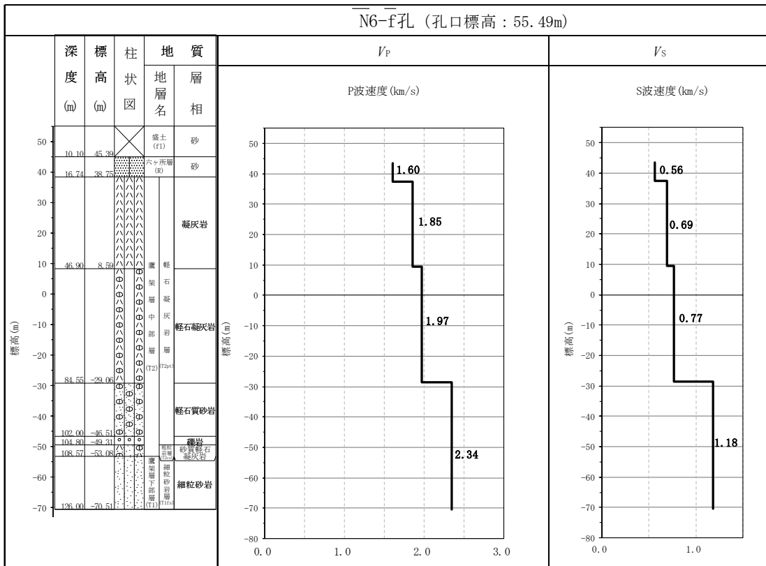
参考 2-1 図 燃料加工建屋の速度構造データ (5/8)
