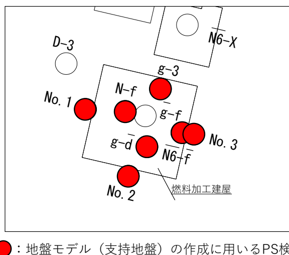
第 3.1-1 図 燃料加工建屋の地盤モデル作成に用いる PS 検層孔位置図 (表層地盤)
