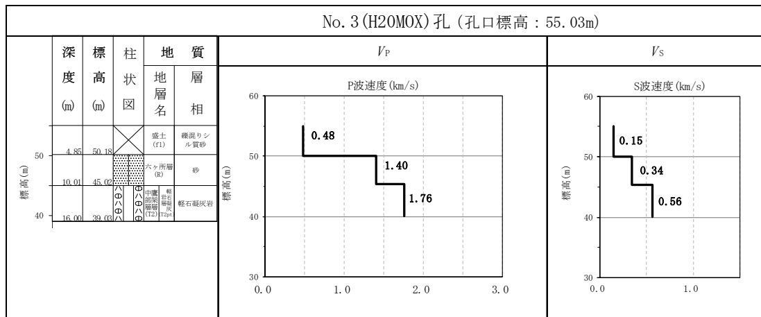
参考 2-1 図 燃料加工建屋の速度構造データ (8/8)
