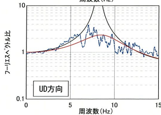
伝達関数 (EL. -17m/EL. -90m) の比較
