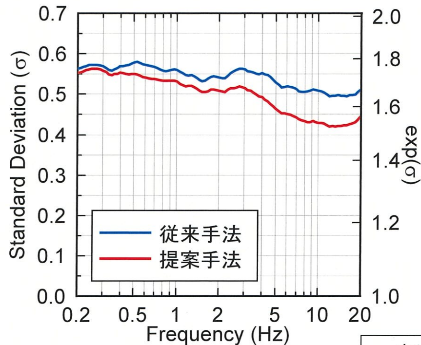
残差の標準偏差の比較
