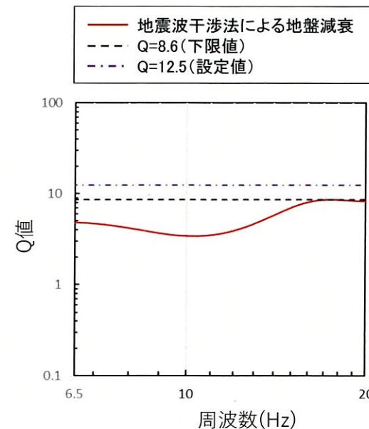
地震波干渉法により推定された地盤減衰(EL.11.0m~EL.-90.0m)
