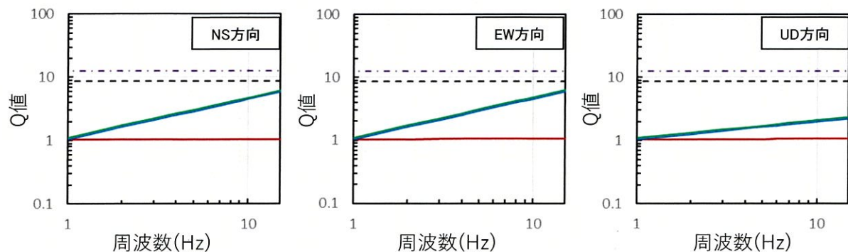
伝達関数により同定された地盤減衰(EL.11.0m~EL.-90.0m)
