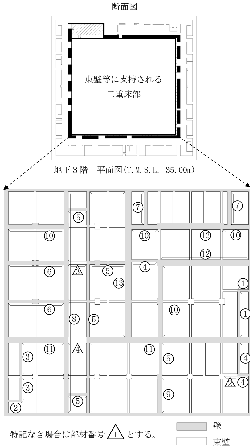
第 3.2-2 図 束壁部及び壁の部材リスト (T.M.S.L. 34.23m~34.40m)
