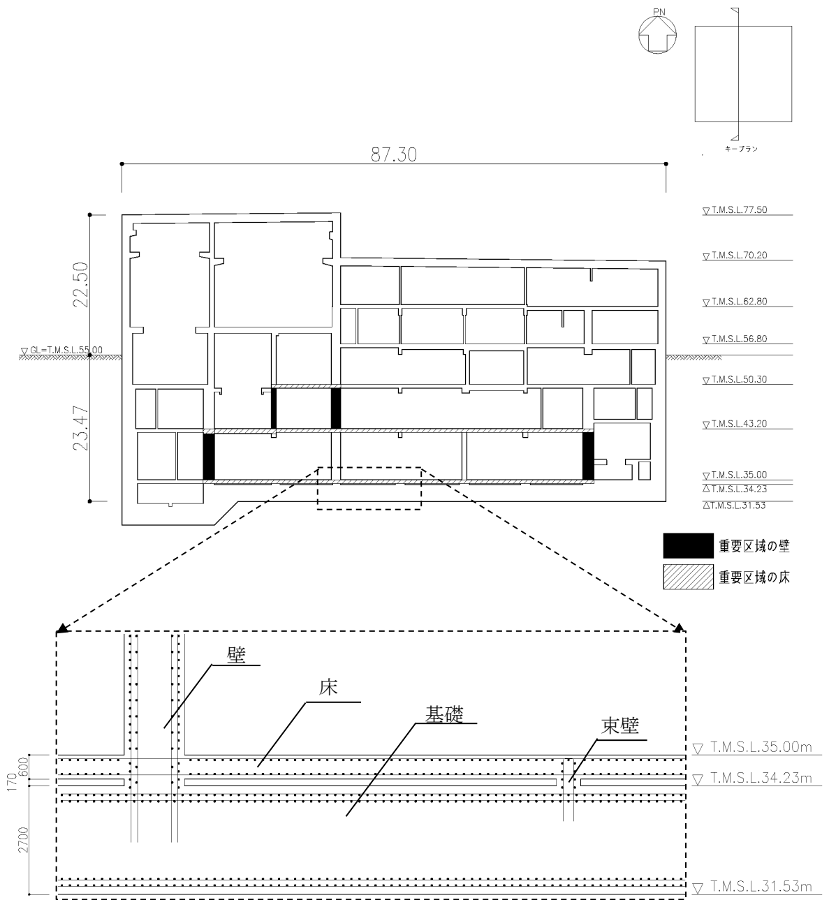
第 3.2-1 図 二重床部の詳細断面図
