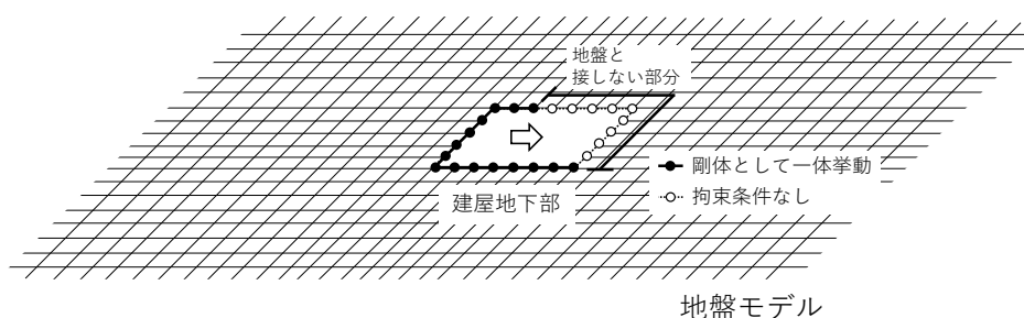
第5.1-1図 周辺地盤との接触状況の実状を考慮した評価の概念図
