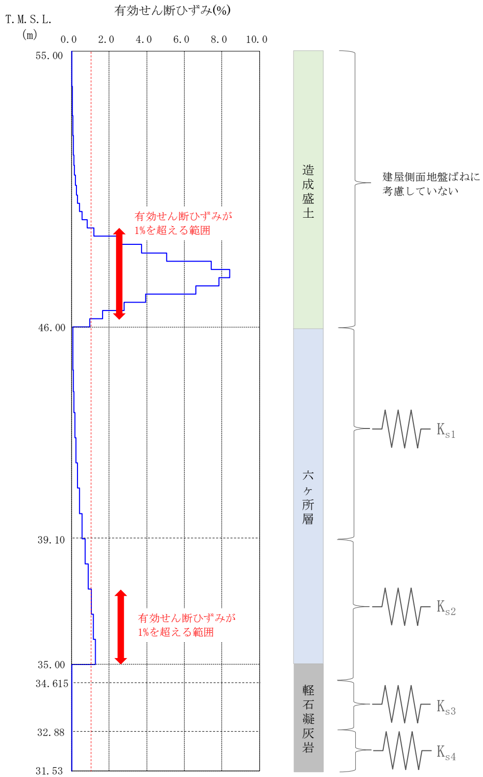
第 2.-1 図 地盤の有効せん断ひずみ (基準地震動 Ss-C1, 地盤物性- \sigma )
