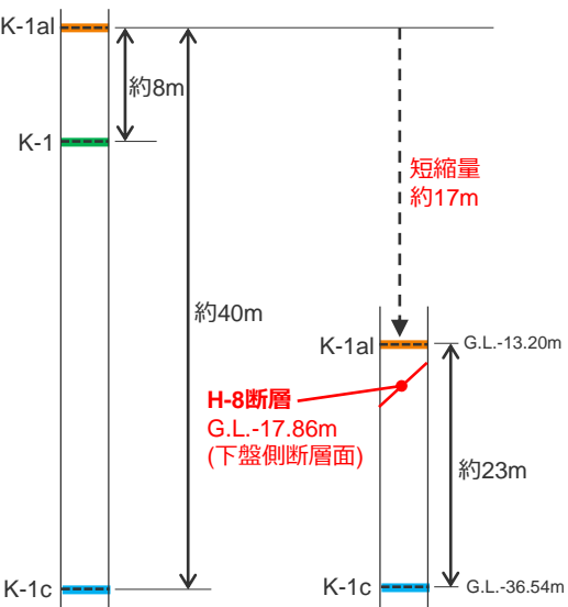
D-2孔の簡易柱状図
