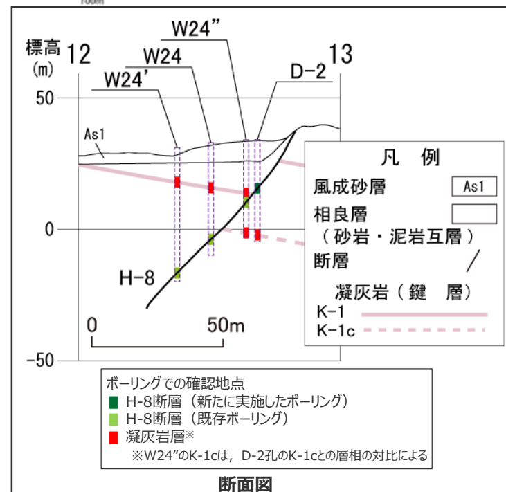
断面図
