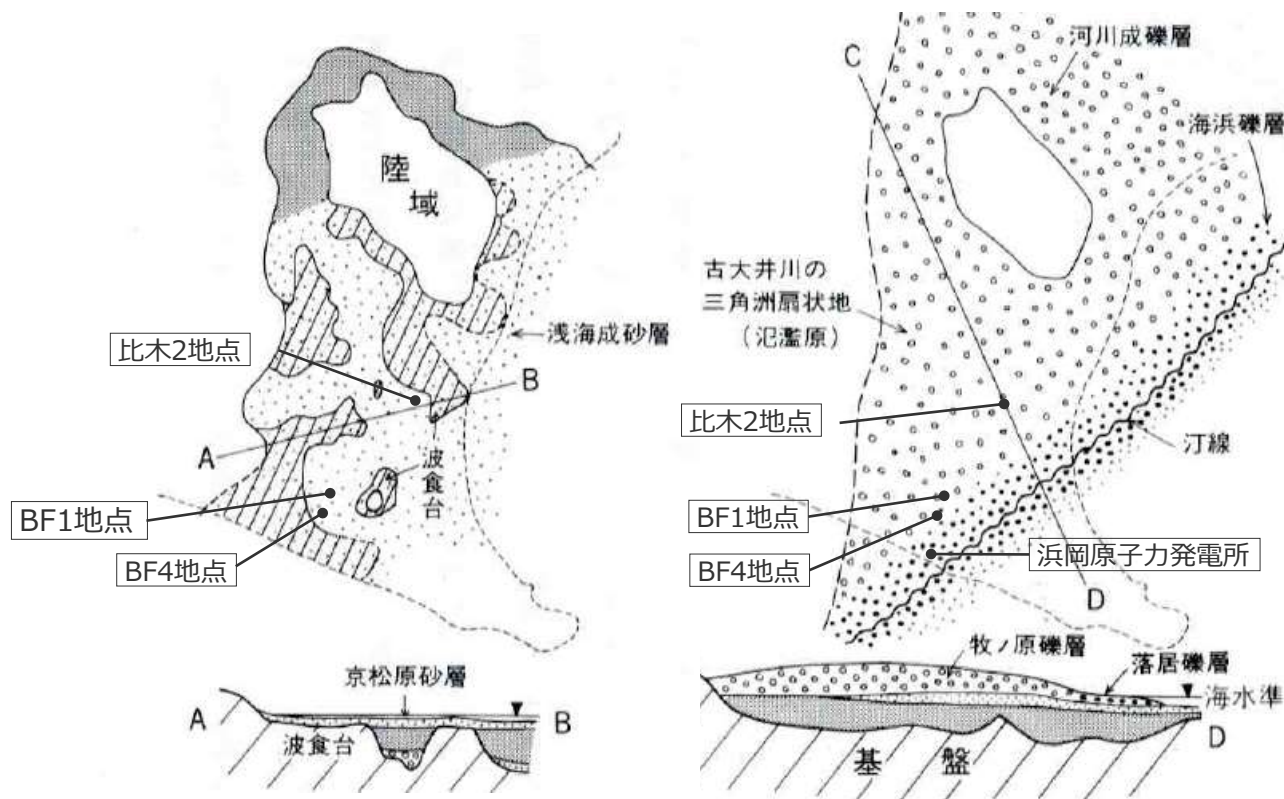
杉山ほか（1988）の「4京松原砂層の堆積時」,「5牧ノ原礫層の堆積時（後期）」に加筆
