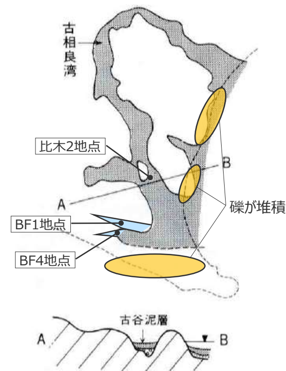
杉山ほか（1988）の「2 古谷泥層中部の堆積時」に加筆
