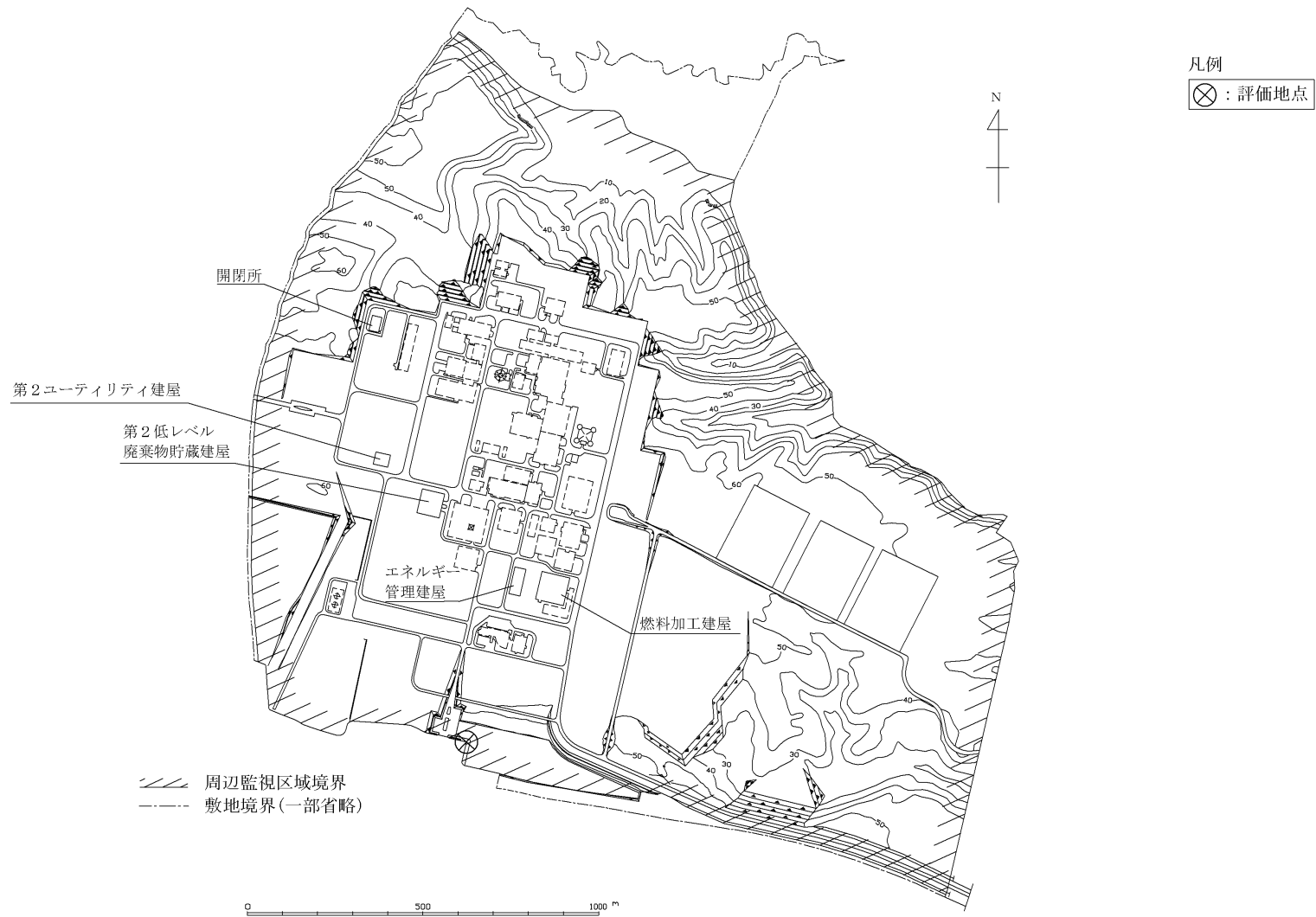
第 3.-1 図 加工施設からの直接線及びスカイシャイン線による一般公衆の線量率評価地点
