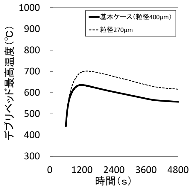
第4図 ULOF(iii)デブリベット最高温度の履歴
