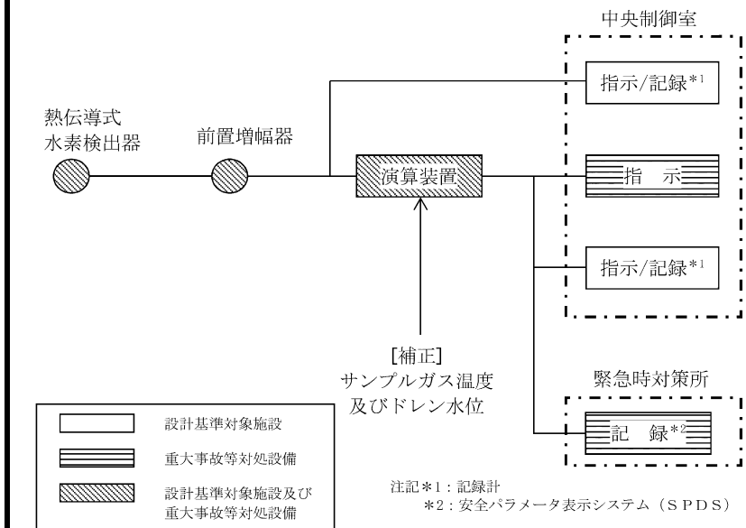
図 3-61 格納容器水素濃度 (B系) の概略構成図
