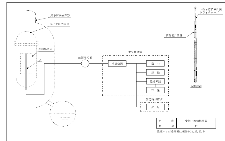
図 3-2 検出器の構造図 (中性子源領域計装)
