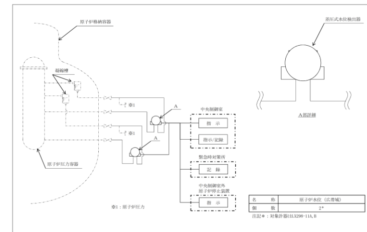
図 3-38 検出器の構造図 (原子炉水位 (広帯域))
