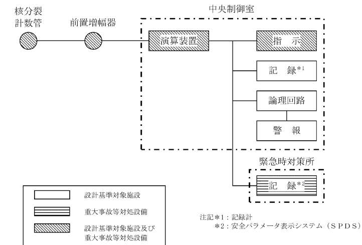
図 3-1 中性子源領域計装の概略構成図
