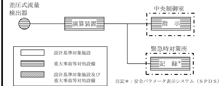
図 3-31 残留熱代替除去系原子炉注水流量の概略構成図
