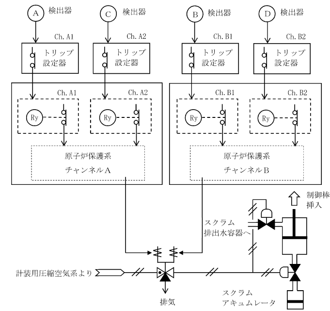
図3-119 原子炉保護系の構成例
