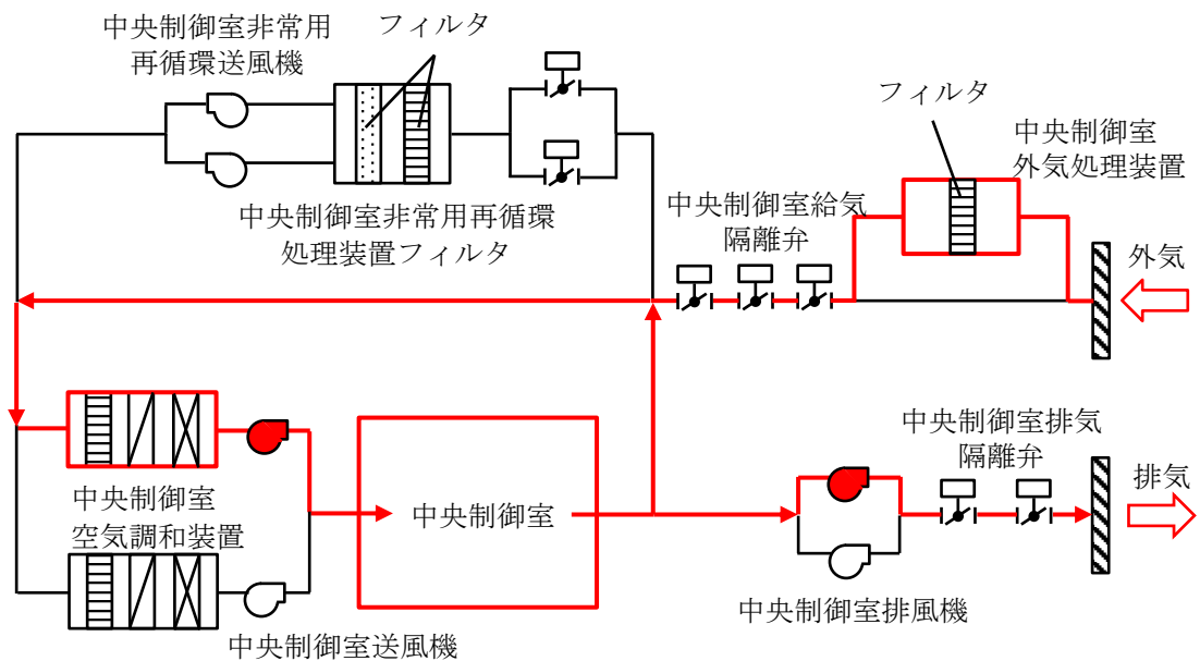
図1-5 中央制御室換気空調系の概要図（通常運転時）
