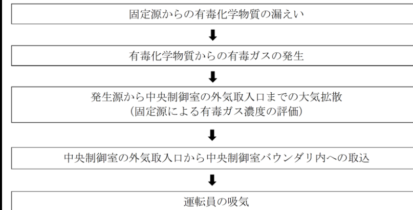
図 4-1 中央制御室の有毒ガスの到達経路
