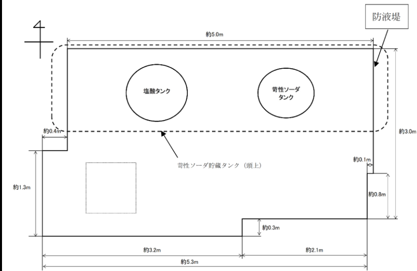
図 2-4 受動的に機能を発揮する設備 (敷地内固定源)
