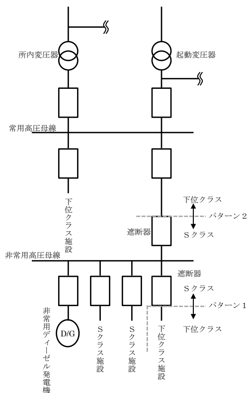
図 5-2-1 受電系統概念図
