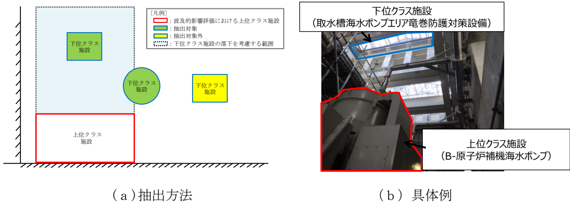
図 4-1 下位クラス施設の落下に伴う上位クラス施設への衝突を想定した抽出方法及び具体例
