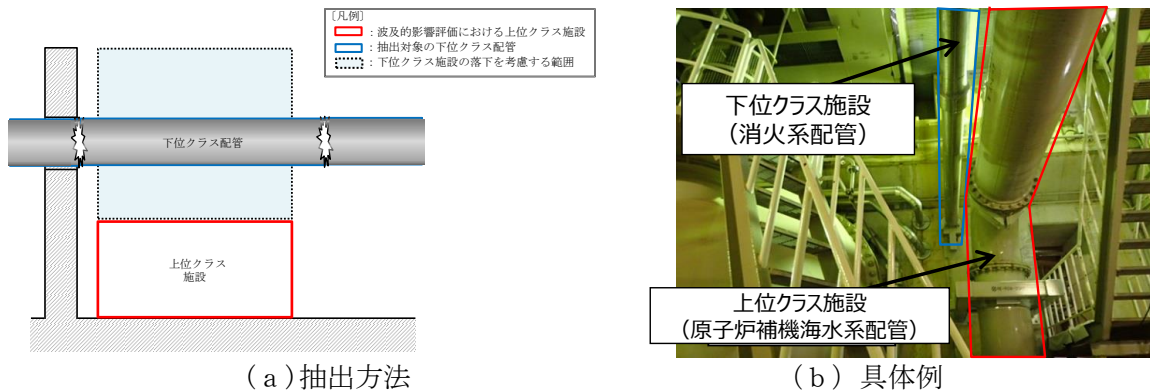
図 4-2 下位クラスの配管の落下に伴う上位クラス施設への衝突を想定した抽出方法及び具体例
