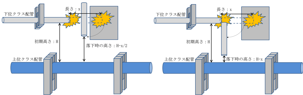
(a) 2 箇所の同時破損を想定
