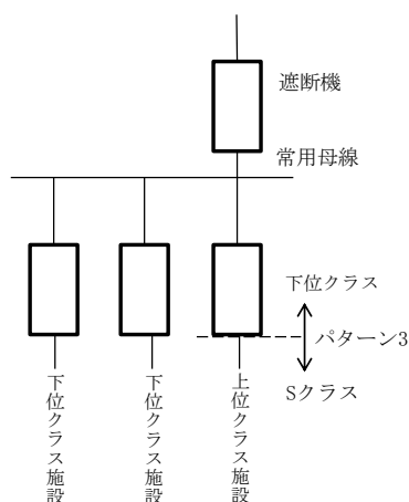
図5-2-2 受電系統概念図（パターン1，2以外）
