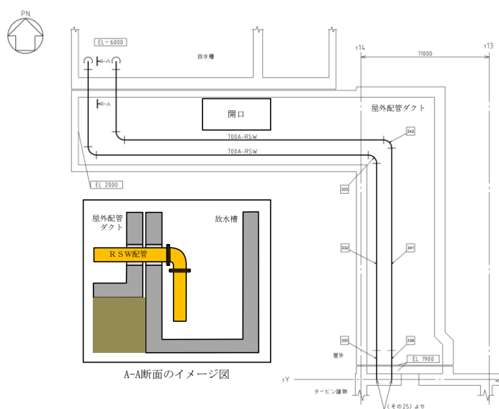
図 1 R S W配管放水ラインの概略構造図
