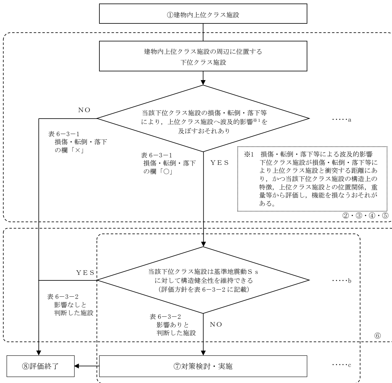
図 5-3 損傷，転倒，落下等により建物内上位クラス施設へ影響を及ぼすおそれのある下位クラス施設の抽出及び評価フロー
