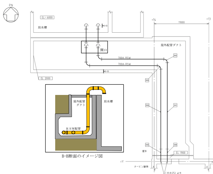
図 2 R S W配管放水ラインの信頼性向上の例
