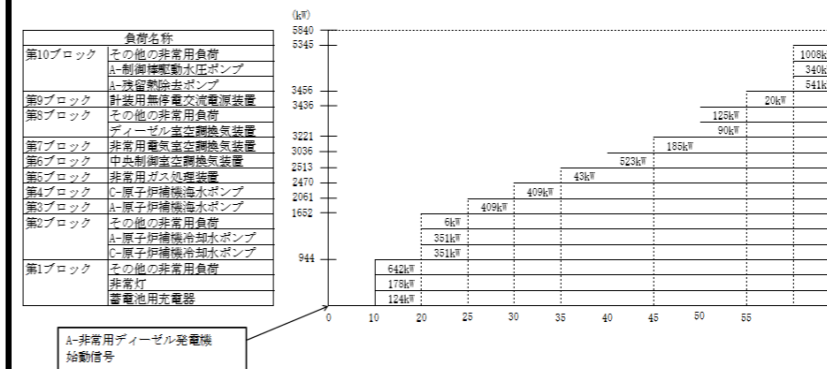
図 3-1 発電所を安全に停止するために必要な負荷 (A-非常用ディーゼル発電機) 積算イメージ
