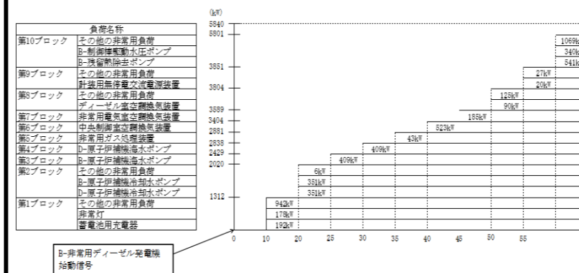
図 3-2 発電所を安全に停止するために必要な負荷 (B-非常用ディーゼル発電機) 積算イメージ
