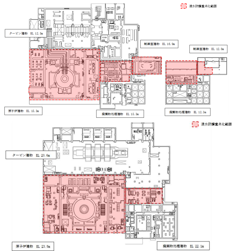
図 3-29 浸水防護重点化範囲 (平面図) (2/4)
