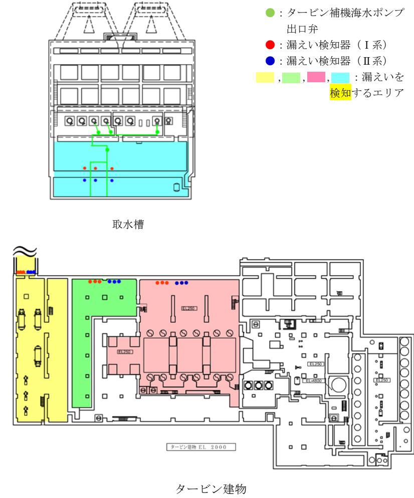
図 4-3 漏えい検知器及びタービン補機海水ポンプ出口弁配置図
