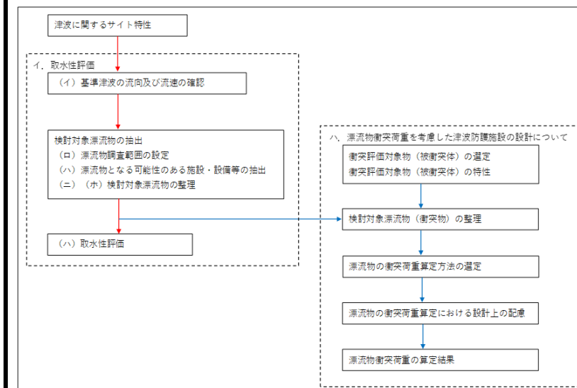
図 3-36 漂流物評価フロー(1/2)
