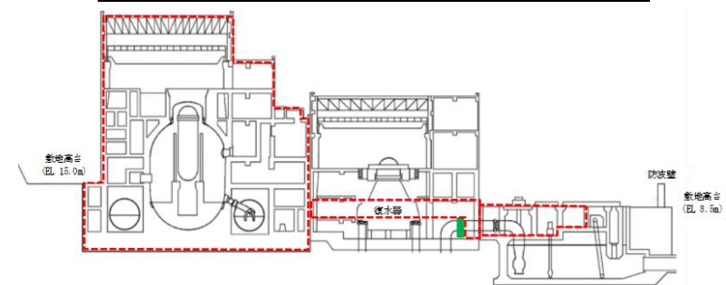
図 3-29 浸水防護重点化範囲 (断面図)
