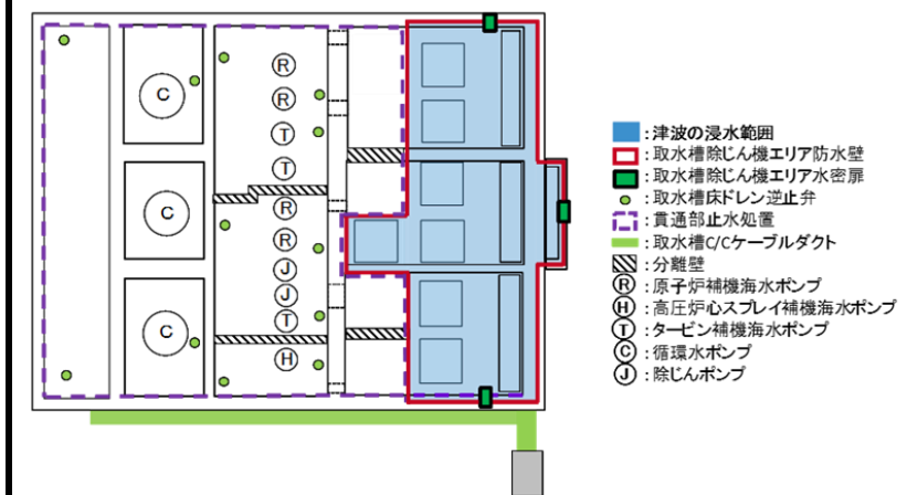
図 3-8 取水槽の浸水対策の概要 (平面図)
