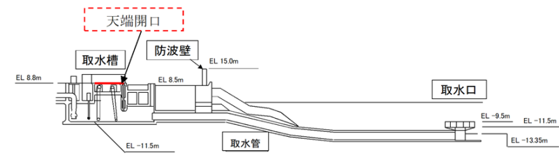
図 3-17 1号機 取水施設の断面図
