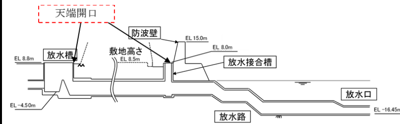
図 3-11 2号機 放水施設の断面図
