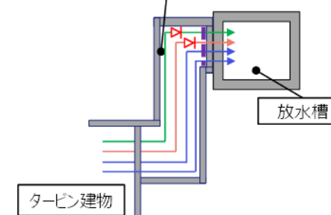
図 3-12 屋外配管ダクト平面図
