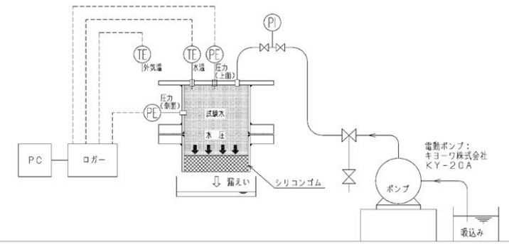
図 4-6 シール材の漏えい試験の概要
