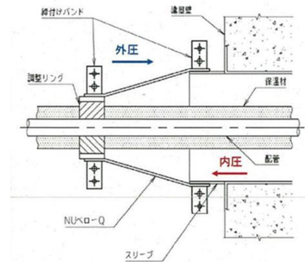
図 4-7 ブーツの漏えい試験の概要
