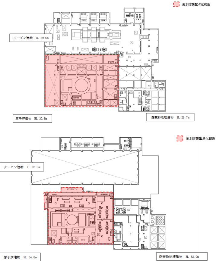
図 3-29 浸水防護重点化範囲 (平面図) (3/4)
