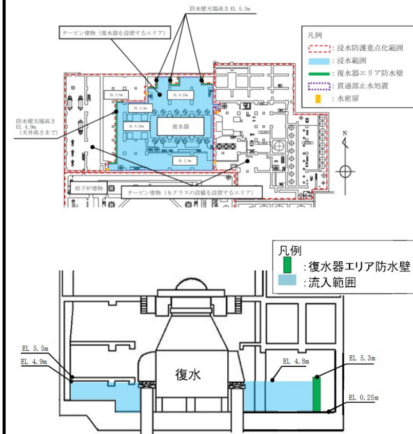
図 3-30 タービン建物 (復水器を設置するエリア) における浸水対策
