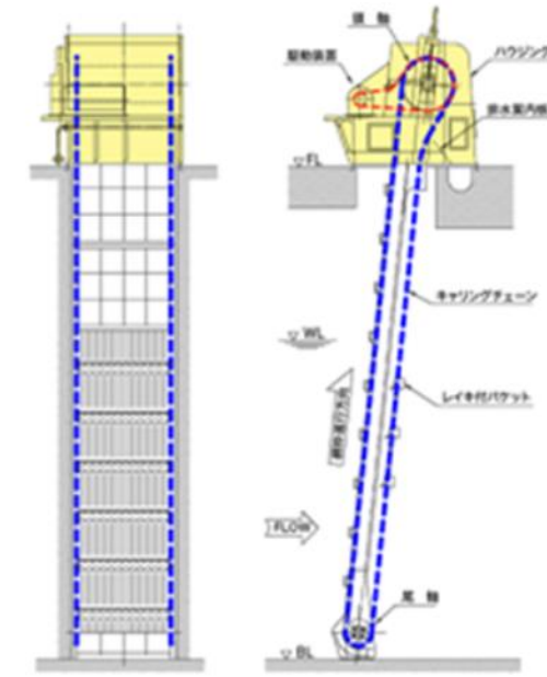
図3-39 除じん装置の概要
