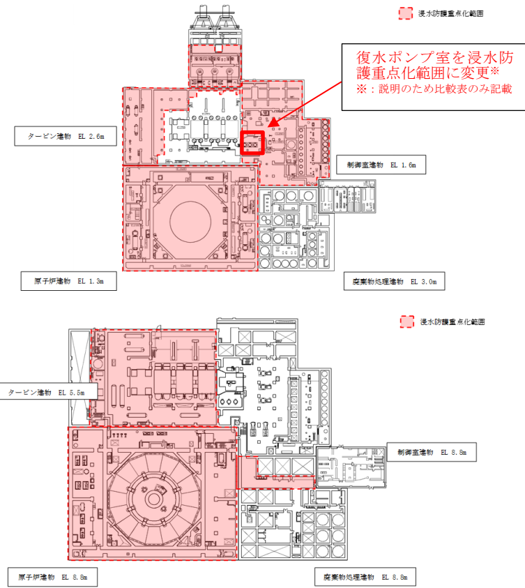
図 3-29 浸水防護重点化範囲 (平面図) (1/4)
