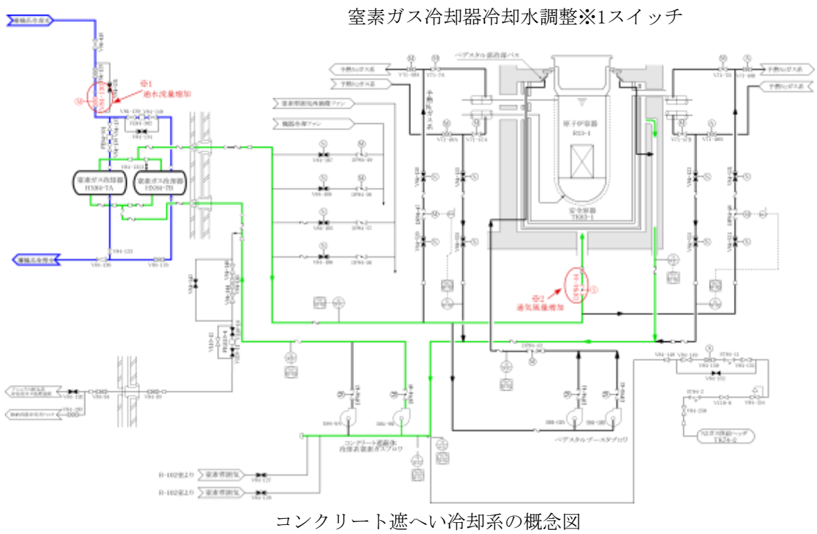
第 3. 6. 1. 3. 1 図 コンクリート遮へい体冷却系による安全容器外面冷却の補足 (1/2)
