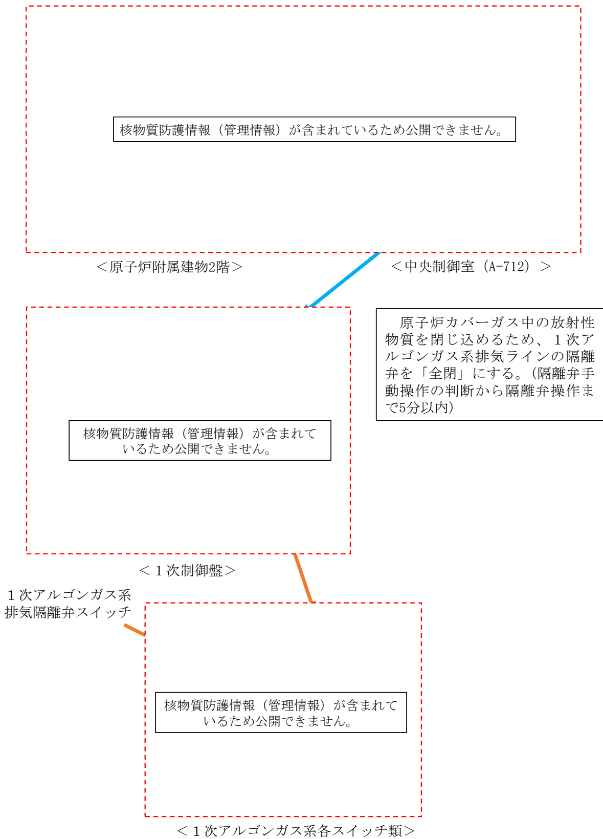
第3.2.6.1図 1次アルゴンガス系の排気側の隔離の補足
