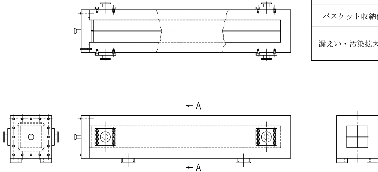
断面AA
