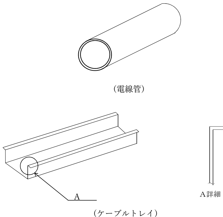
第1図 電線管及びケーブルトレイの構造
