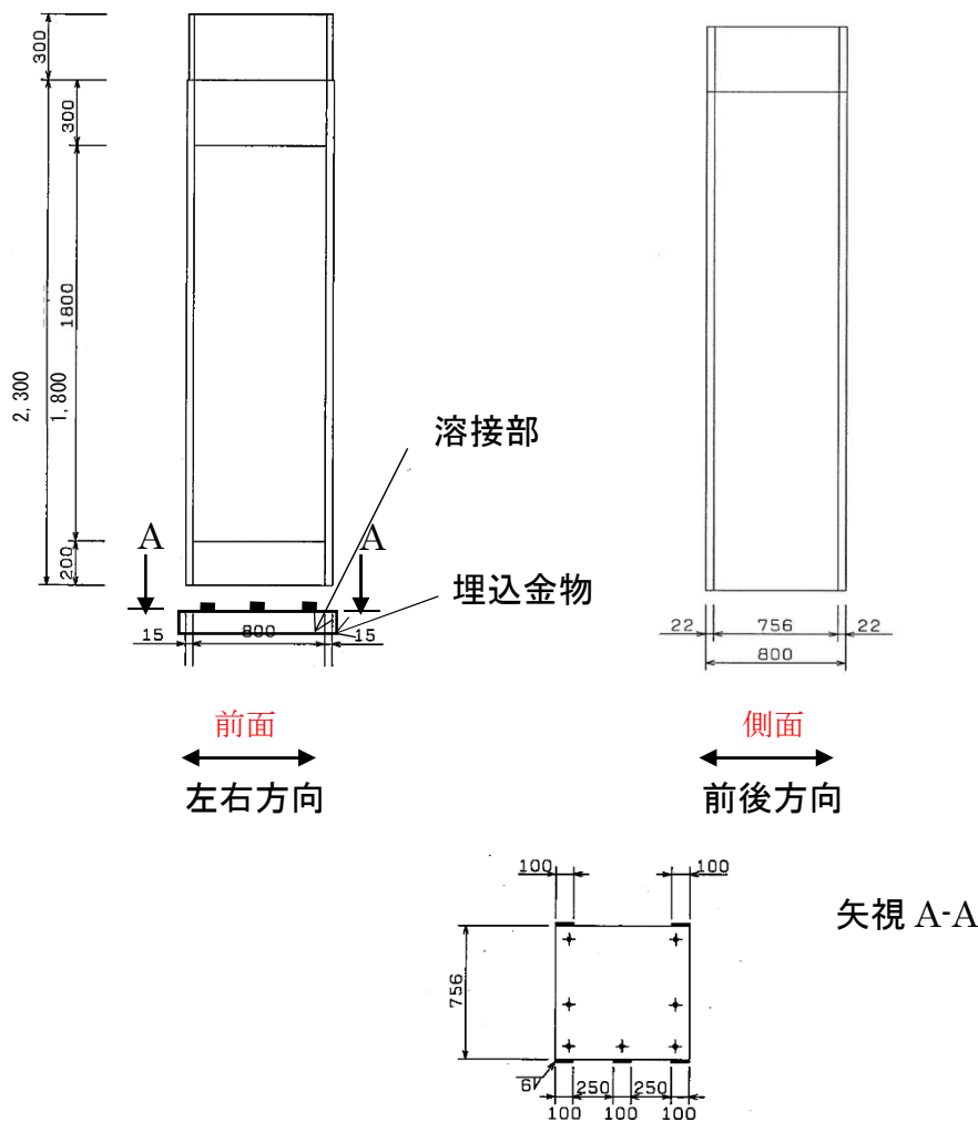
第1図 切替盤の外形図
