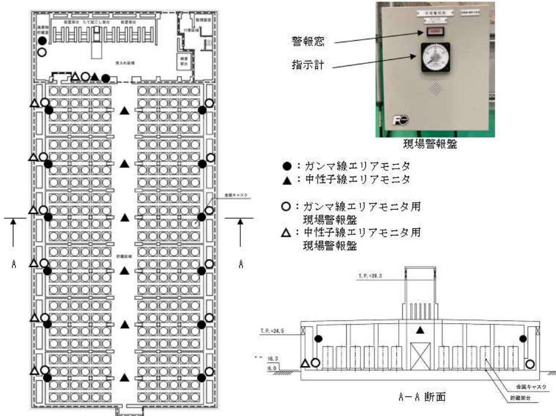
第8-4図 エリア放射線モニタの検出器と現場警報盤の配置図
