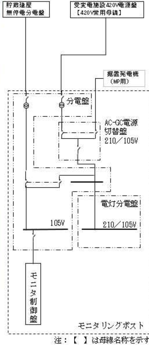
参考-1図 据置発電機, 分電盤, AC-DC切替盤と電源系統図
