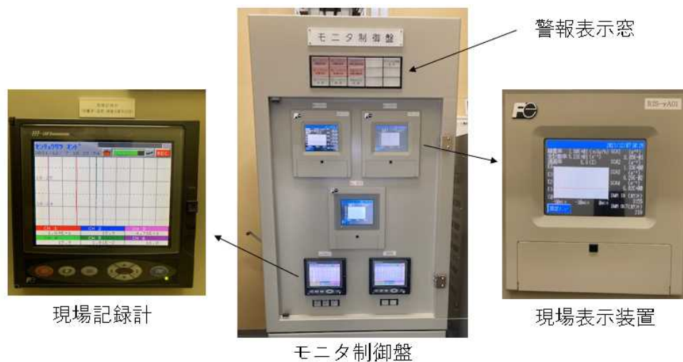
第8－2図 モニタ制御盤の警報表示部及び表示ディスプレイ部
