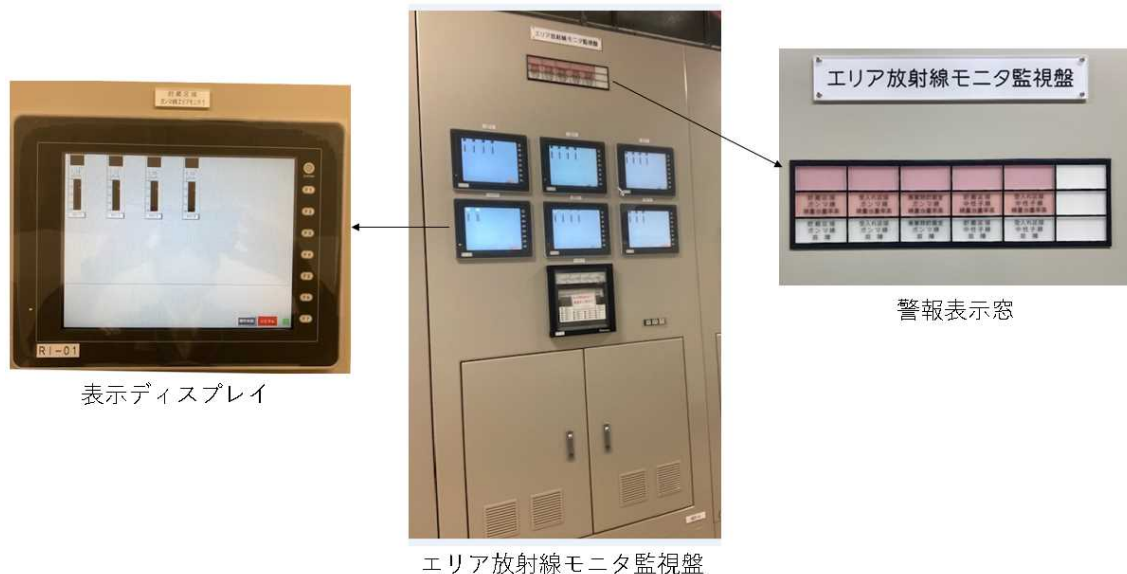
第8-3図 エリア放射線モニタ監視盤の警報表示部とディスプレイ表示部
